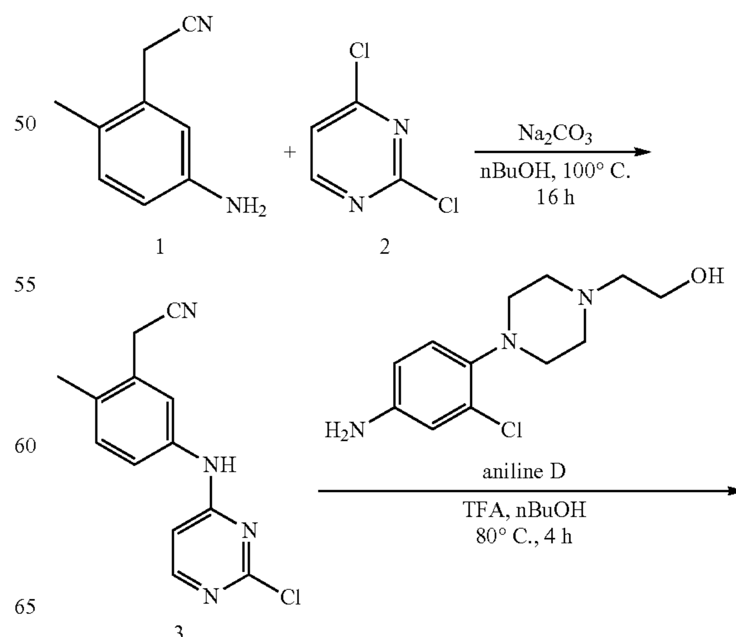
Scheme-16
