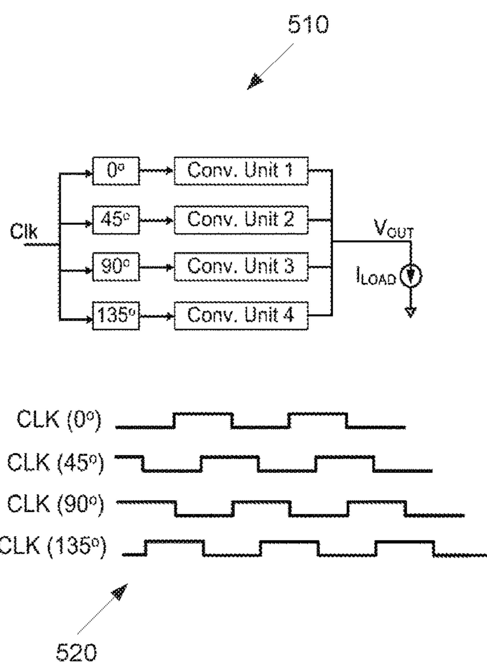
FIG. 5B
