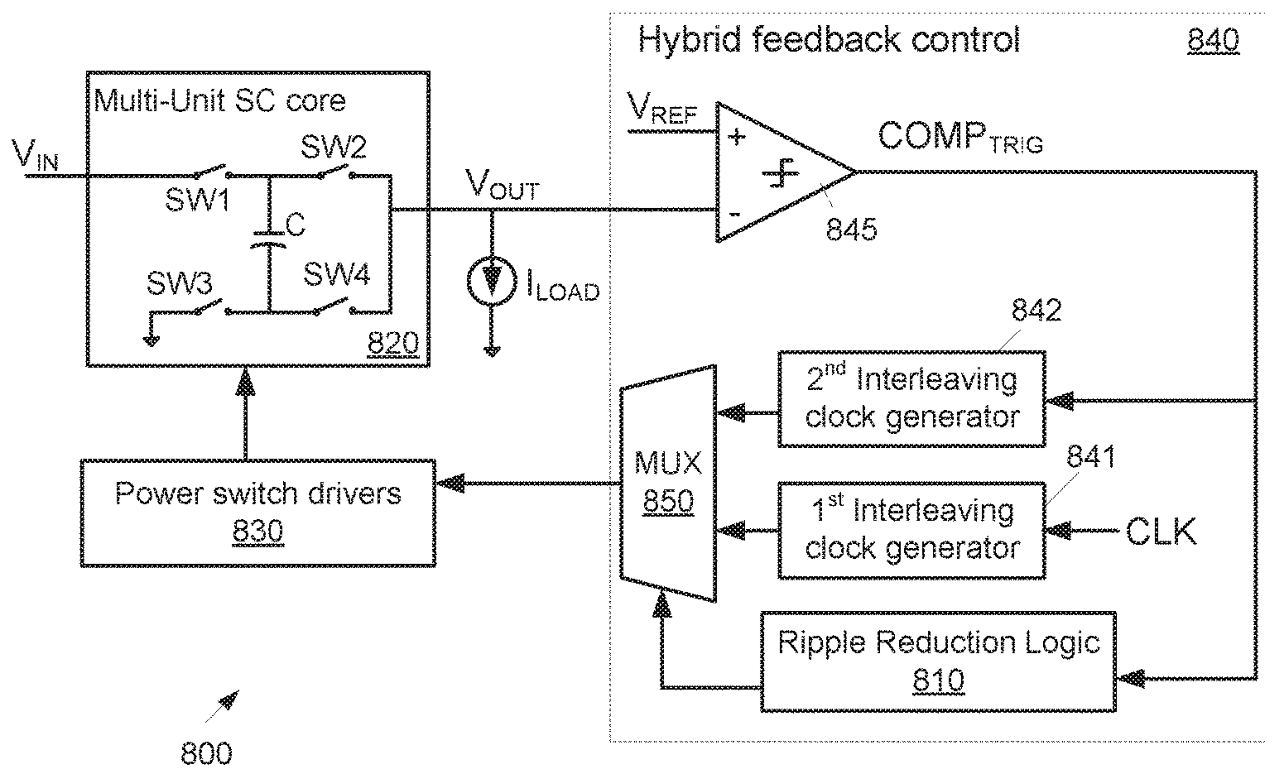
FIG. 8B
