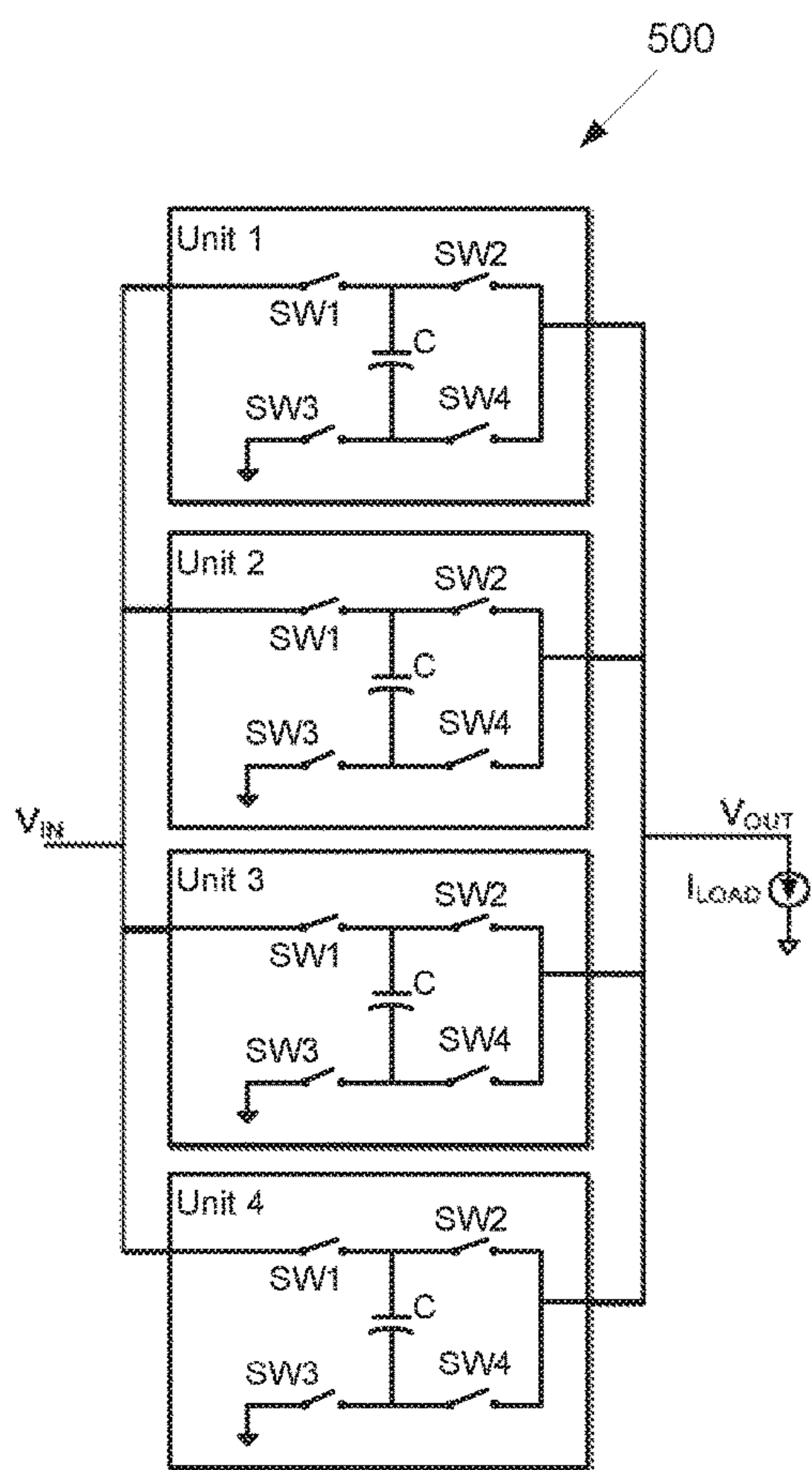
FIG. 5A
