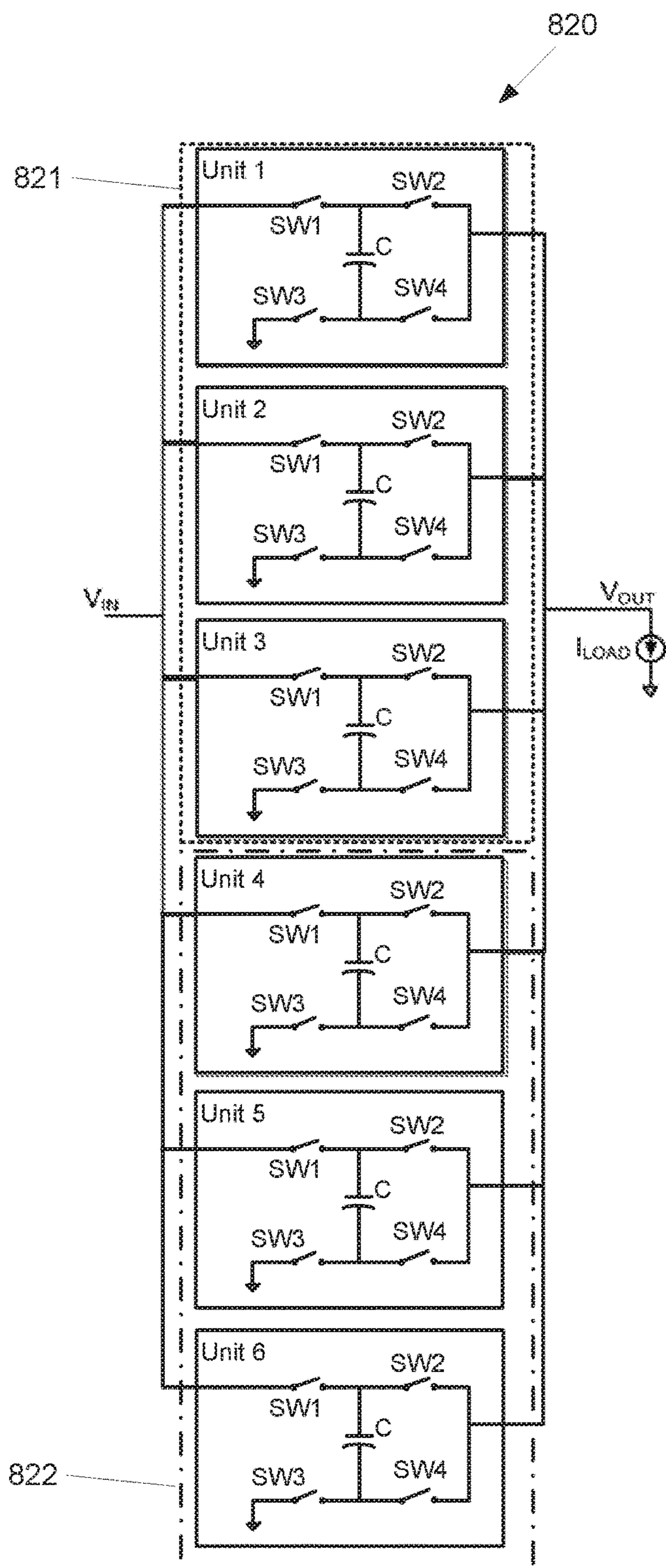
FIG. 8C
