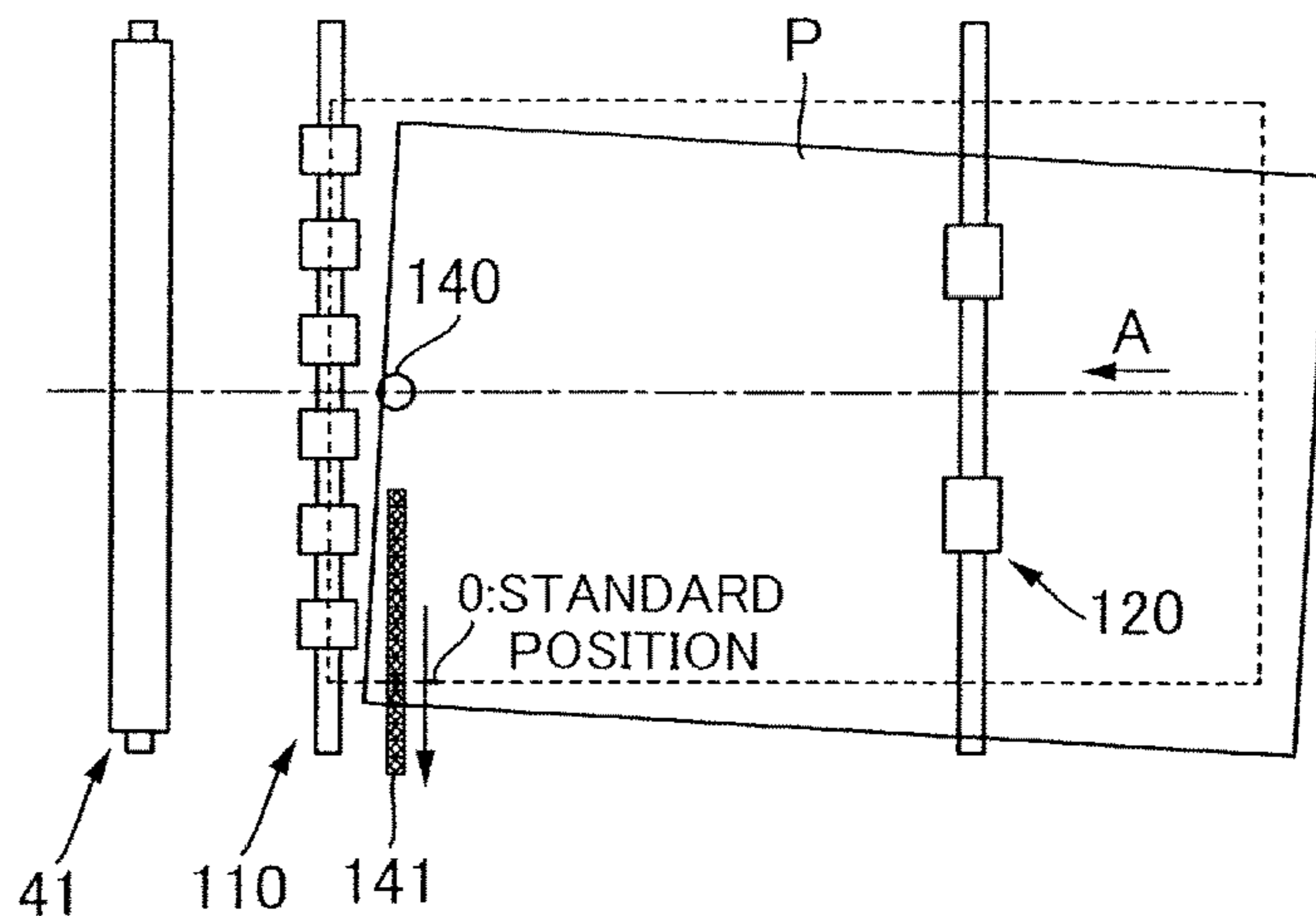
FIG.5B
