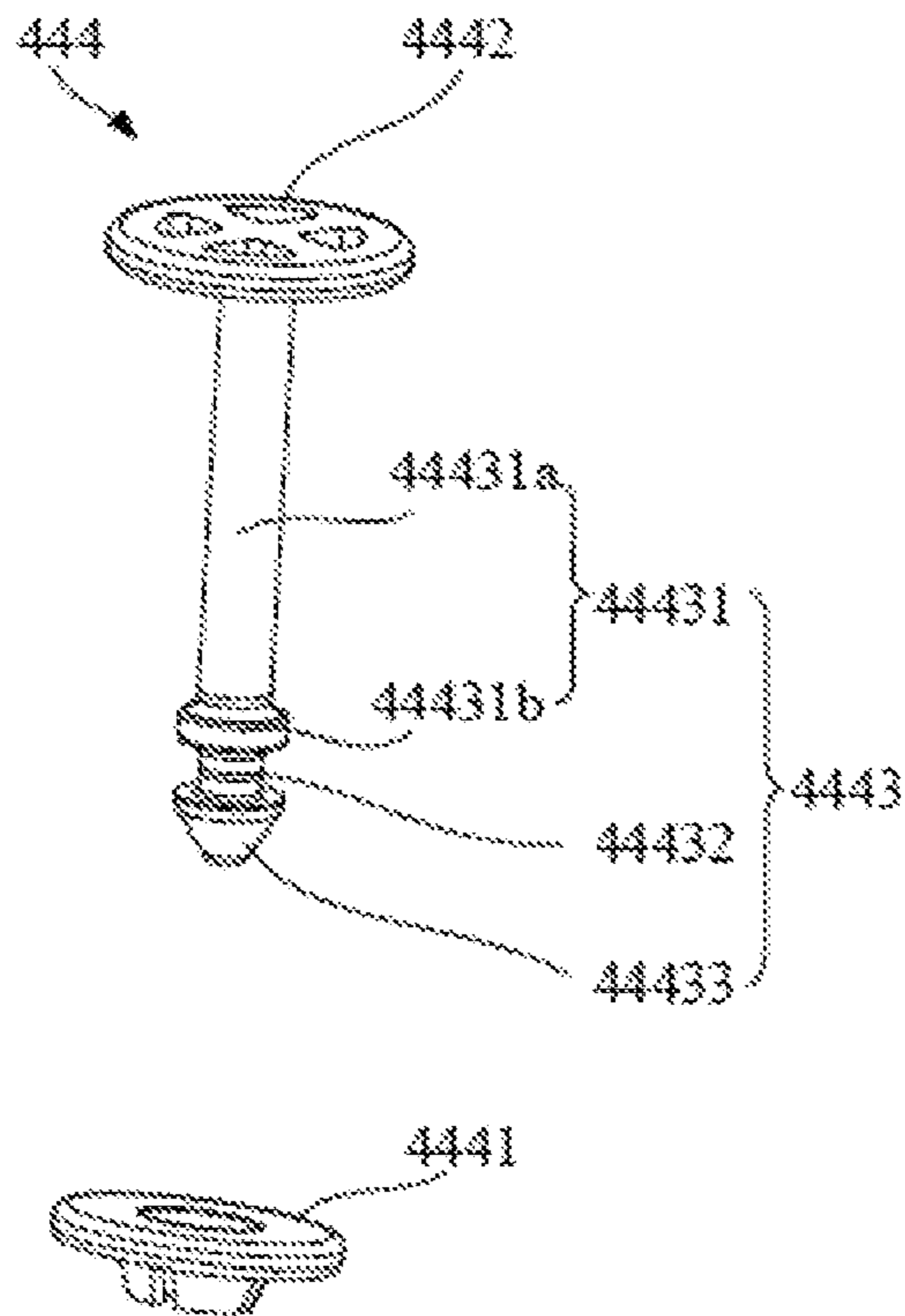
FIG. 15
