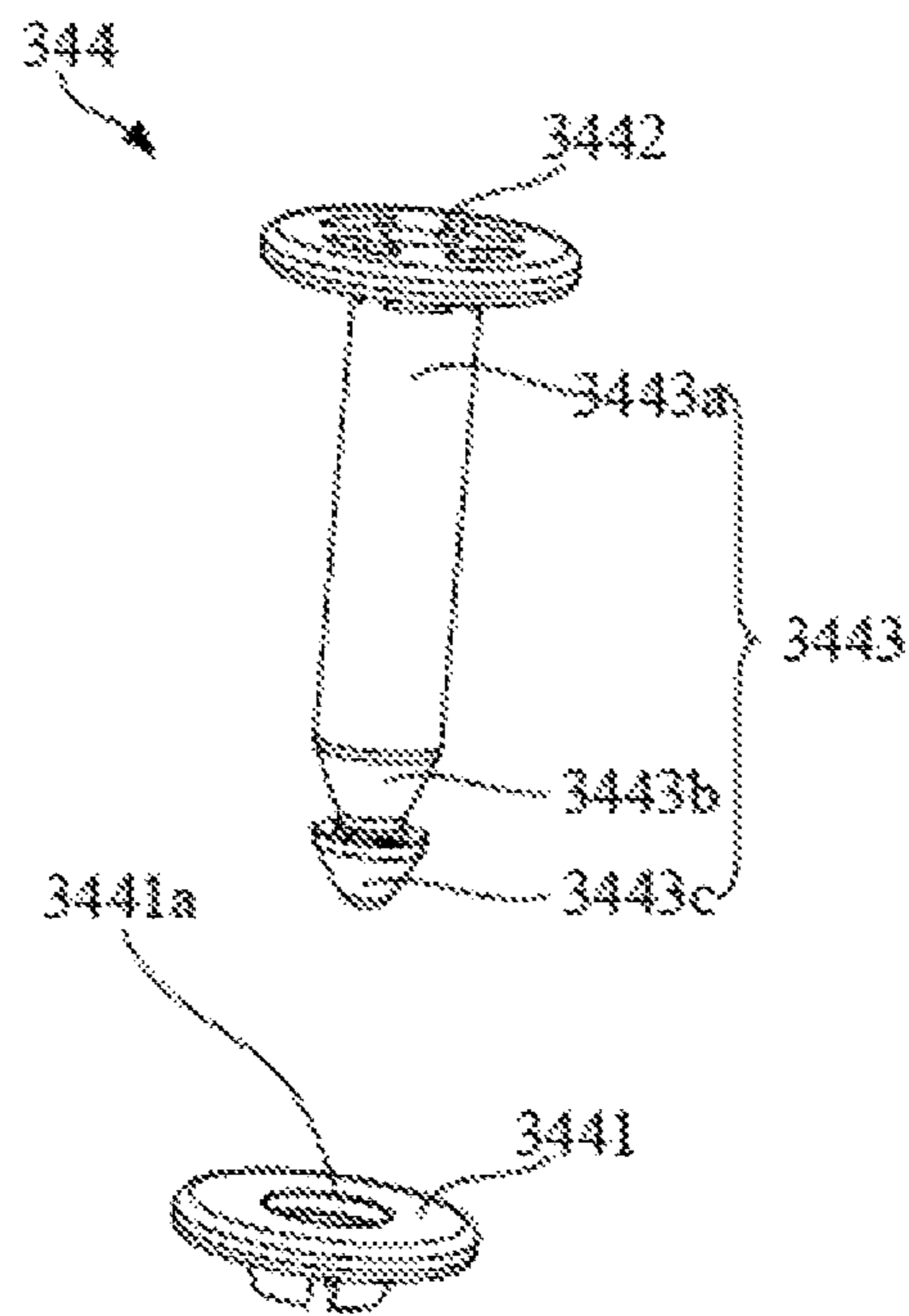
FIG. 14
