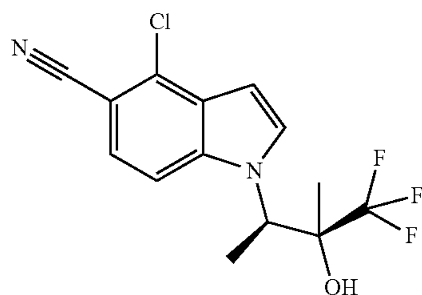
4-Chloro-1-((2R,3S)-4,4,4-trifluoro-3-hydroxy-3-methylbutan-2-yl)-1H-indole-5-carbonitrile
