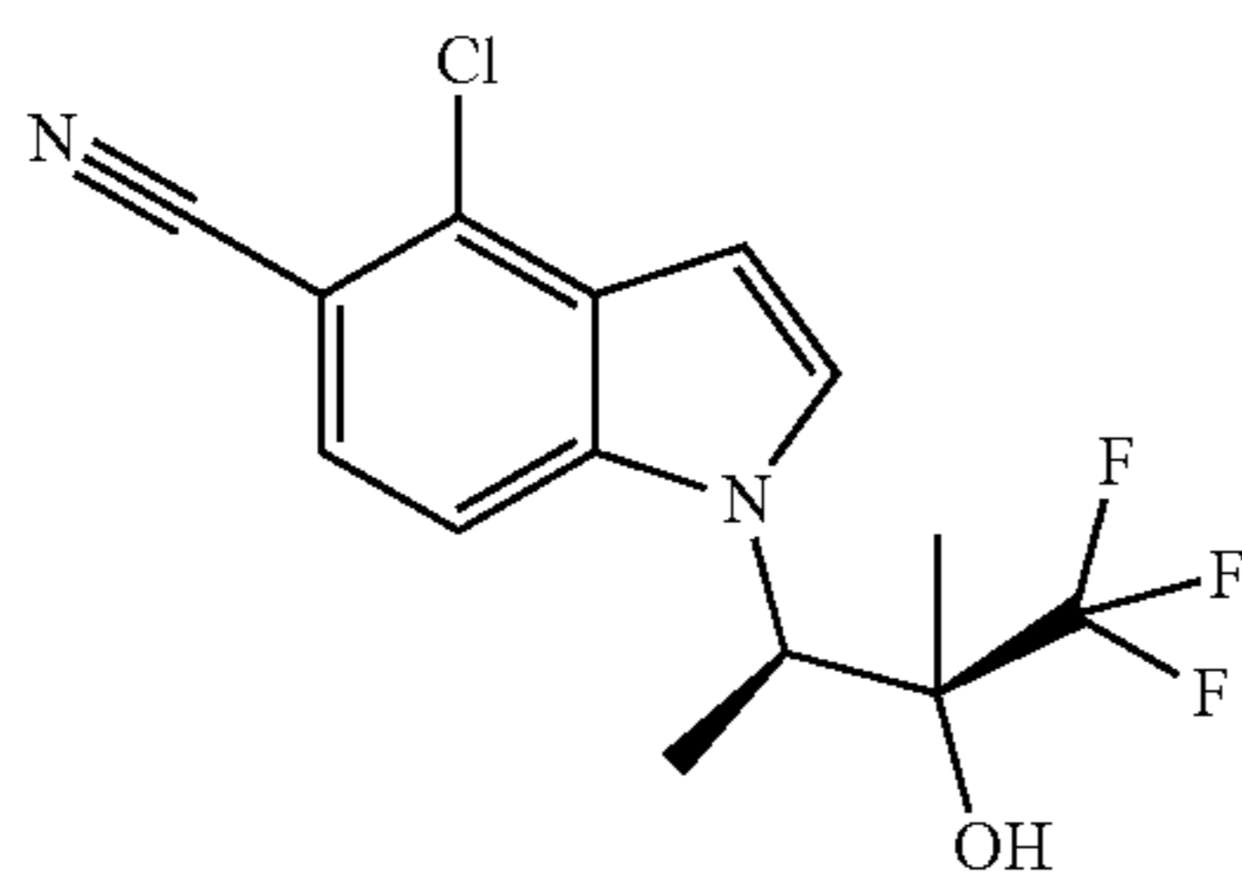
D. 4-Chloro-1-((2R,3S)-4,4,4-trifluoro-3-hydroxy-3-methylbutan-2-yl)-1H-indole-5-carbonitrile
