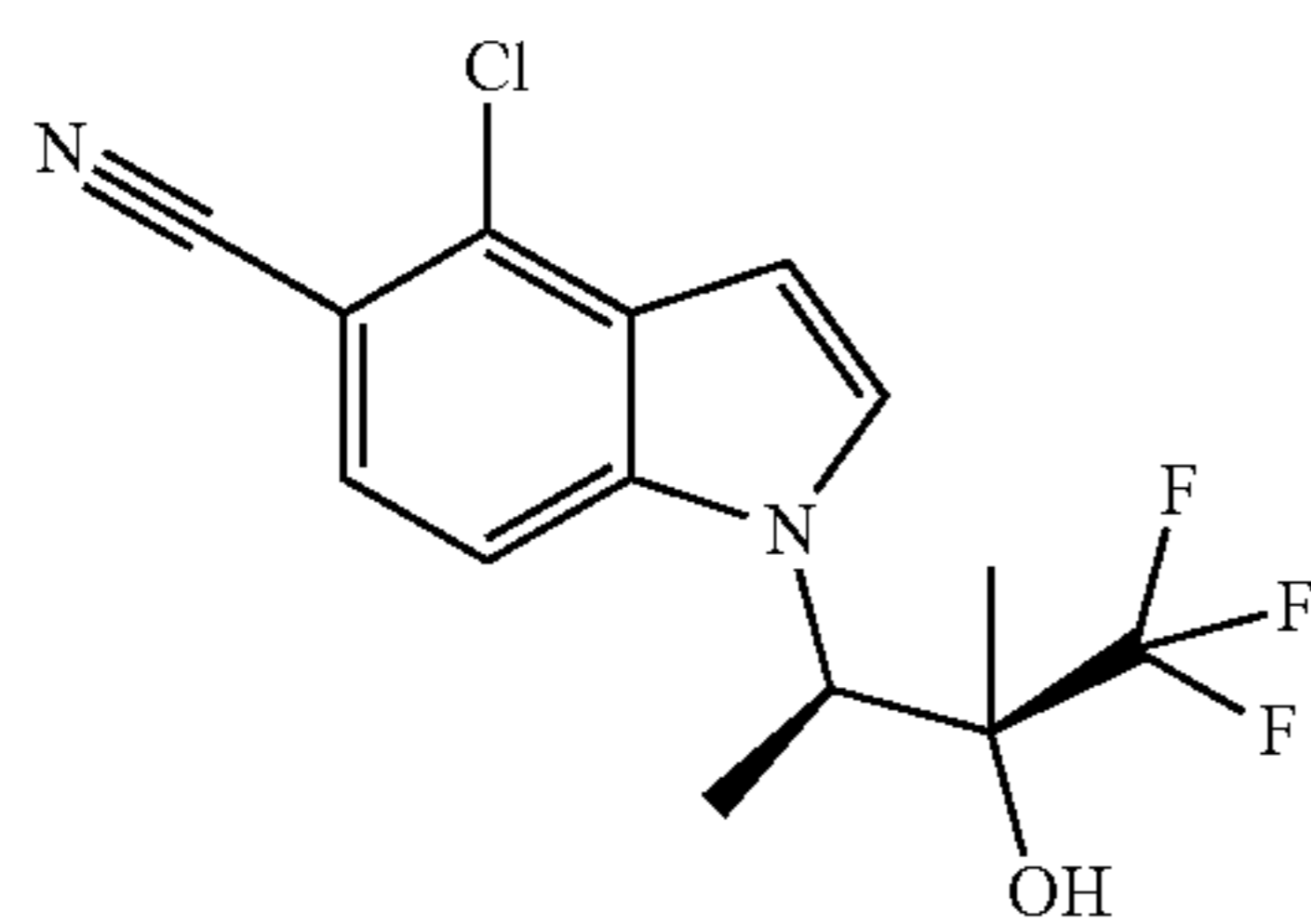
4-Chloro-1-((2R,3S)-4,4,4-trifluoro-3-hydroxy-3-methylbutan-2-yl)-1H-indole-5-carbonitrile
