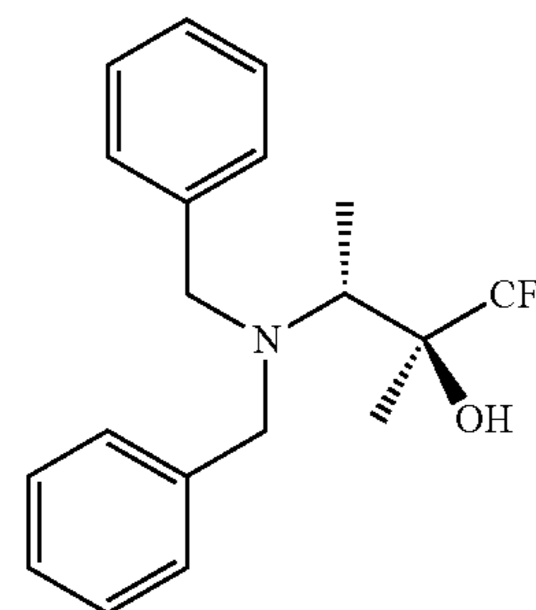
B. (2S,3R)-3-(Dibenzylamino)-1,1,1-trifluoro-2-methylbutan-2-ol
