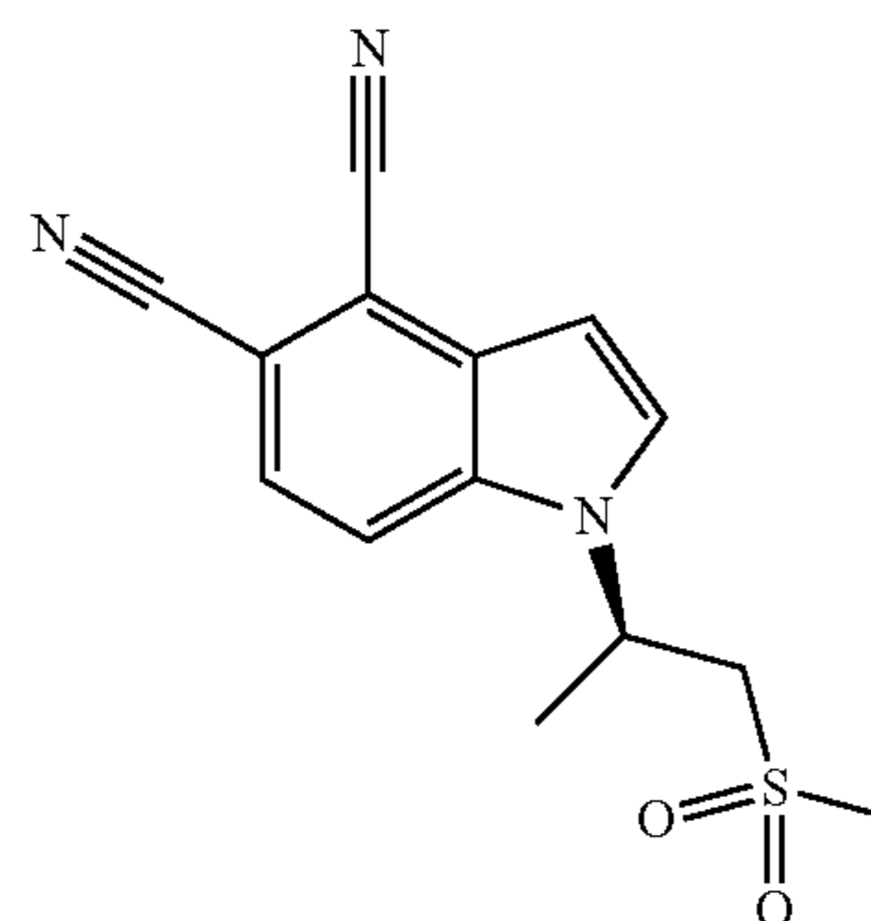
(R)-1-(1-(Methylsulfonyl)propan-2-yl)-1H-indole-4,5-dicarbonitrile
