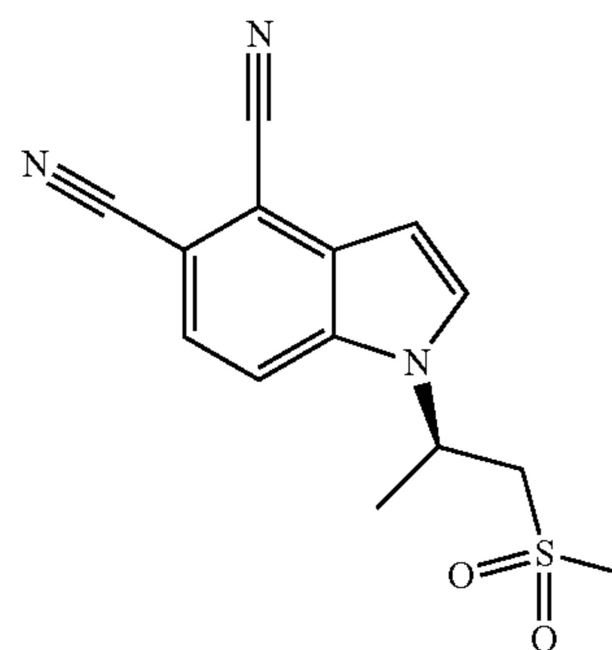
(R)-1-(1-(Methylsulfonyl)propan-2-yl)-1H-indole-4,5-dicarbonitrile
