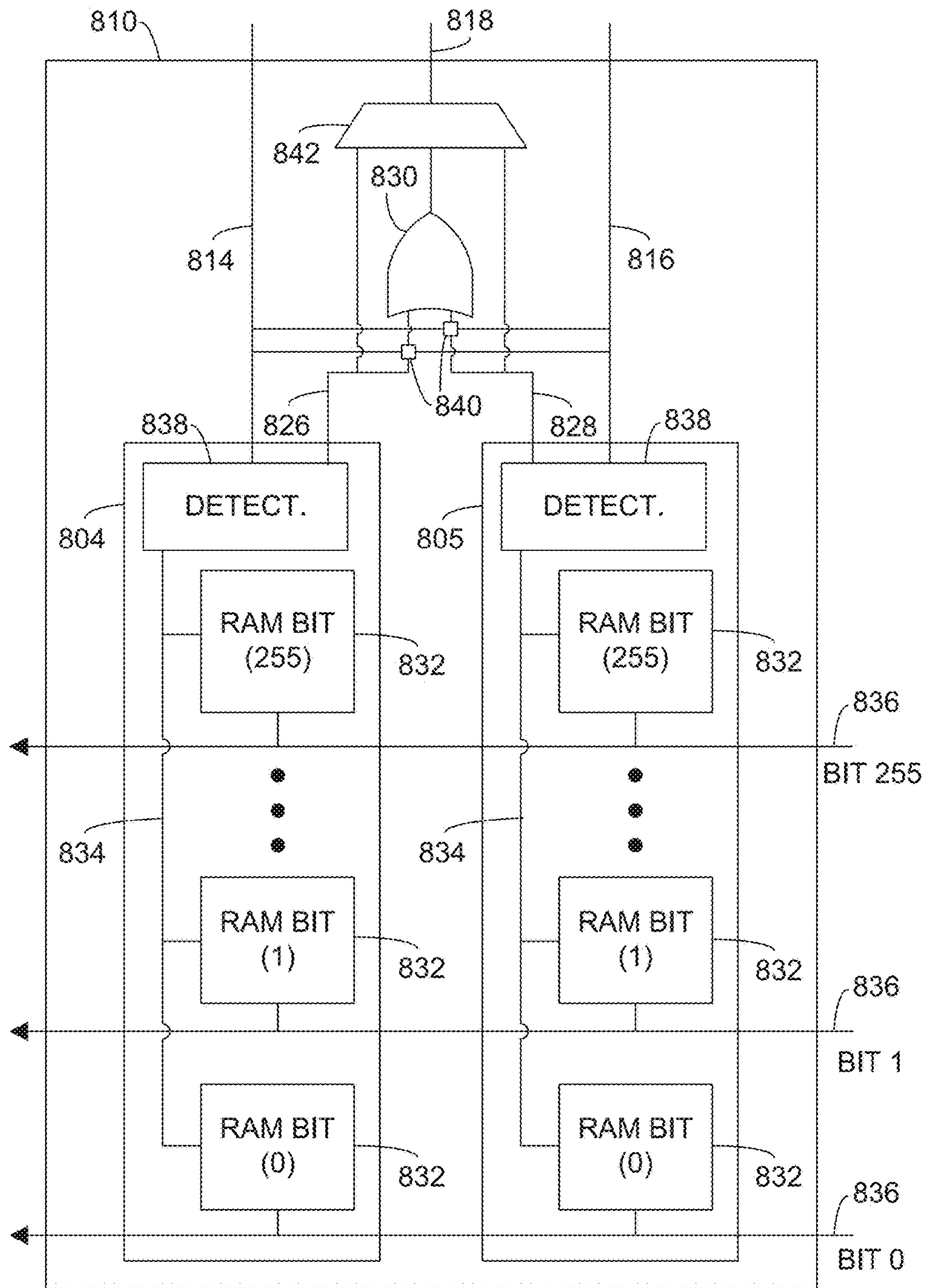
FIG. 18
