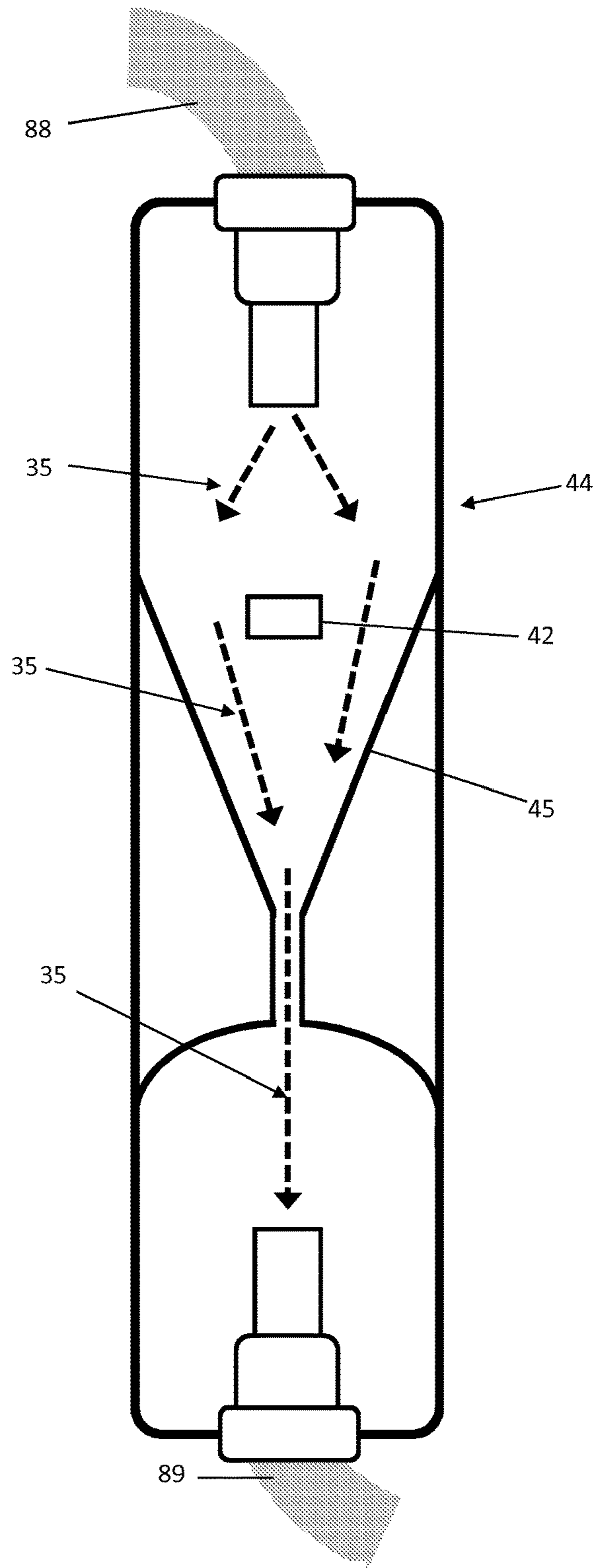
FIG. 10
