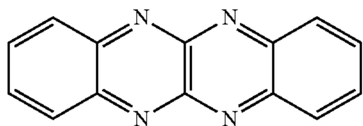
quinoxalino[2,3-b]quinoxaline
