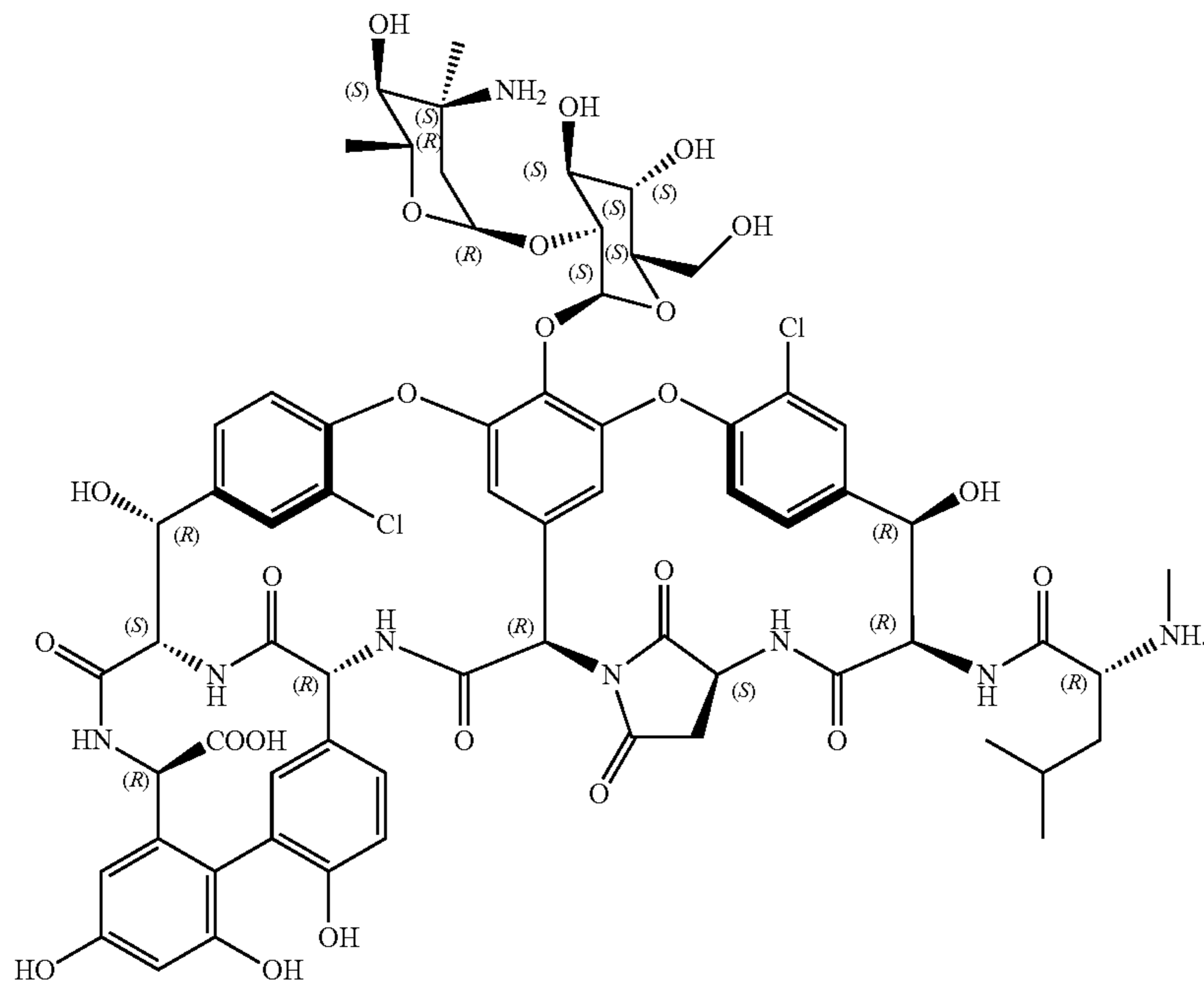
DAmS (Des-(amido)-succinimido-VancomycinB)
