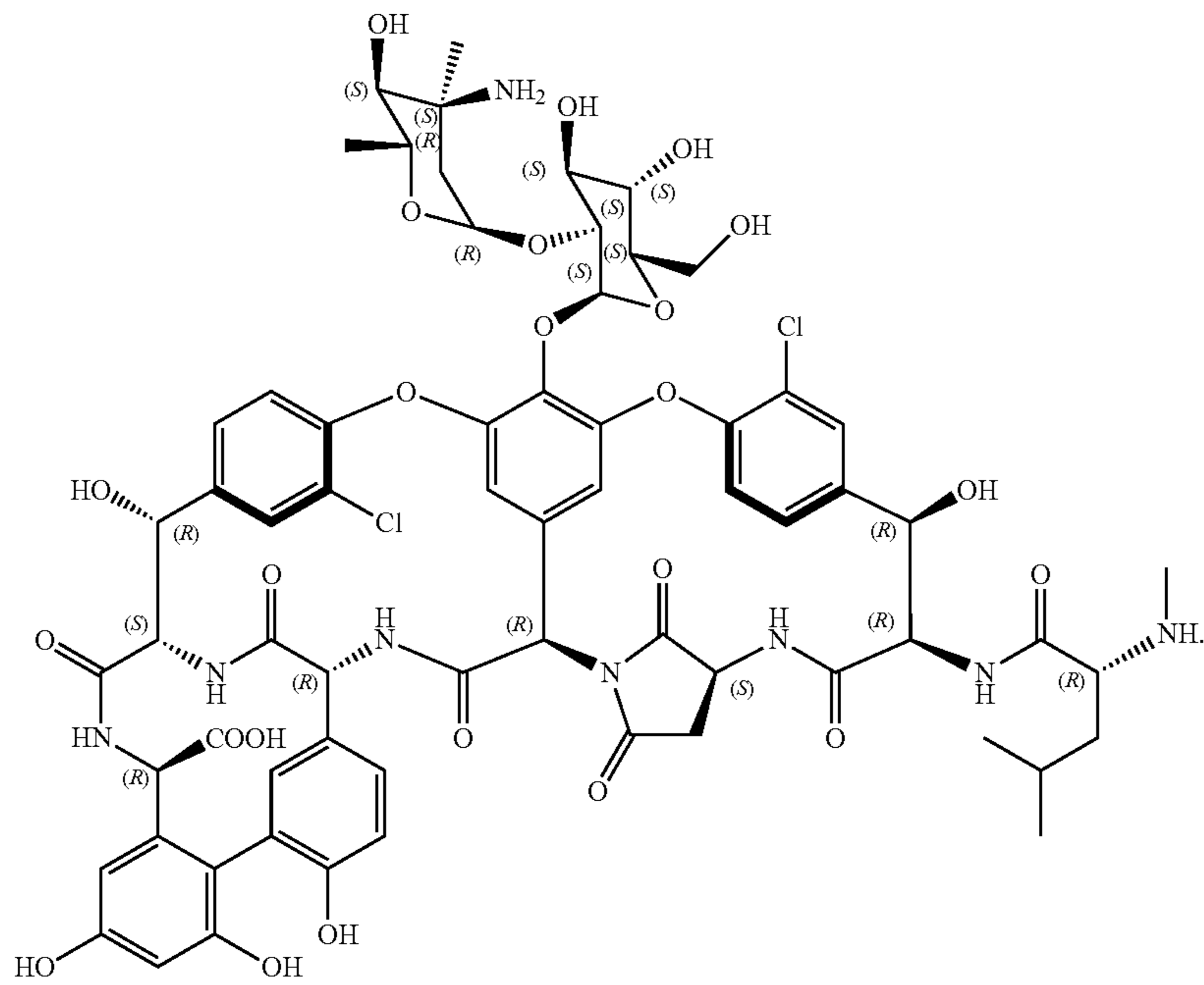
DAmS (Des-(amido)-succinimido-VancomycinB)
