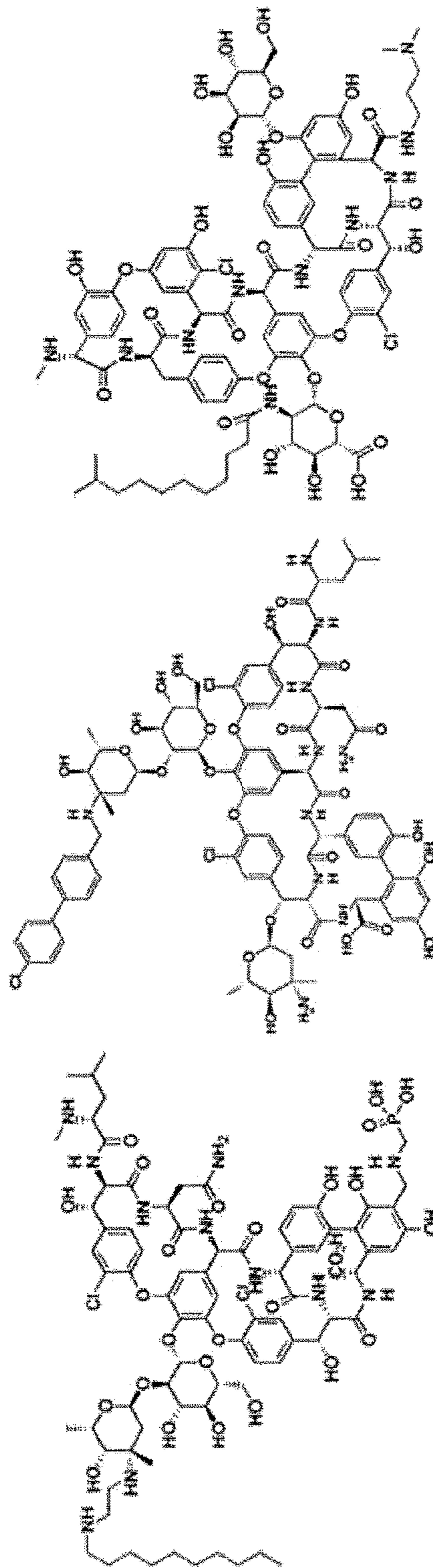
Telavancin
