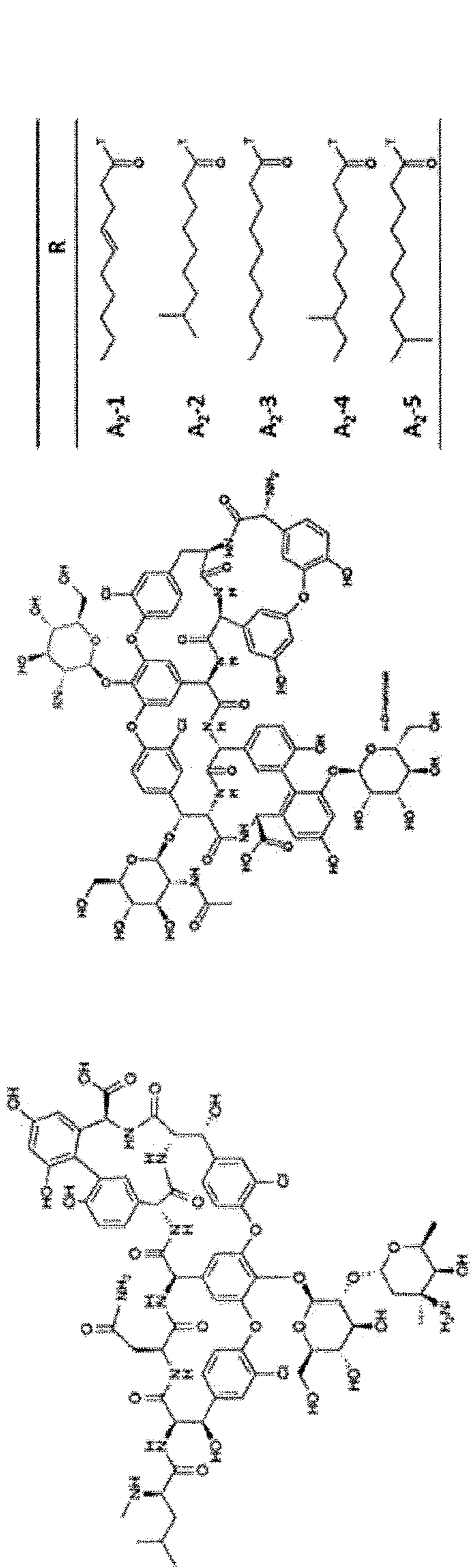
Vancomycin
