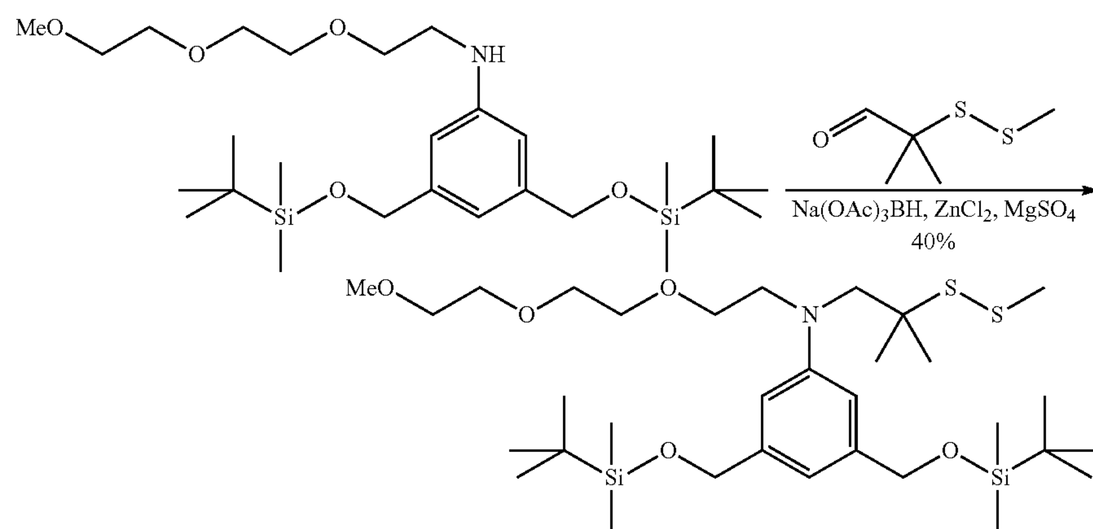
3,5-bis(((tert-butyldimethylsilyl)oxy)methyl)-N-(2-(2-(2-methoxyethoxy)ethoxy)ethyl)-N-(2-methyl-2-(methylthio)propyl)aniline
