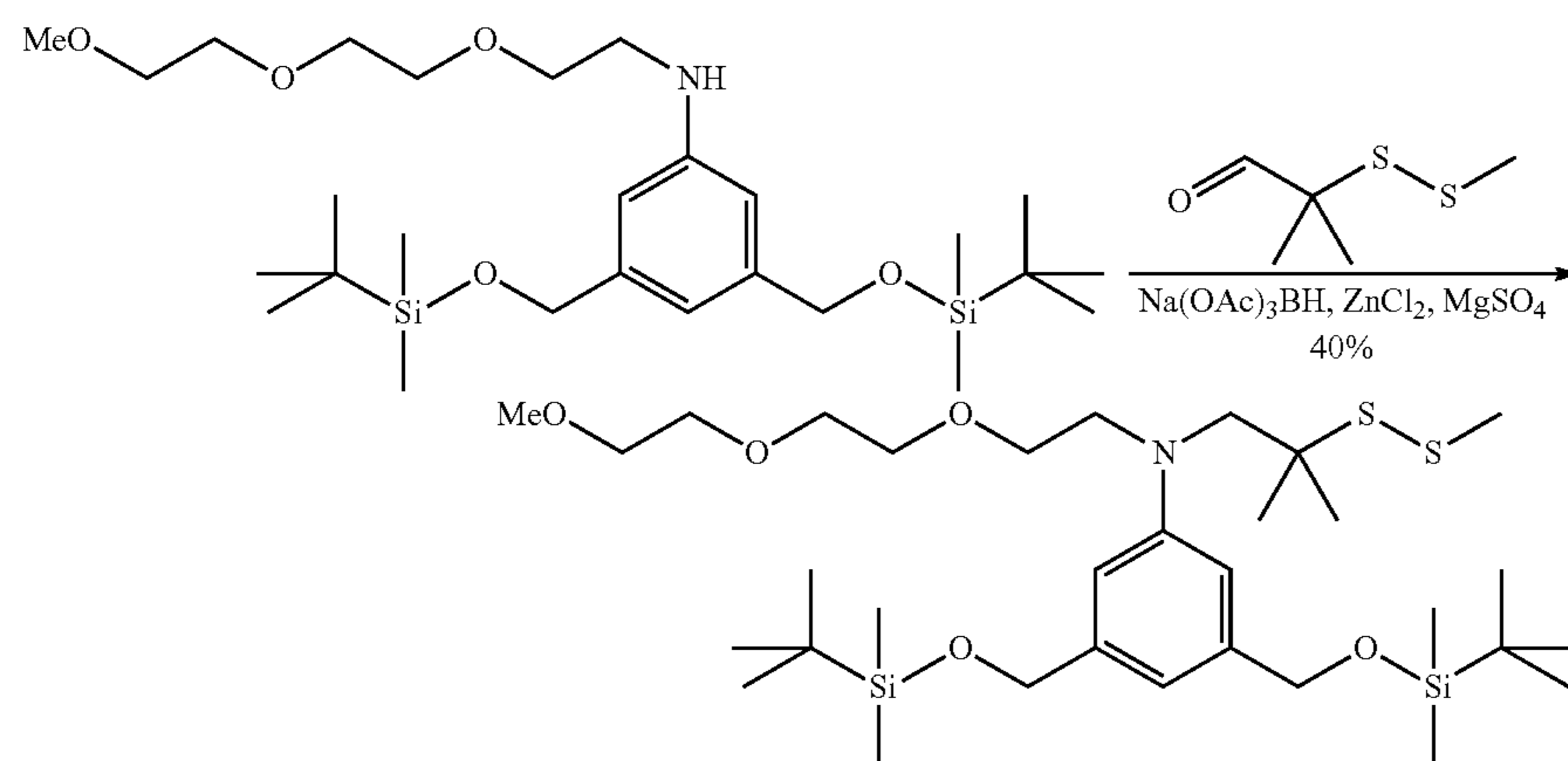
3,5-bis(((tert-butyldimethylsilyl)oxy)methyl)-N-(2-(2-(2-methoxyethoxy)ethoxy)ethyl)-N-(2-methyl-2-(methylthio)ethyl)aniline
