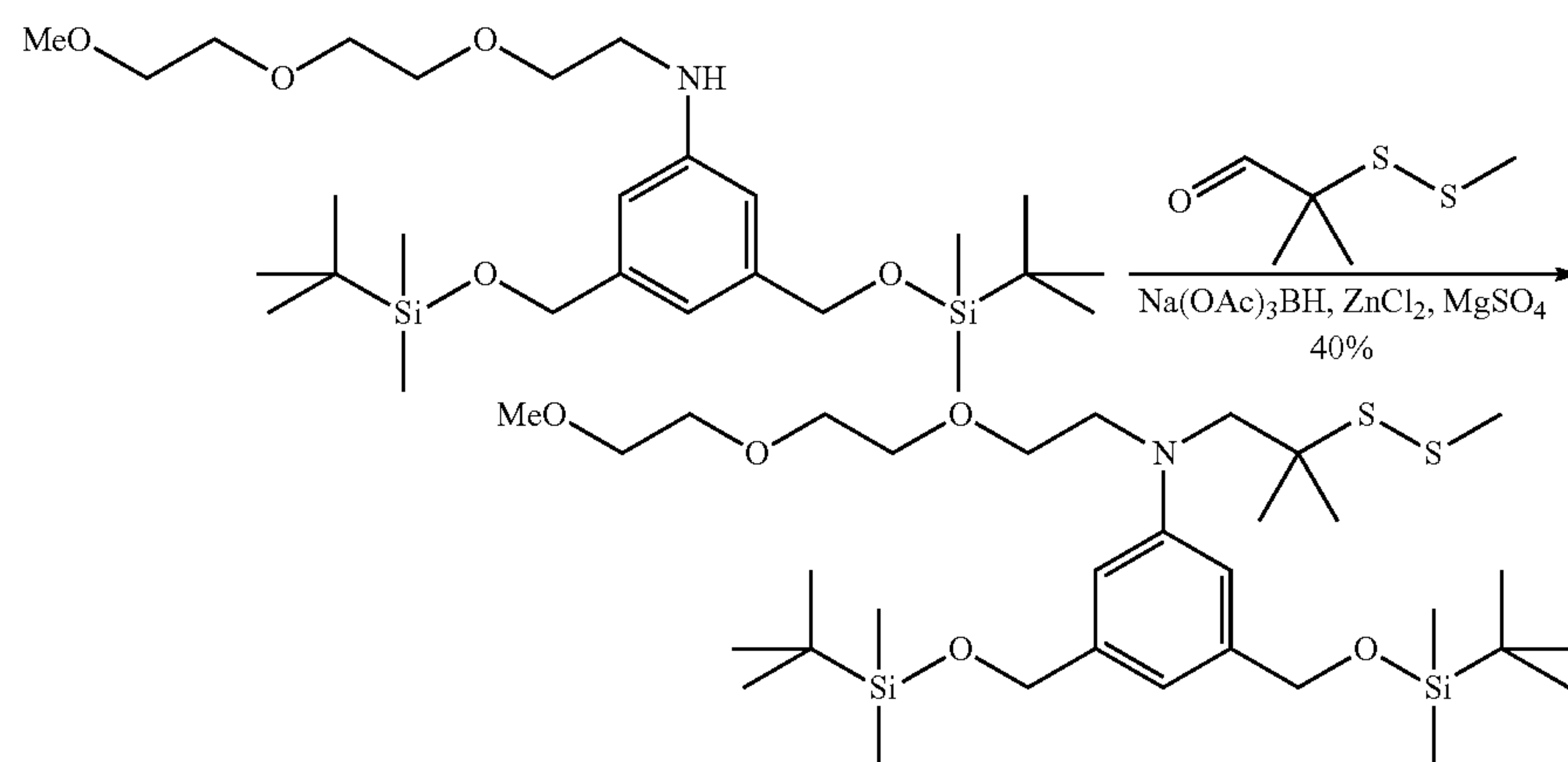
3,5-bis(((tert-butyldimethylsilyl)oxy)methyl)-N-(2-(2-(2-methoxyethoxy)ethoxy)ethyl)-N-(2-methyl-2-(methylthio)ethyl)propyl)aniline
