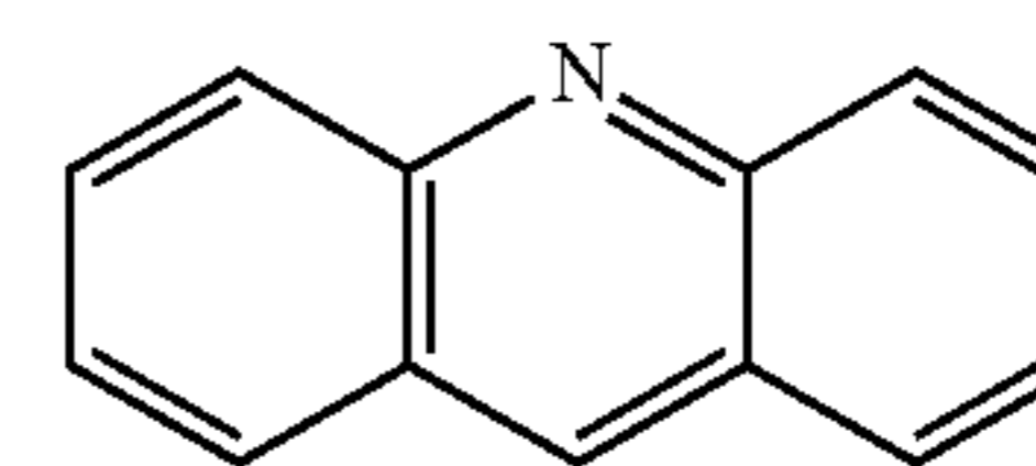
Acridine
