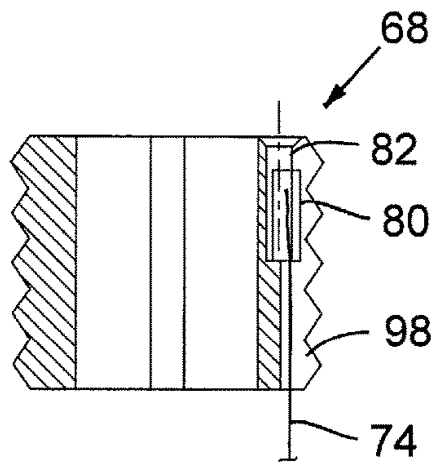
FIG. 5A
