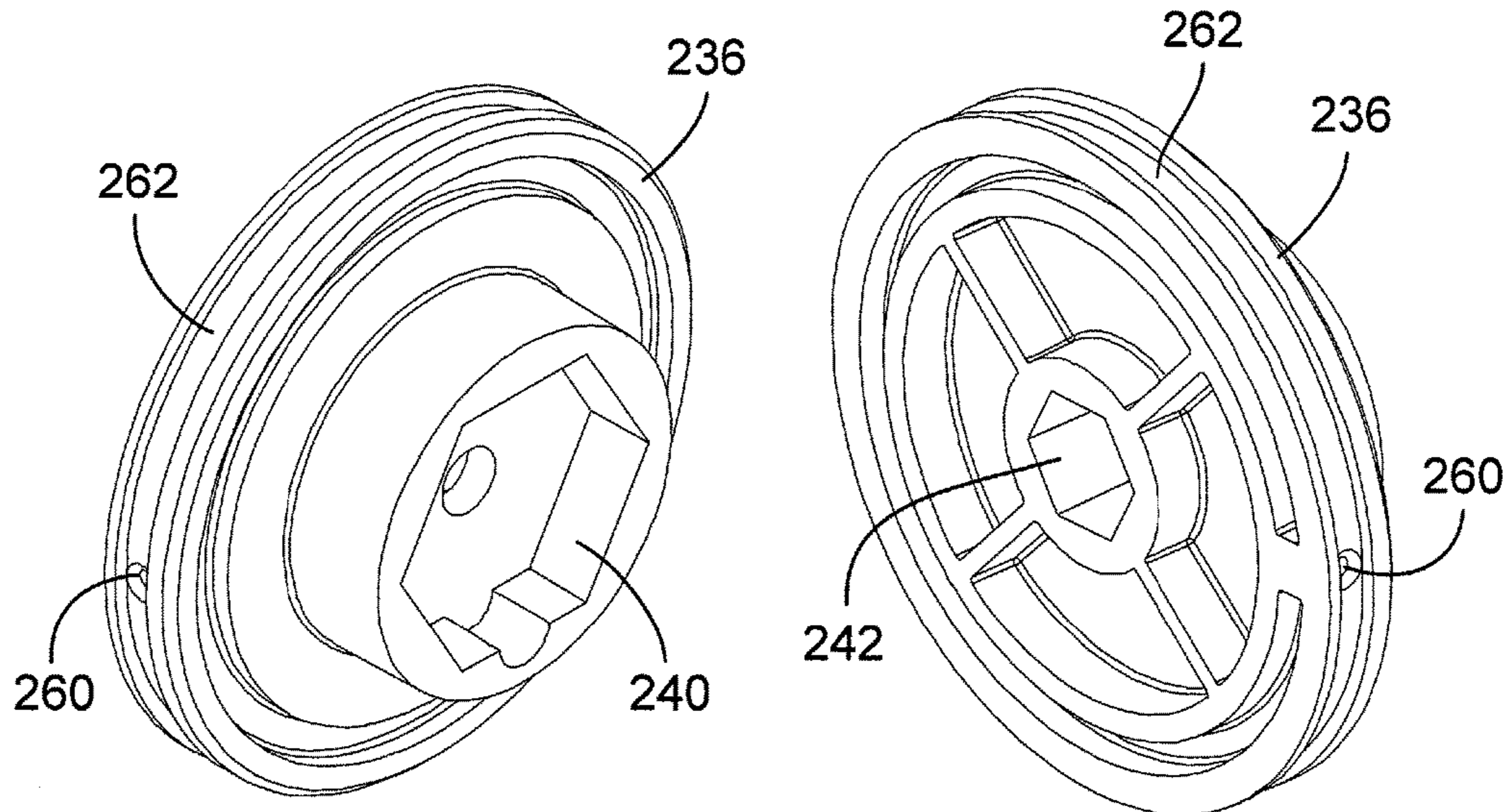
FIG. 16A
