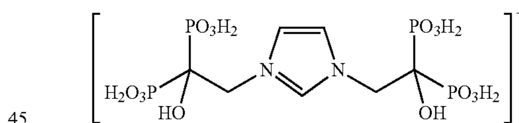
Ion 2
