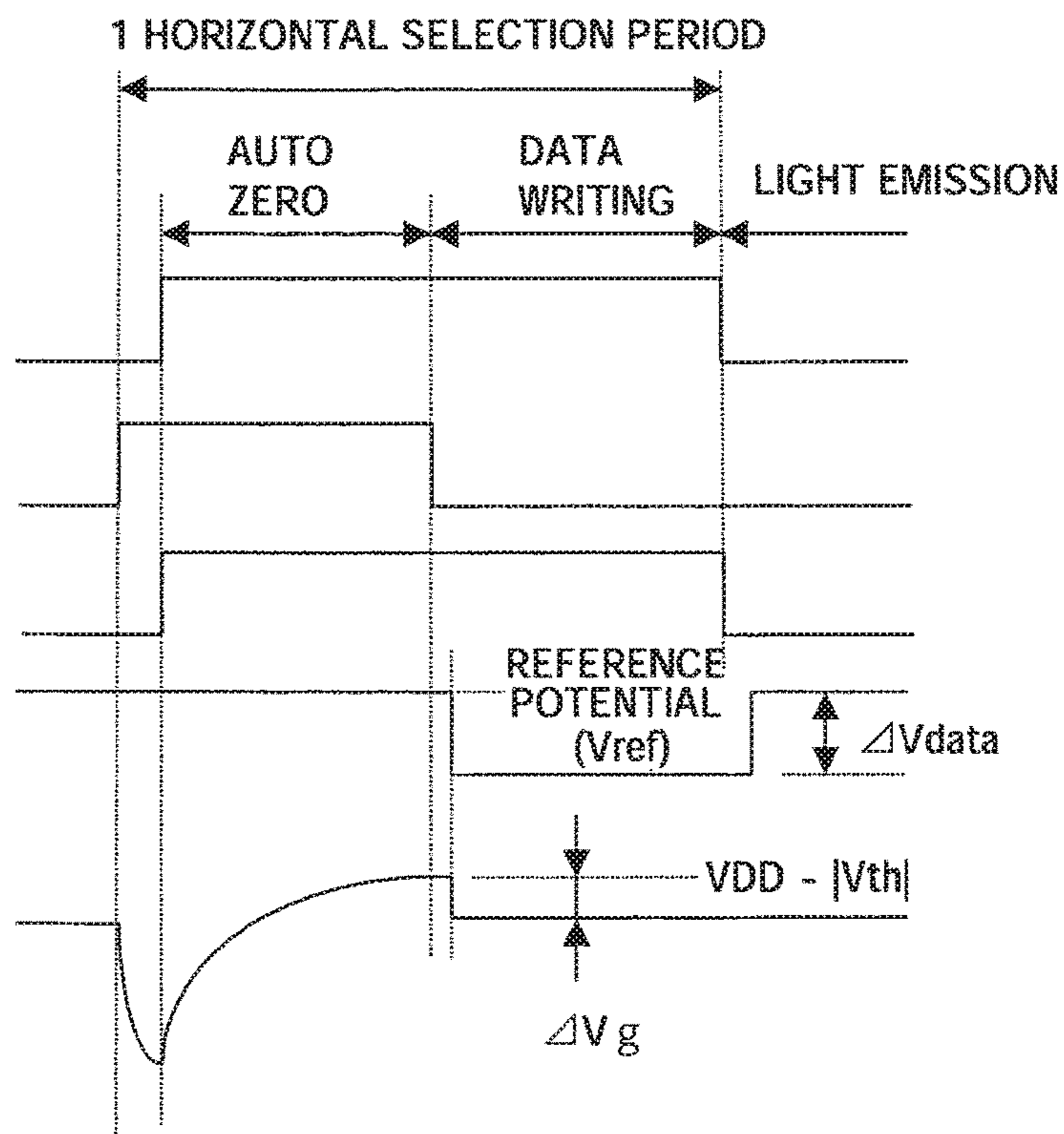
FIG. 4E V_g (TFT21)
