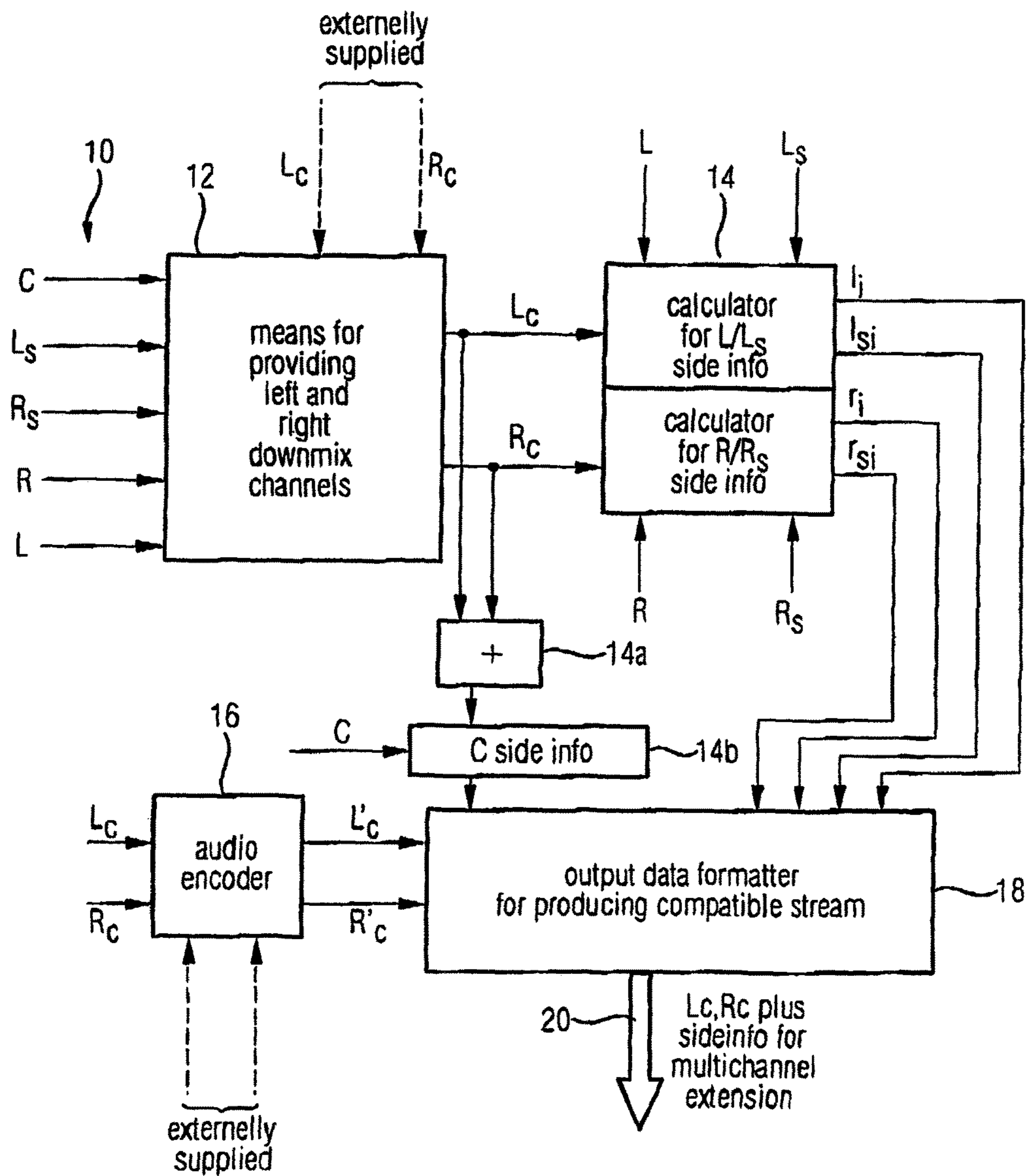
FIG 1 (Encoder)
