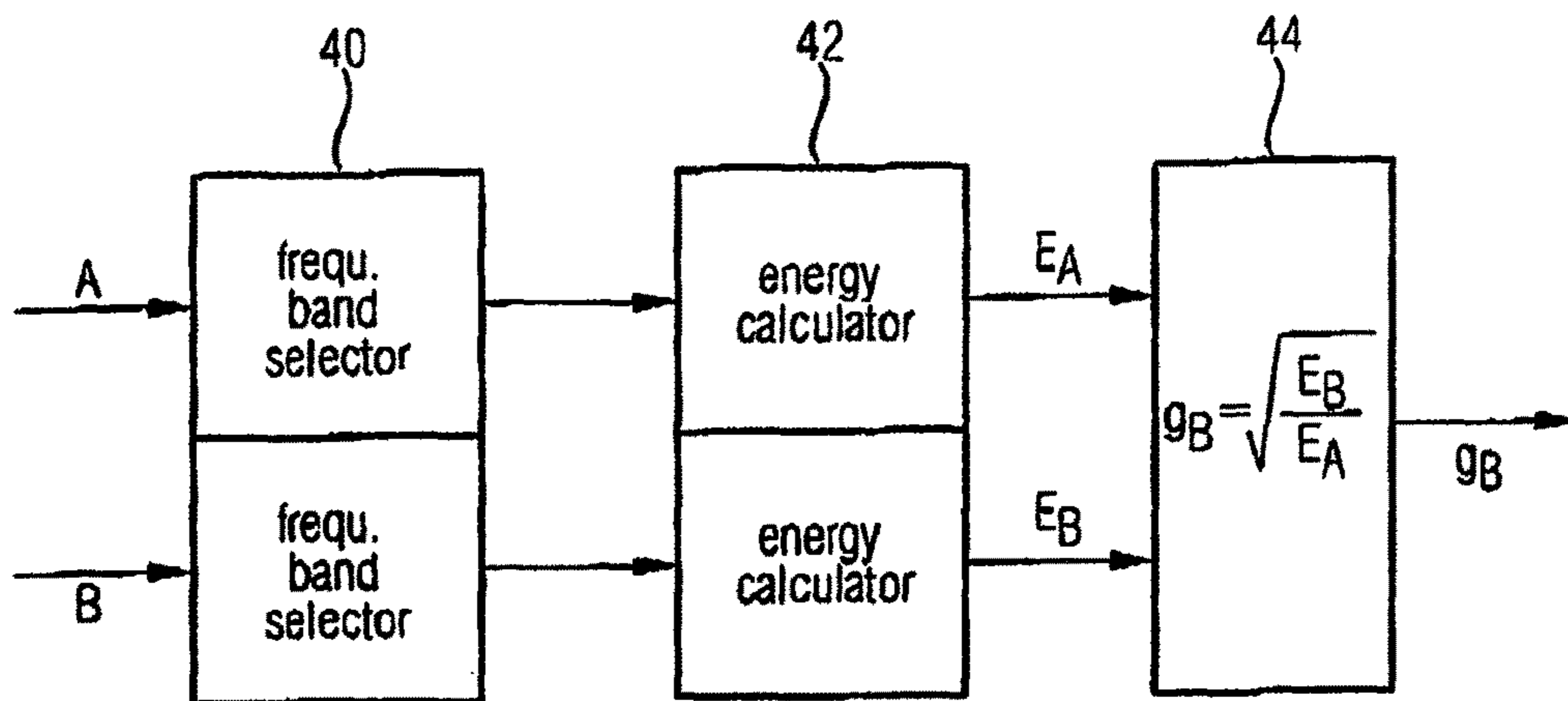
FIG 4 (encoder side)
