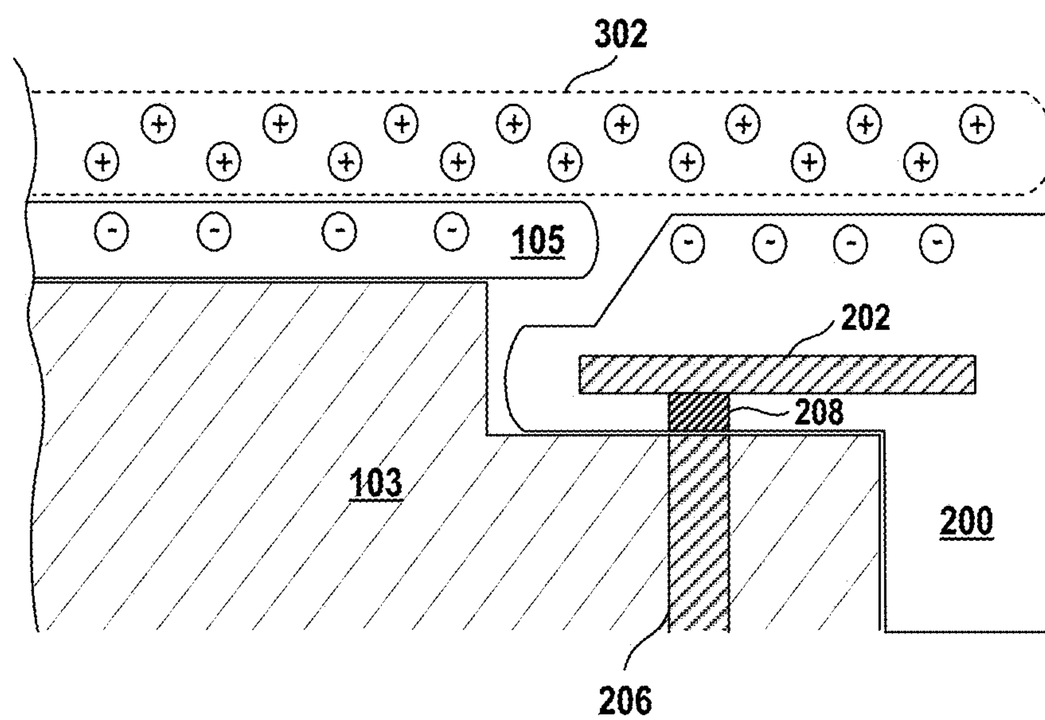
FIG. 3B
