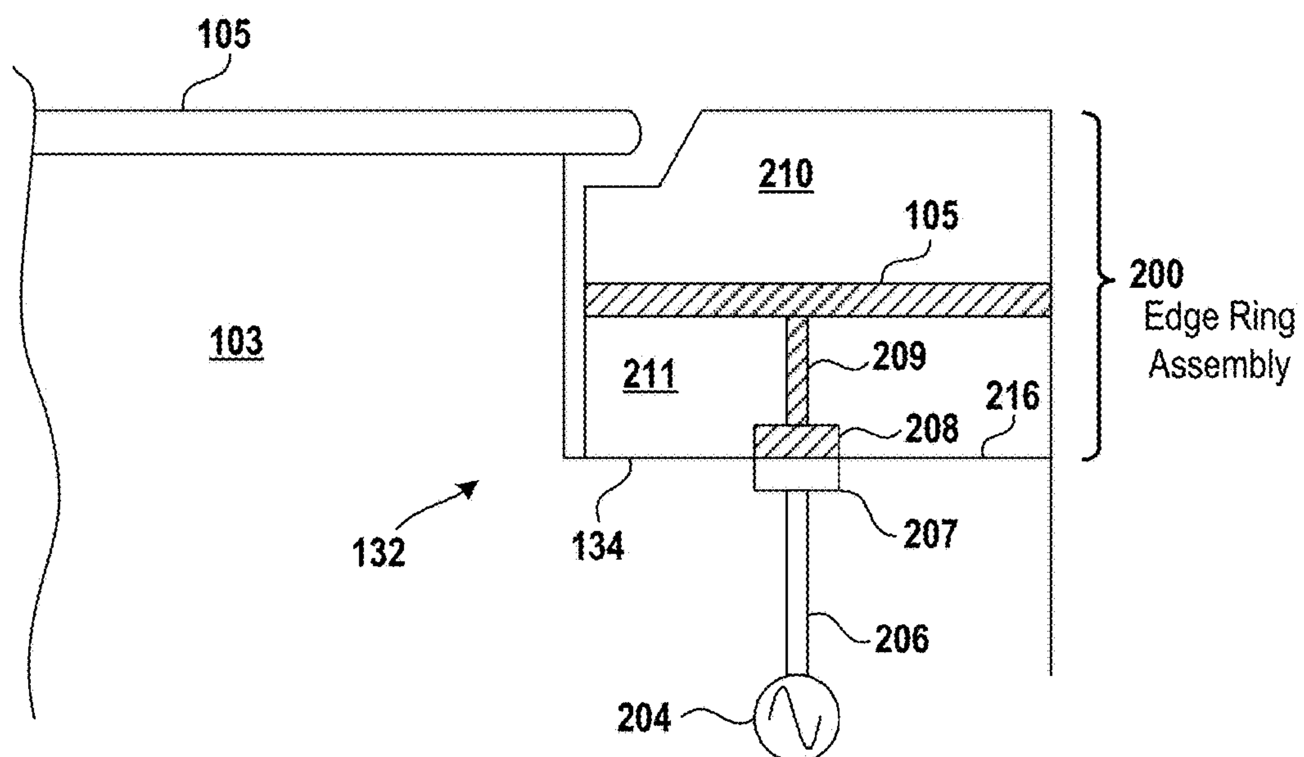
FIG. 2C
