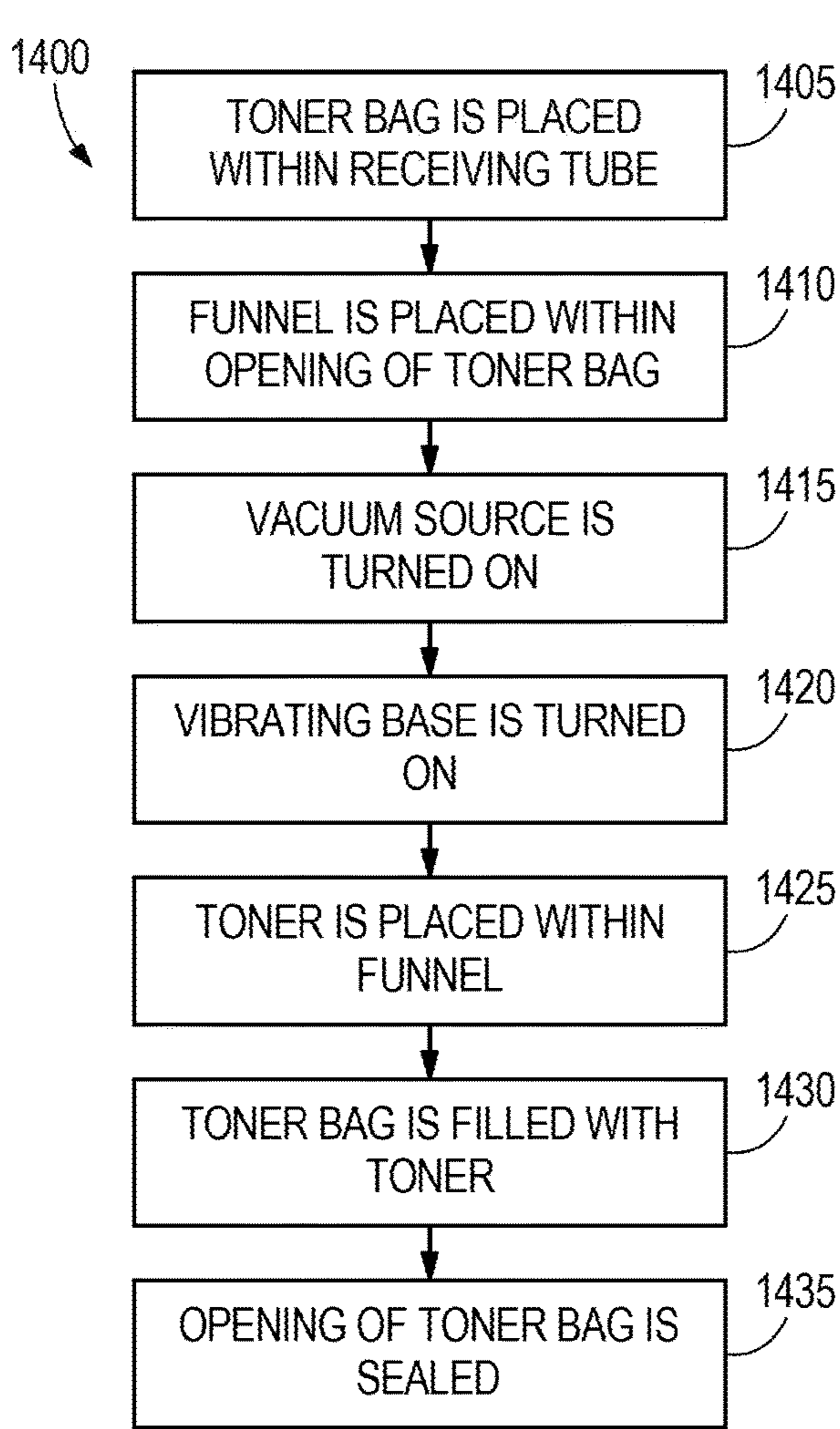
FIG. 13
