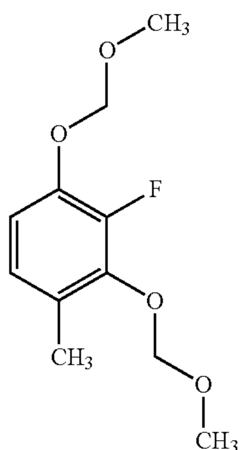
2-fluoro-1,3-bis(methoxymethoxy)-4-methyl-benzene
