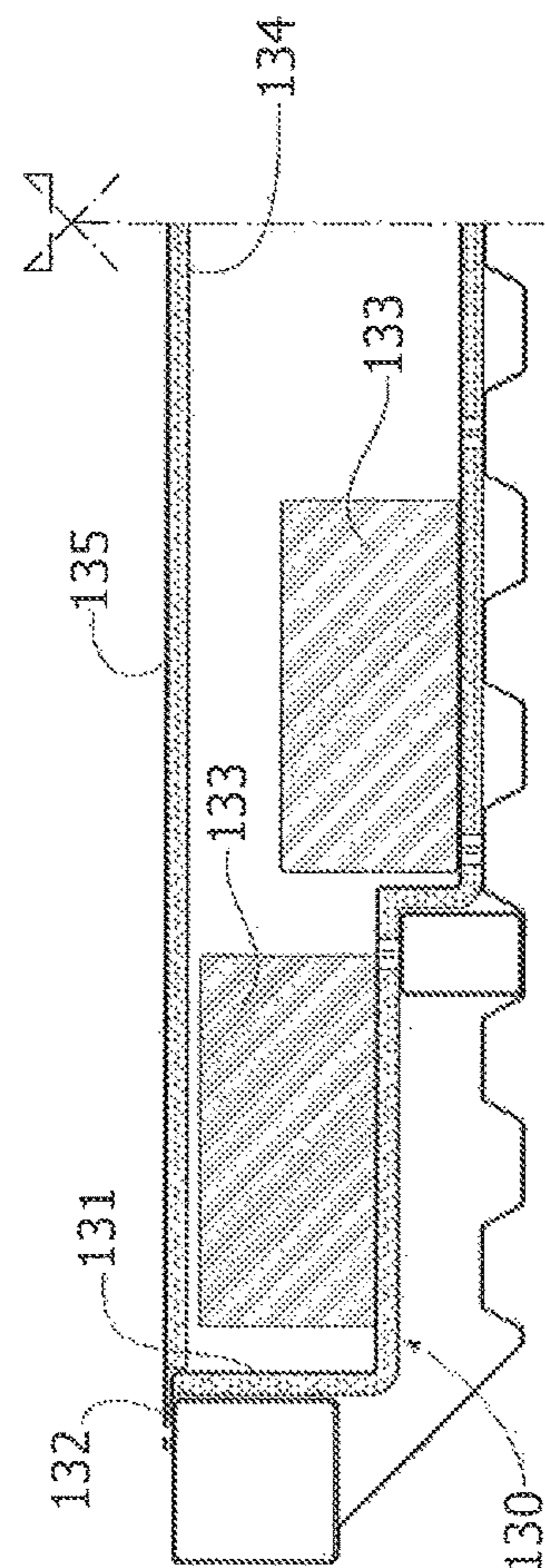
FIG. 10
