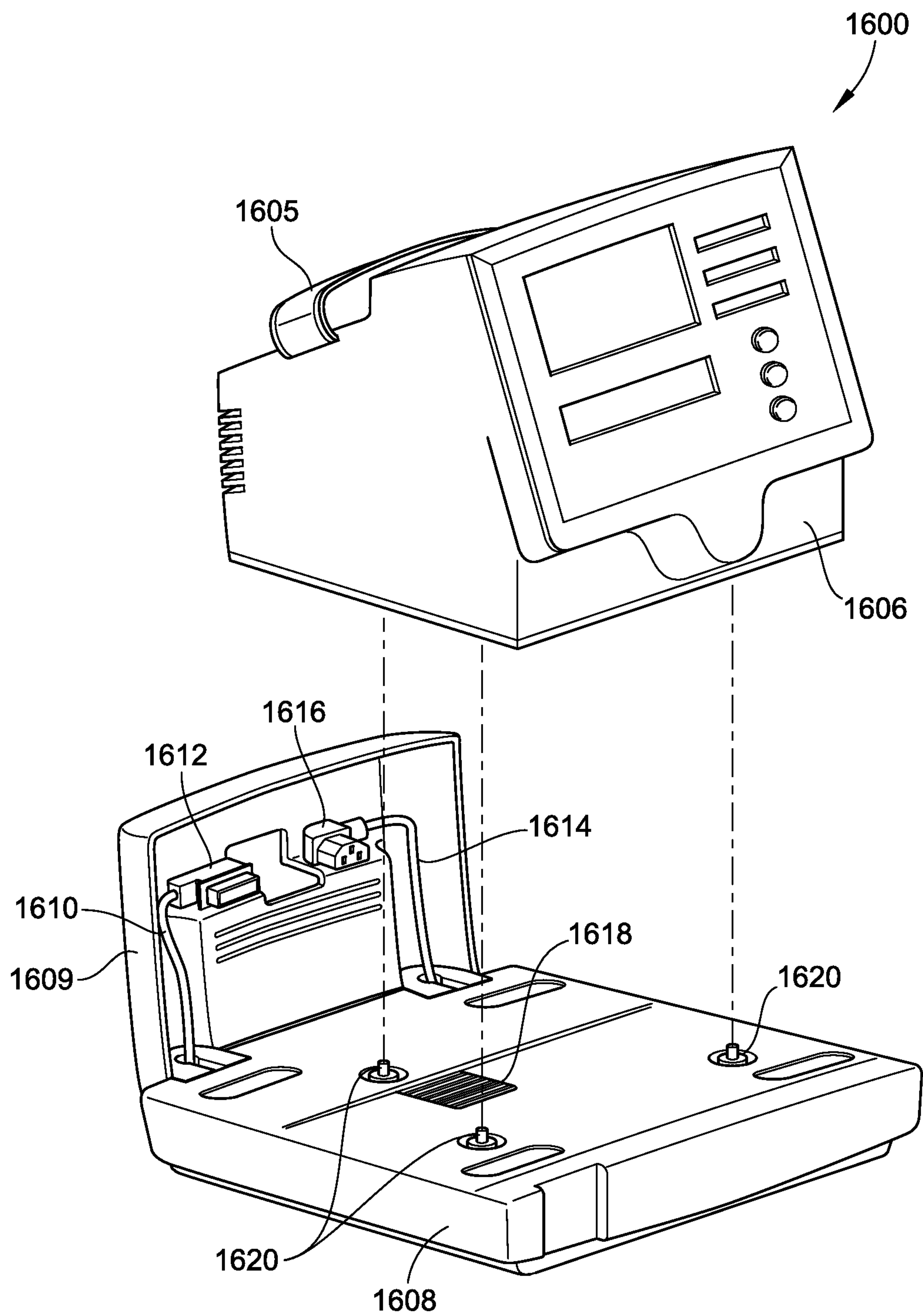
FIG. 29
