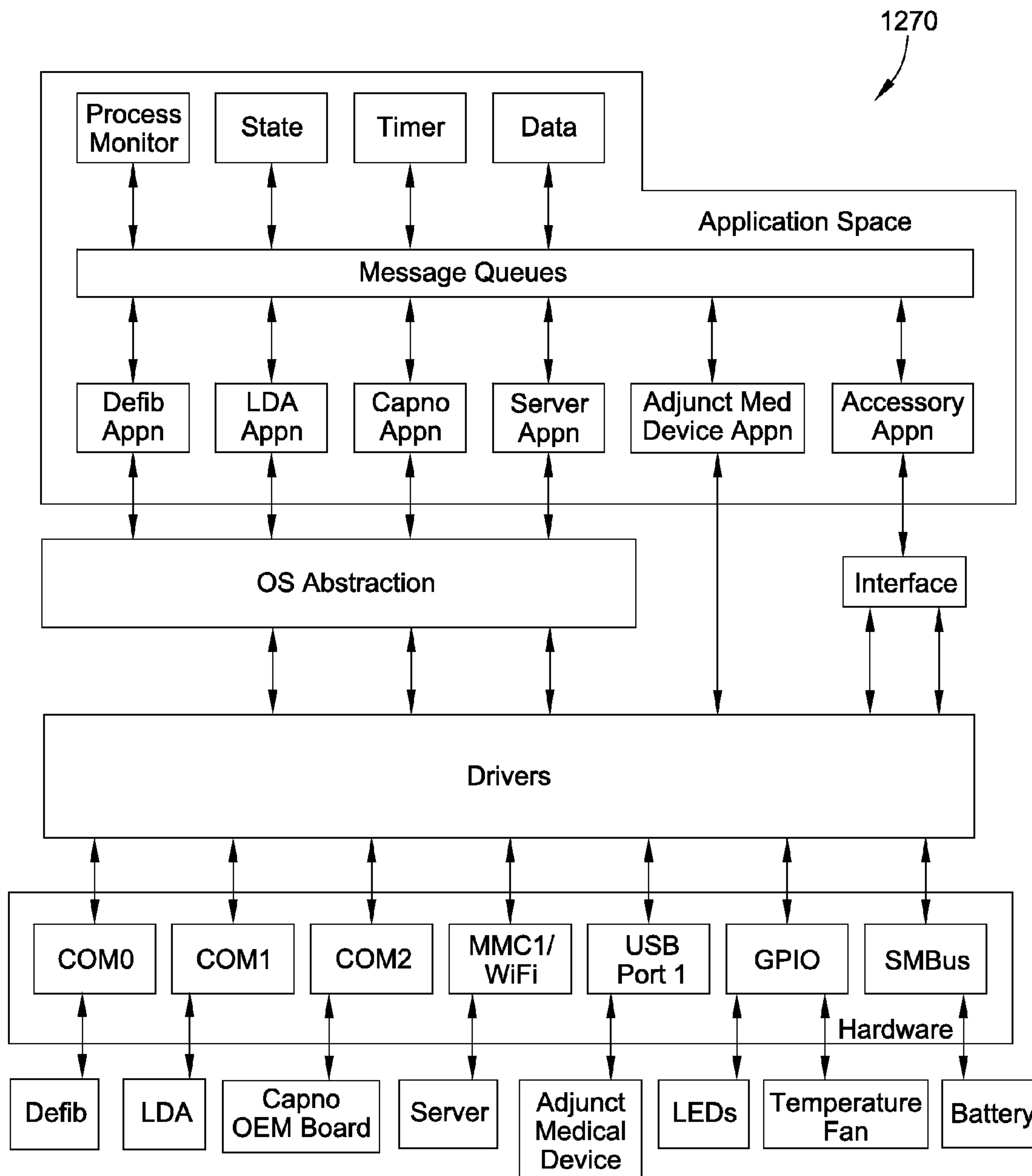
FIG. 24
