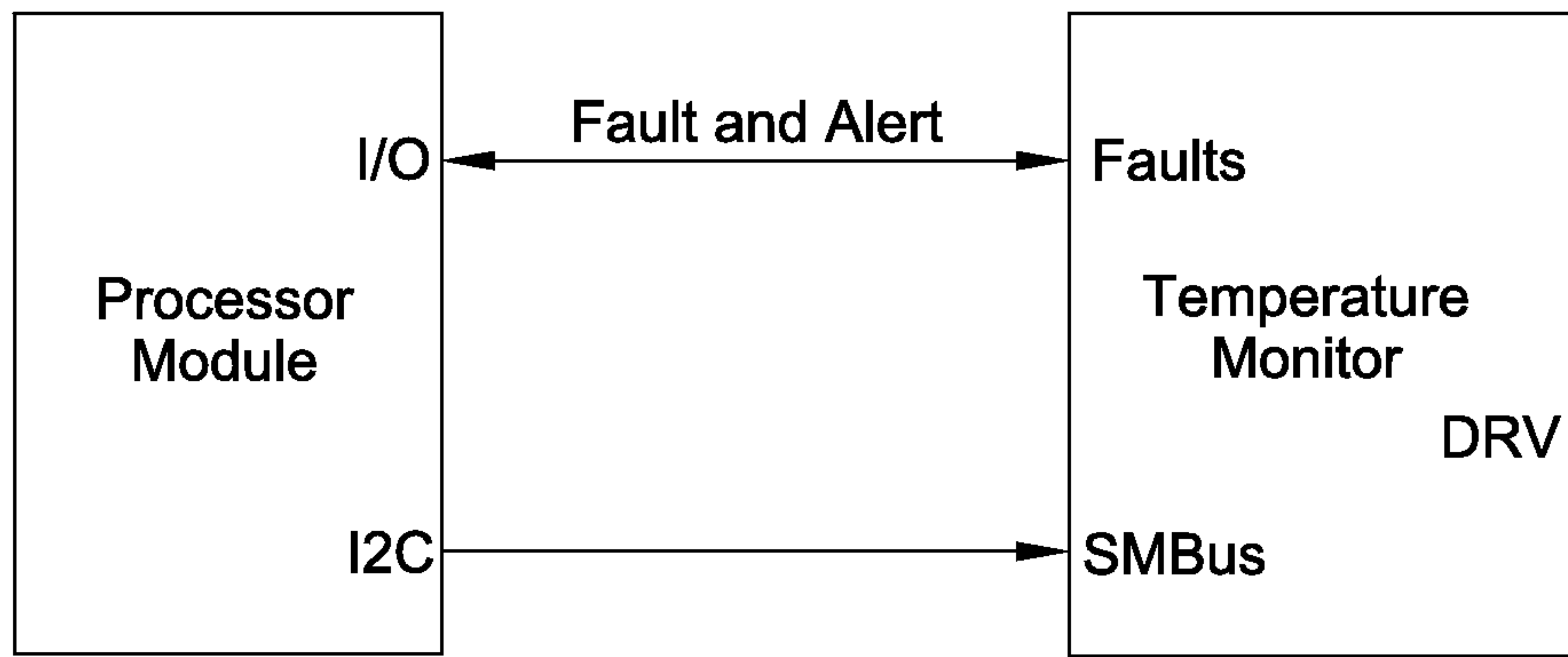
FIG. 8
