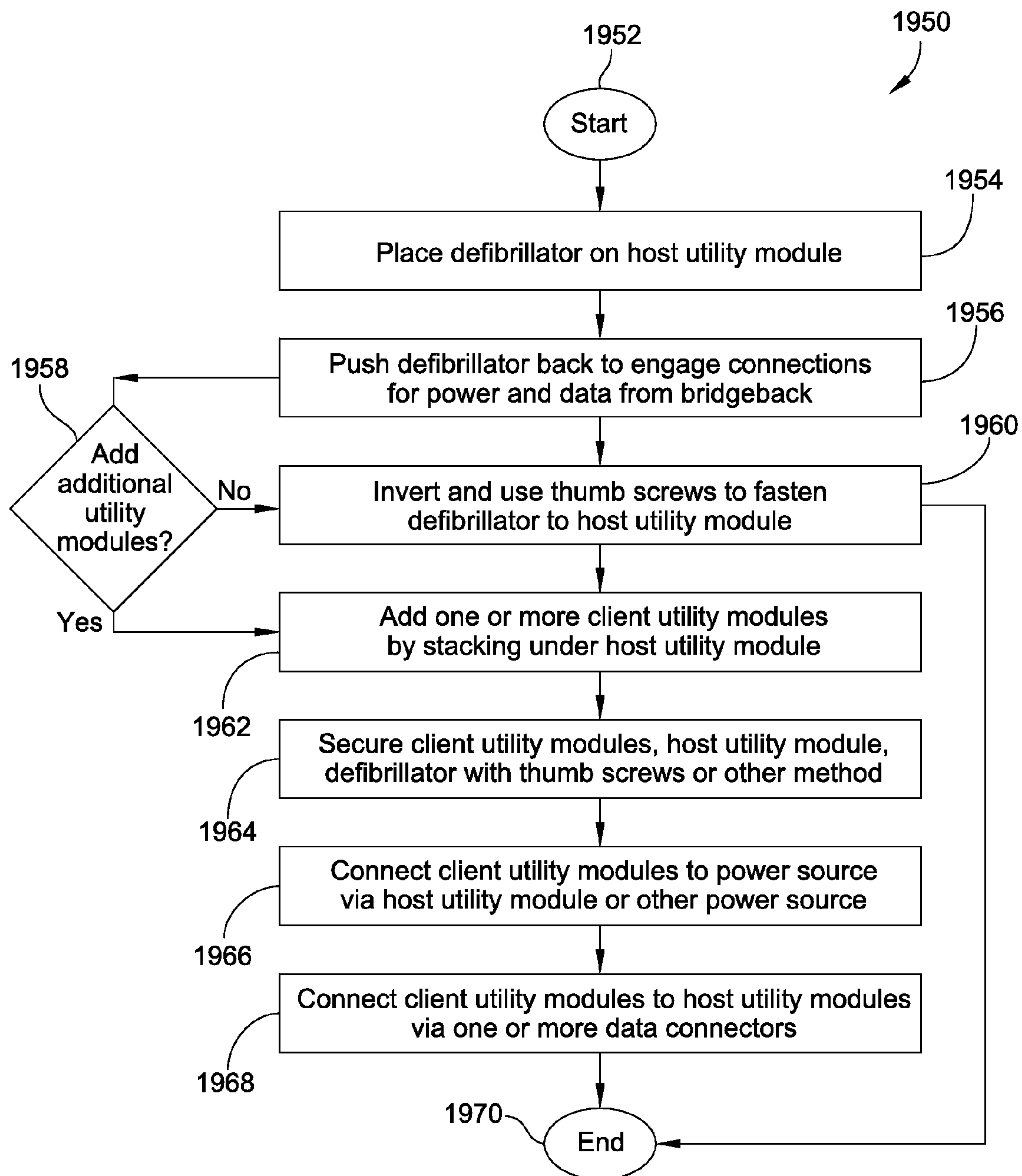
FIG. 35
