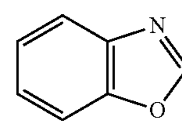
1,3-benzoxazole
