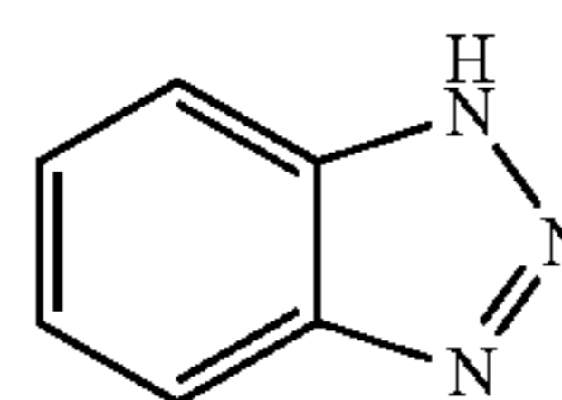
1H-benzotriazole
