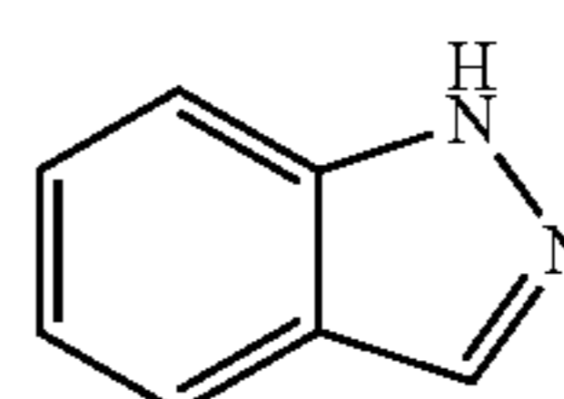
1H-indazole
