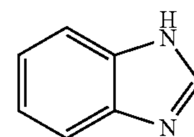
1H-benzimidazole
