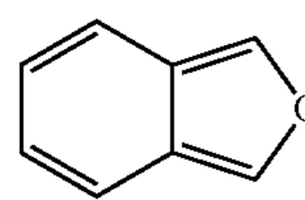
2-benzofuran
