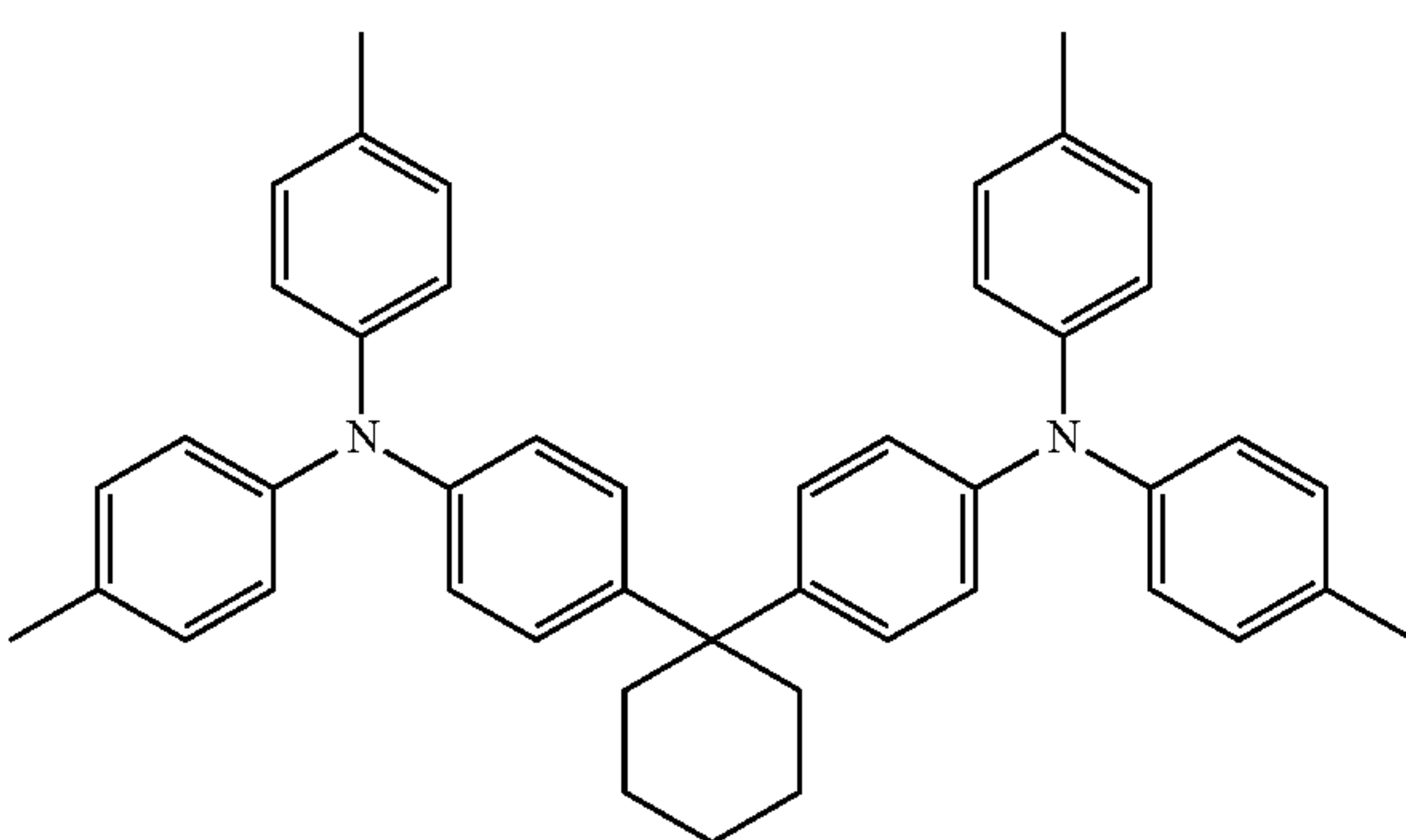
TAPC
