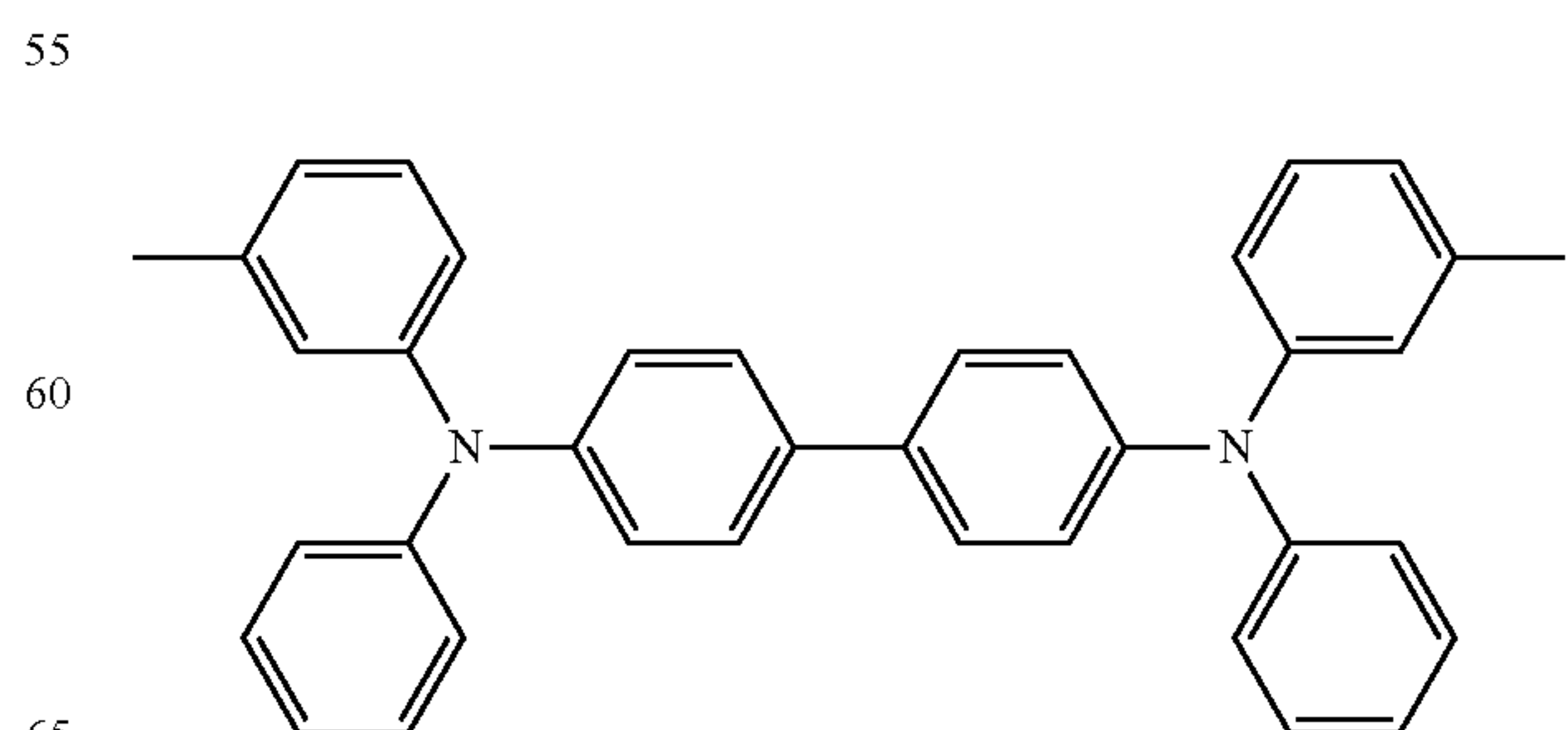
TPD
