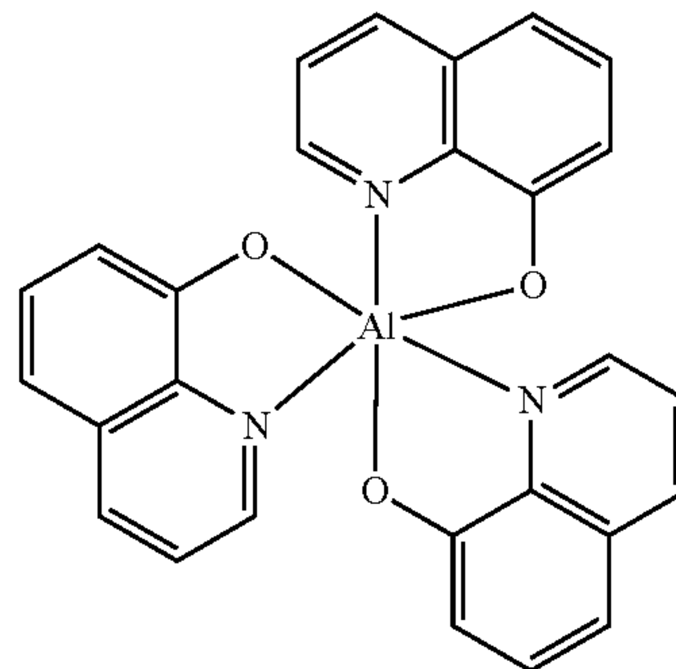
Alq 3
