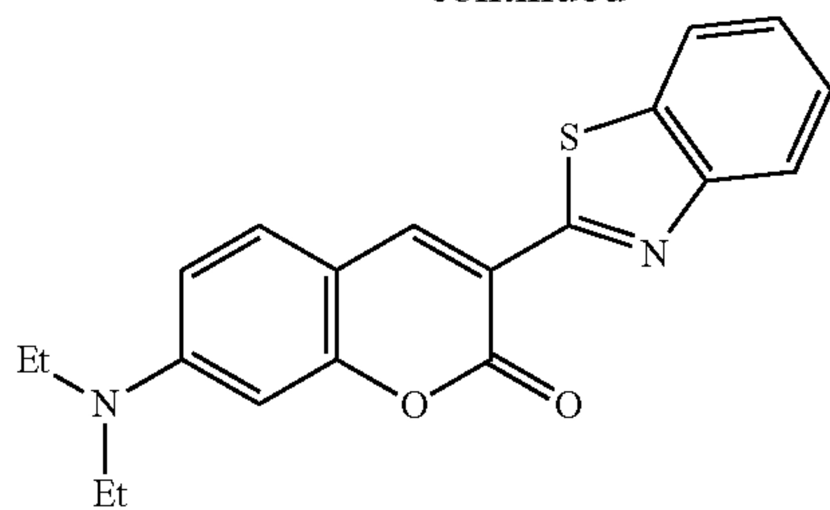
Coumarin 6
