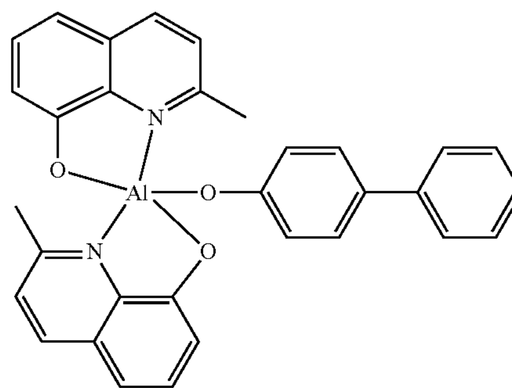
BALq
