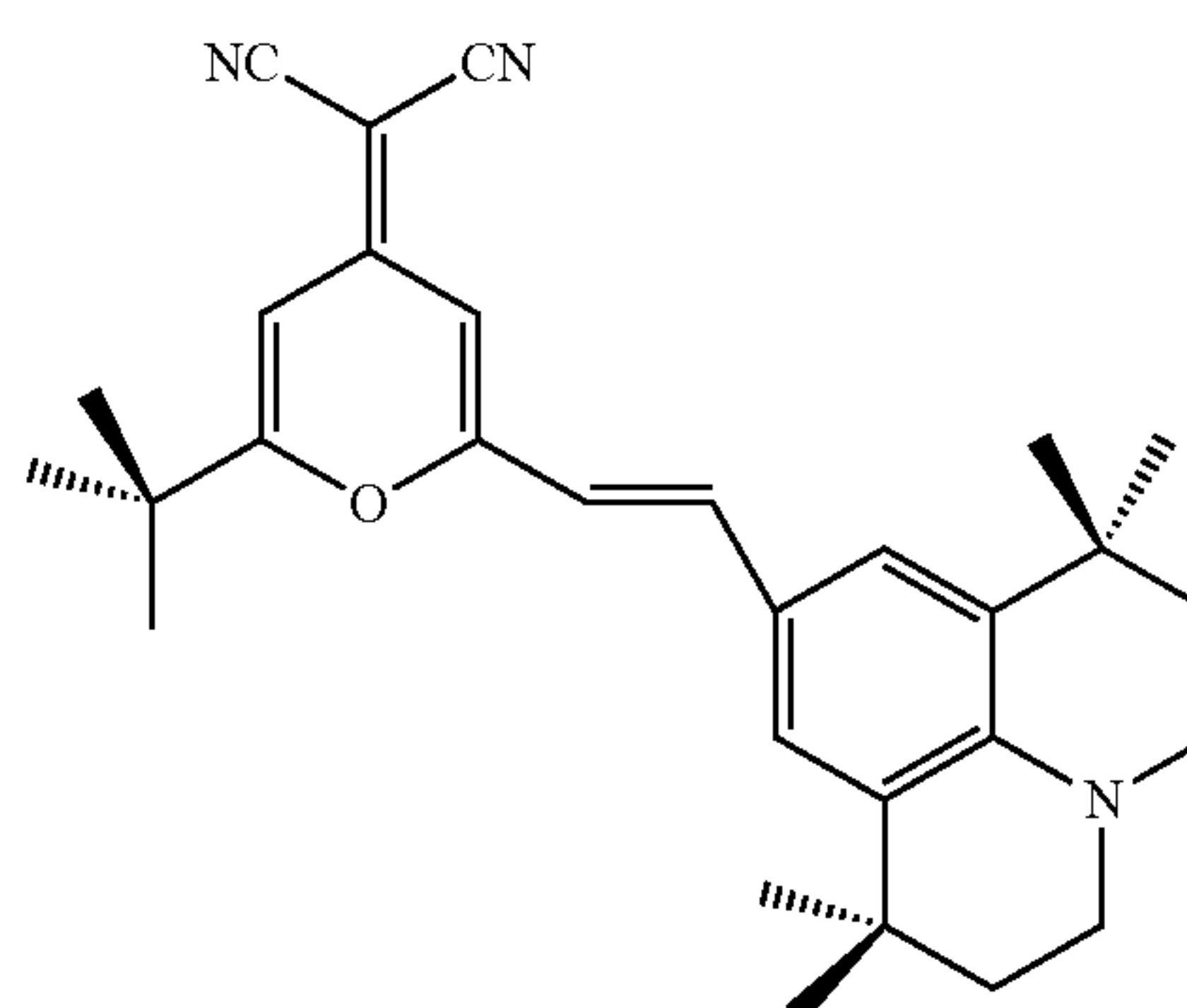
DCJTb
