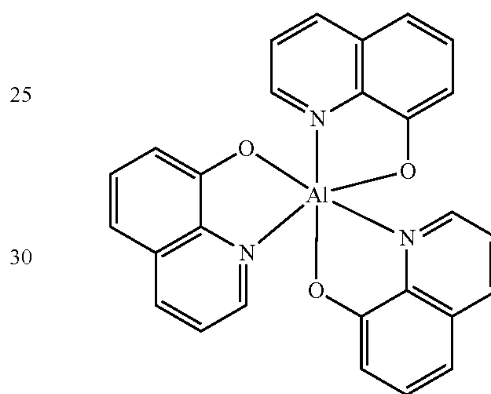
Alq 3
