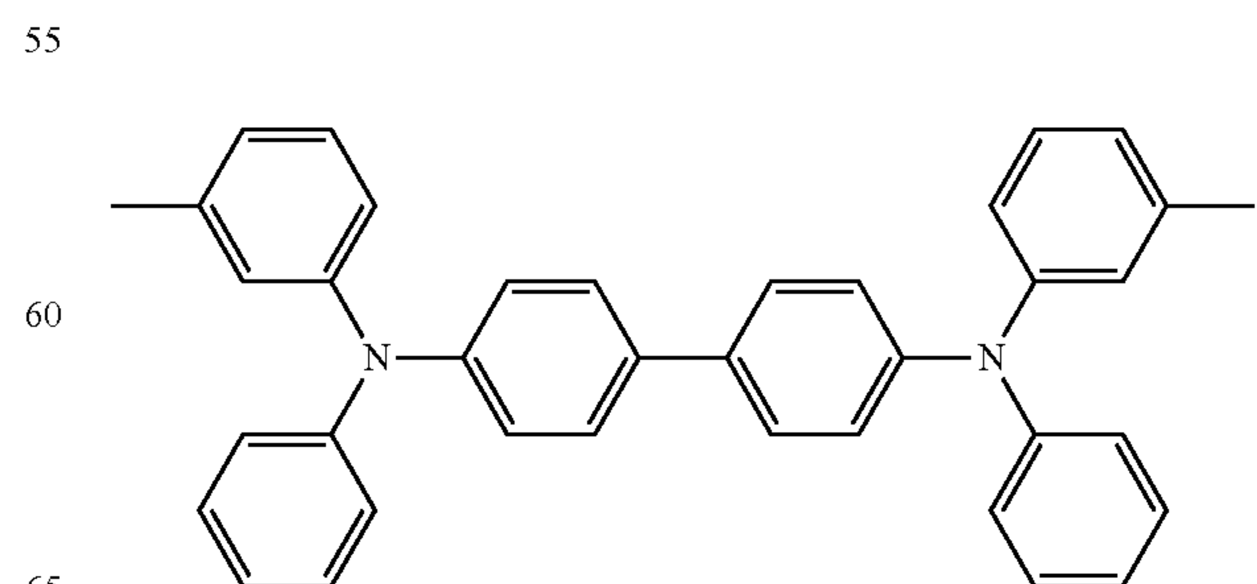
TPD
