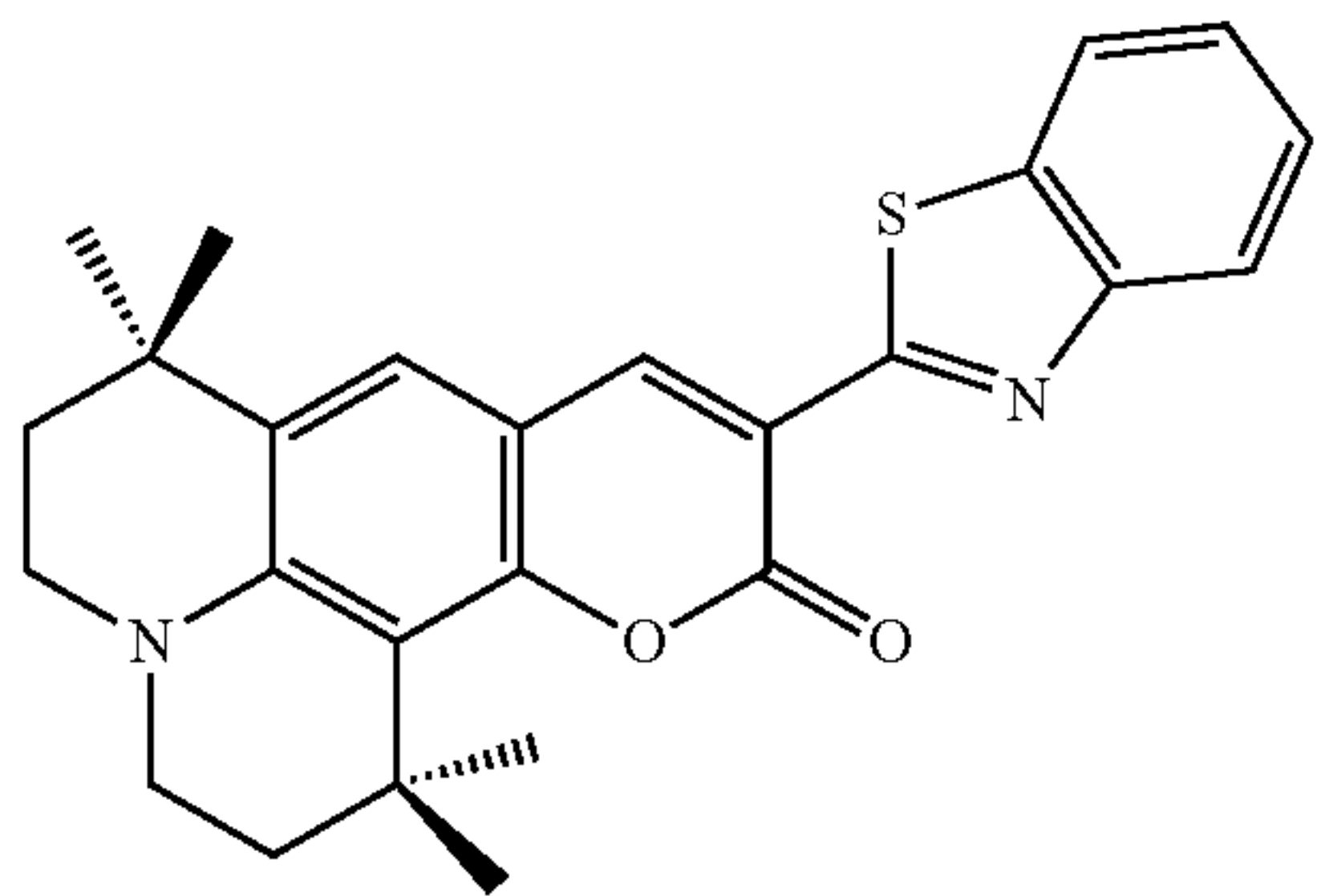
Coumarin 6
