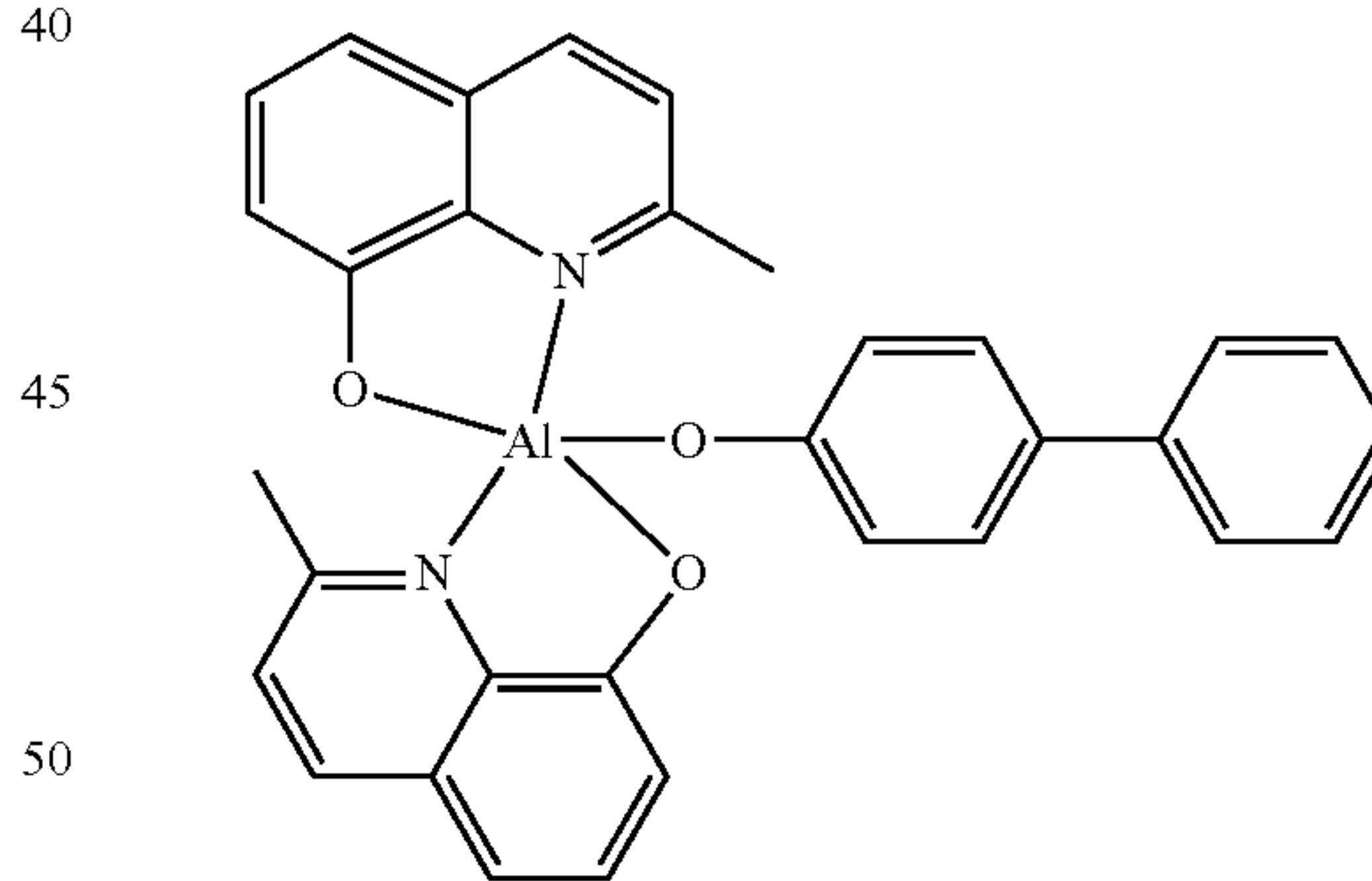
BALq
