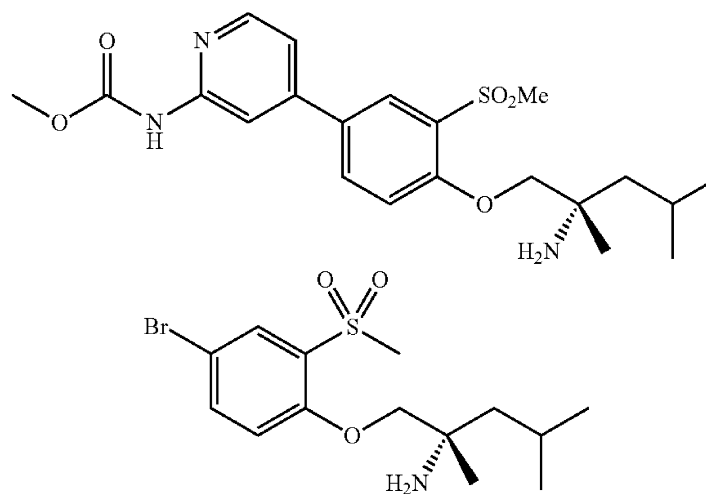
Part A: (S)-1-(4-bromo-2-(methylsulfonyl)phenoxy)-2,4-dimethylpentan-2-amine
