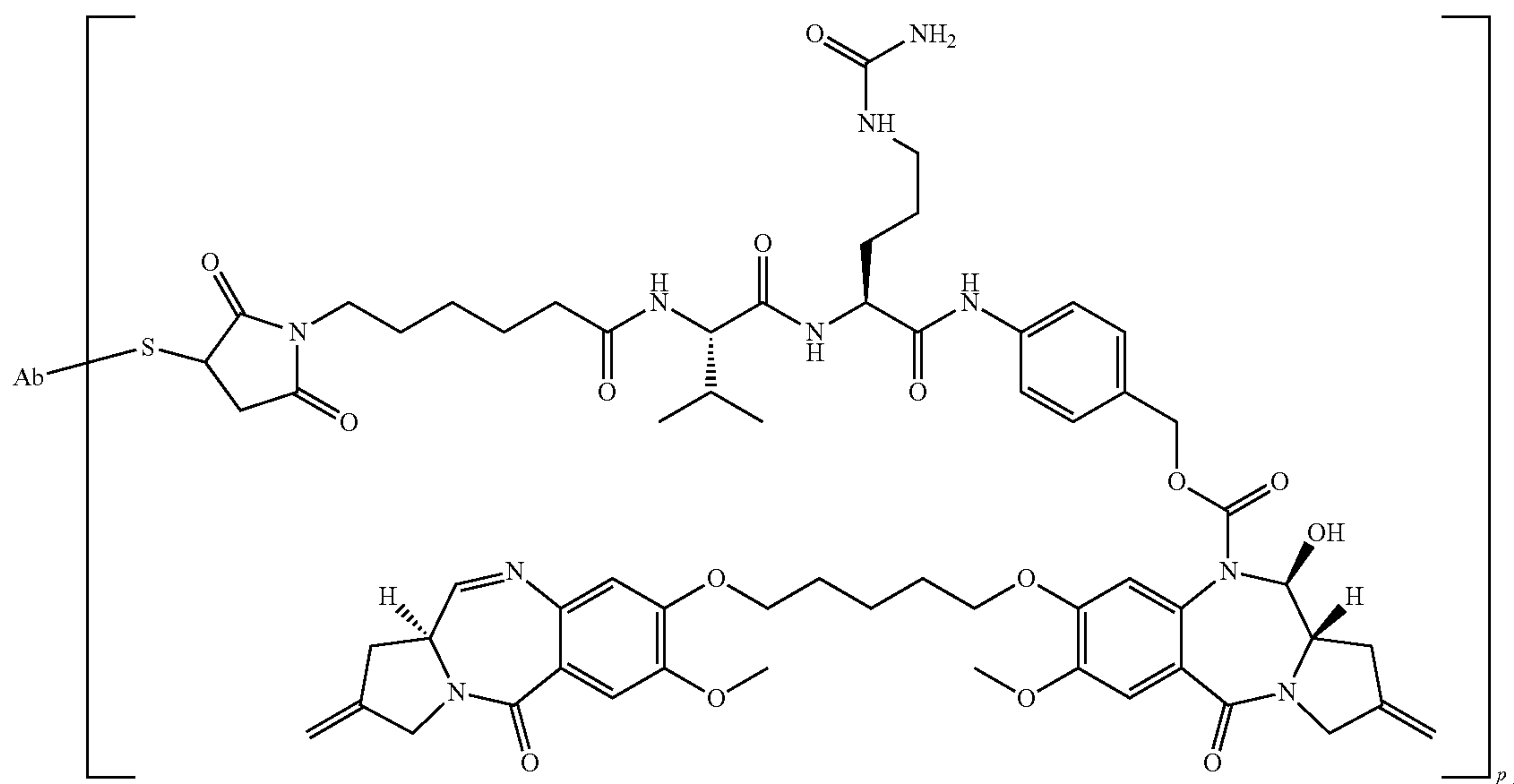
PBD dimer-val-cit-PAB-Ab
