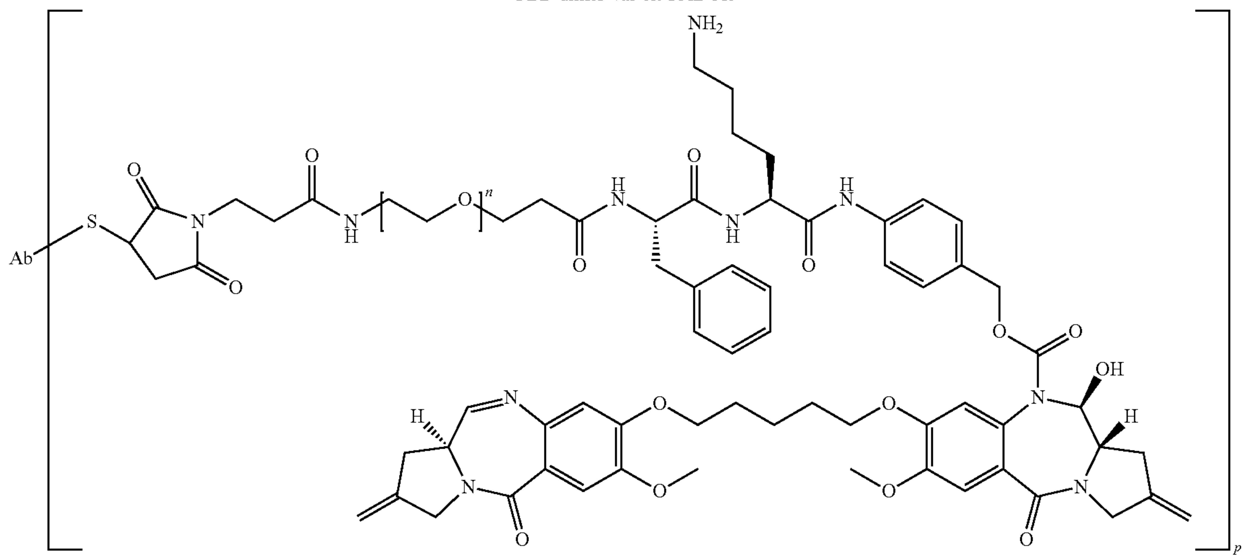
PBD dimer-Phe-Lys-PAB-Ab
