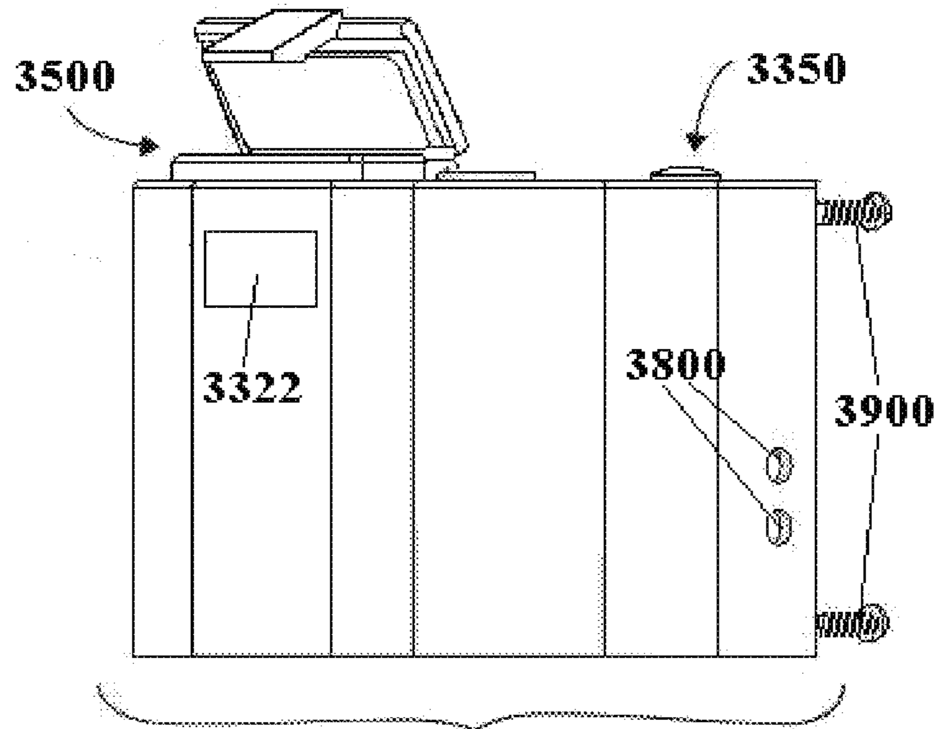
FIG. 13(D)
