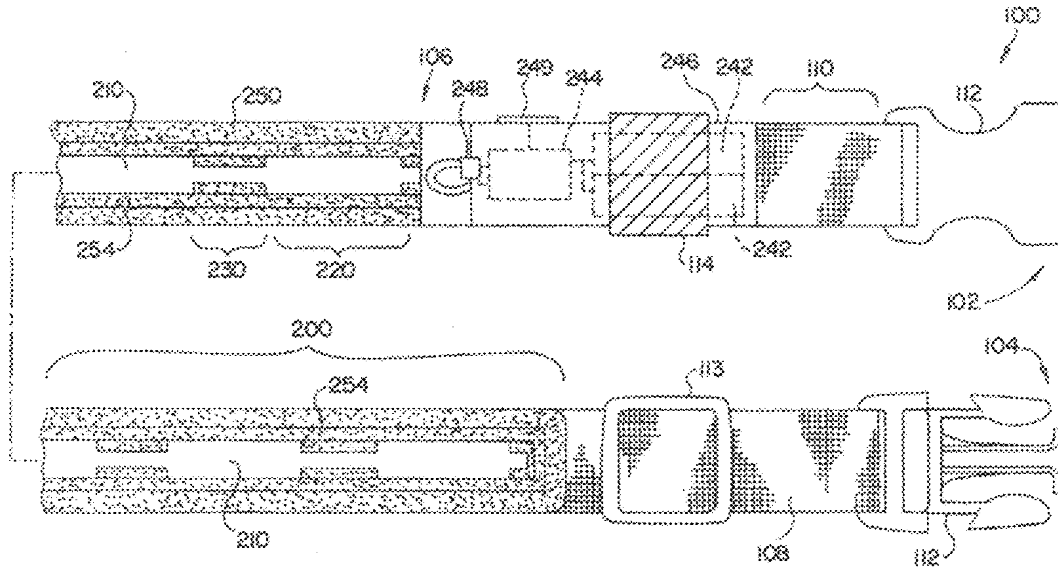
FIG. 1A
