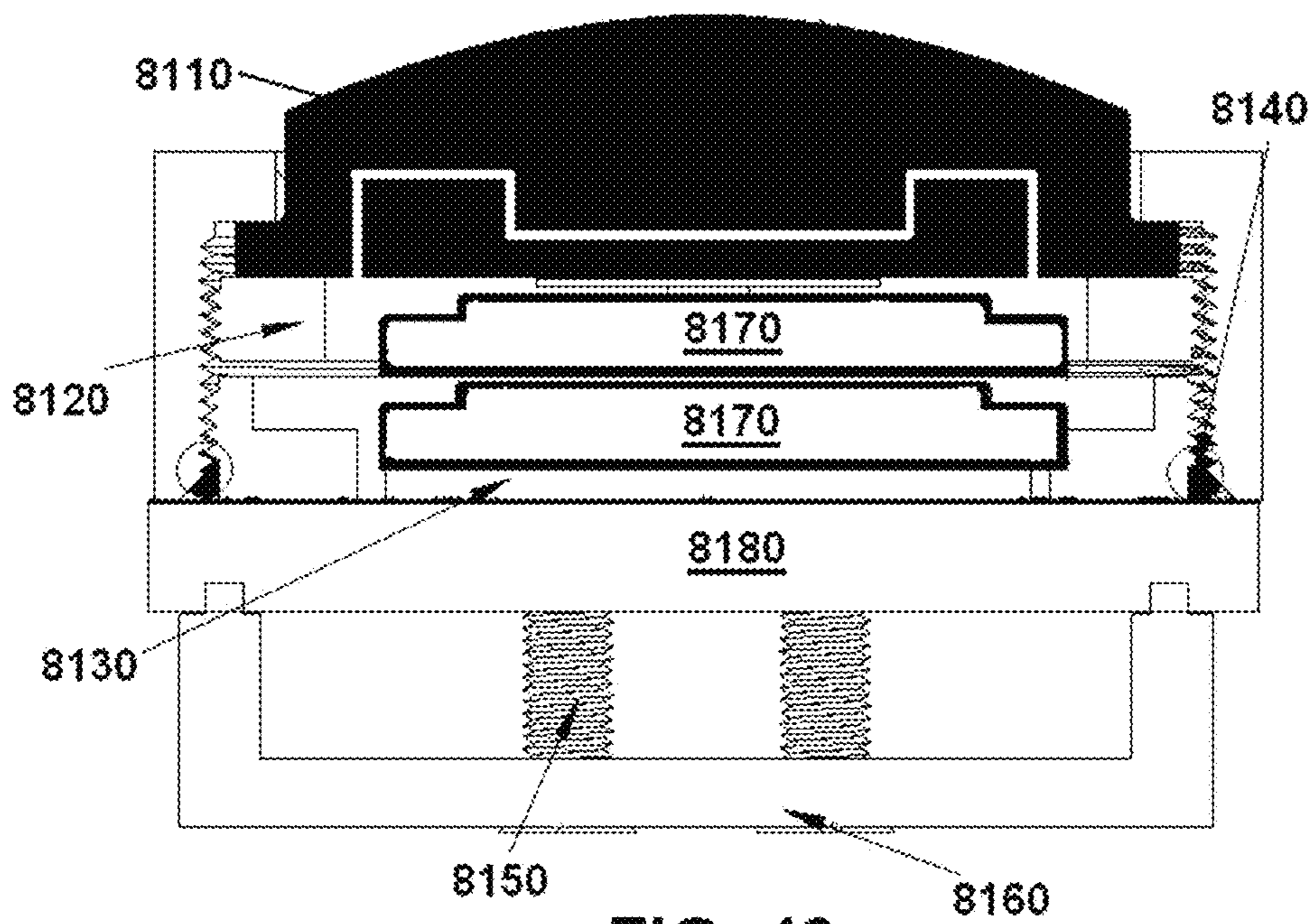
FIG. 40
