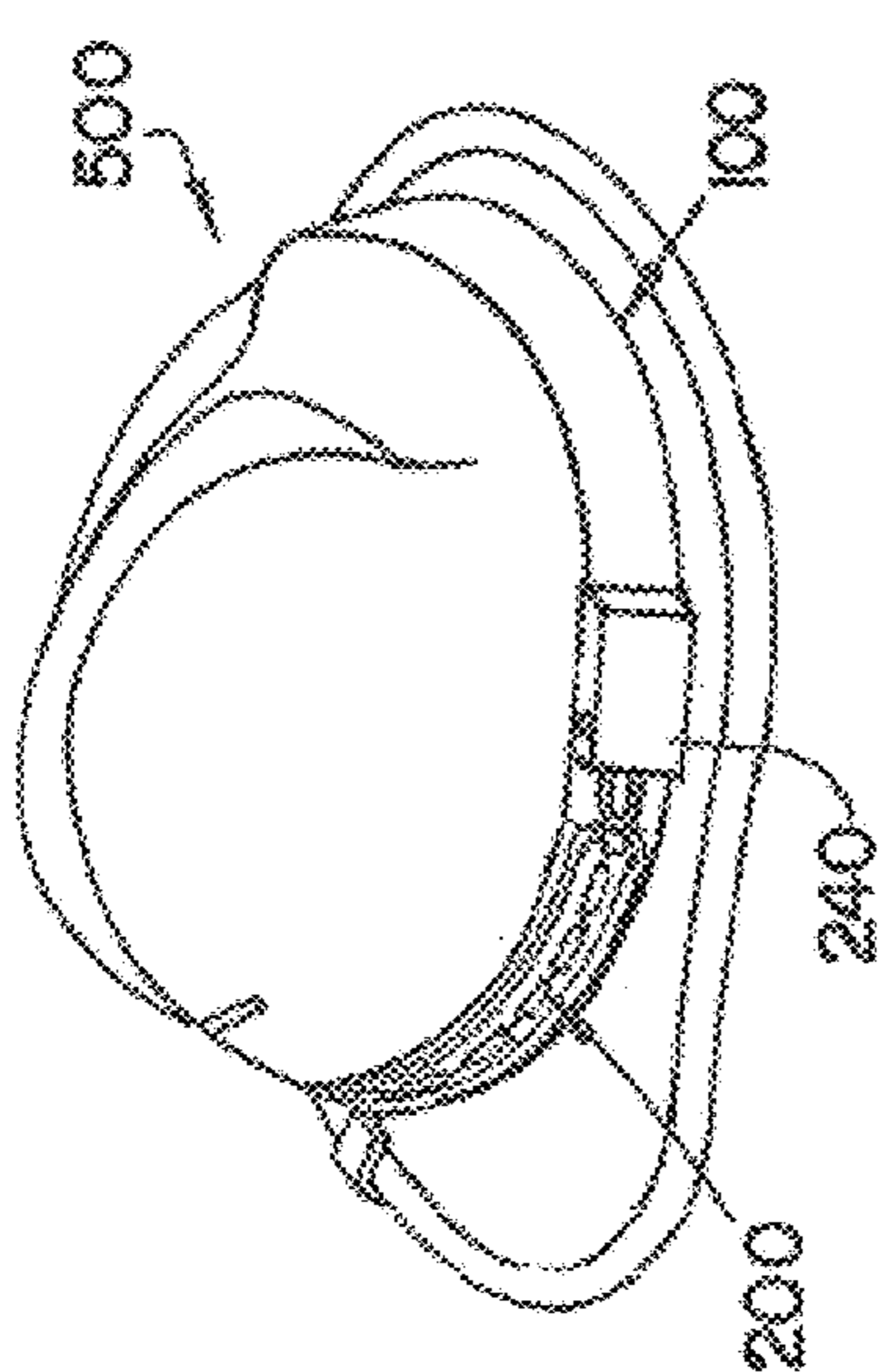
FIG. 8C
