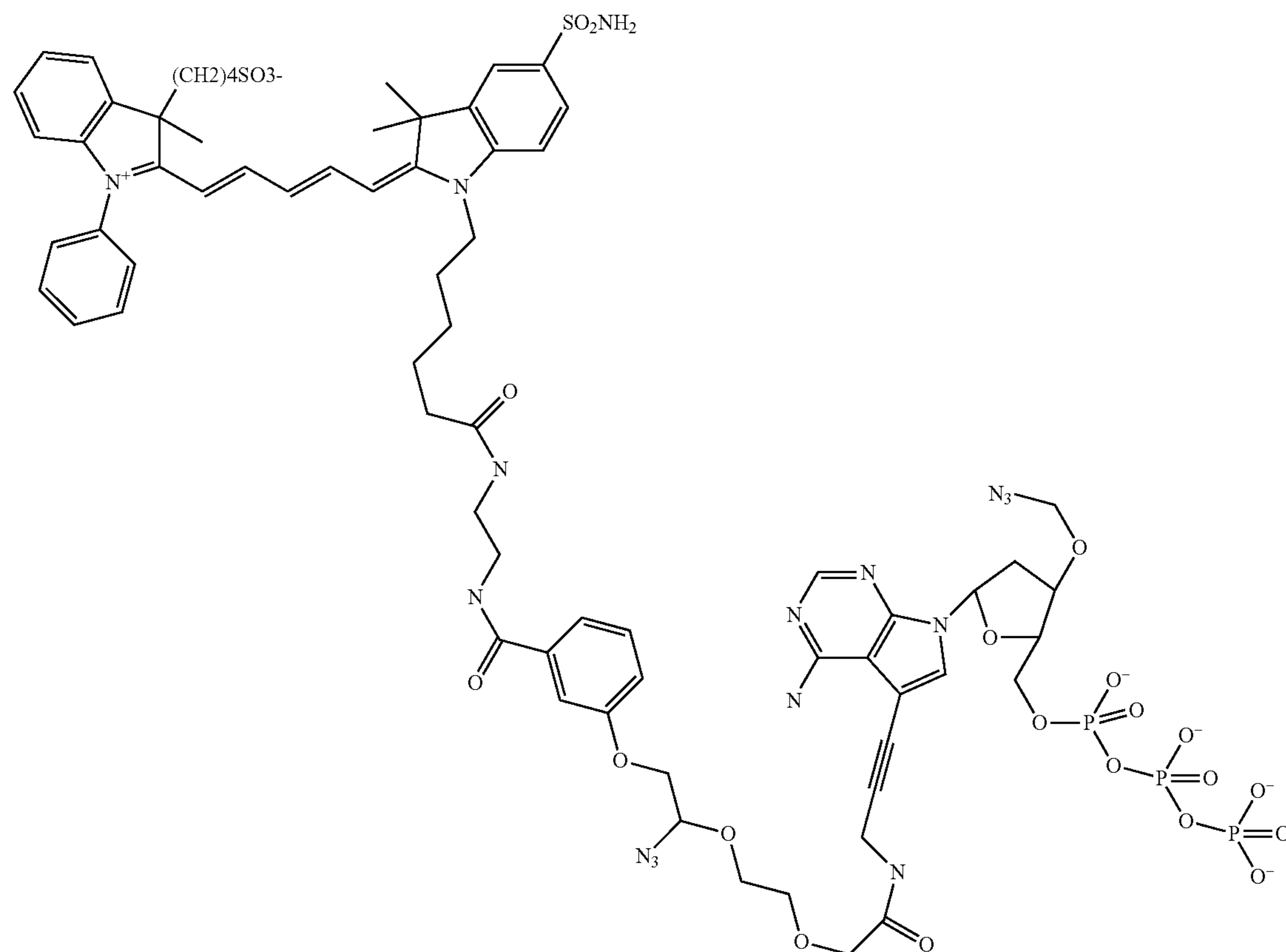
ff-dATP-D7
