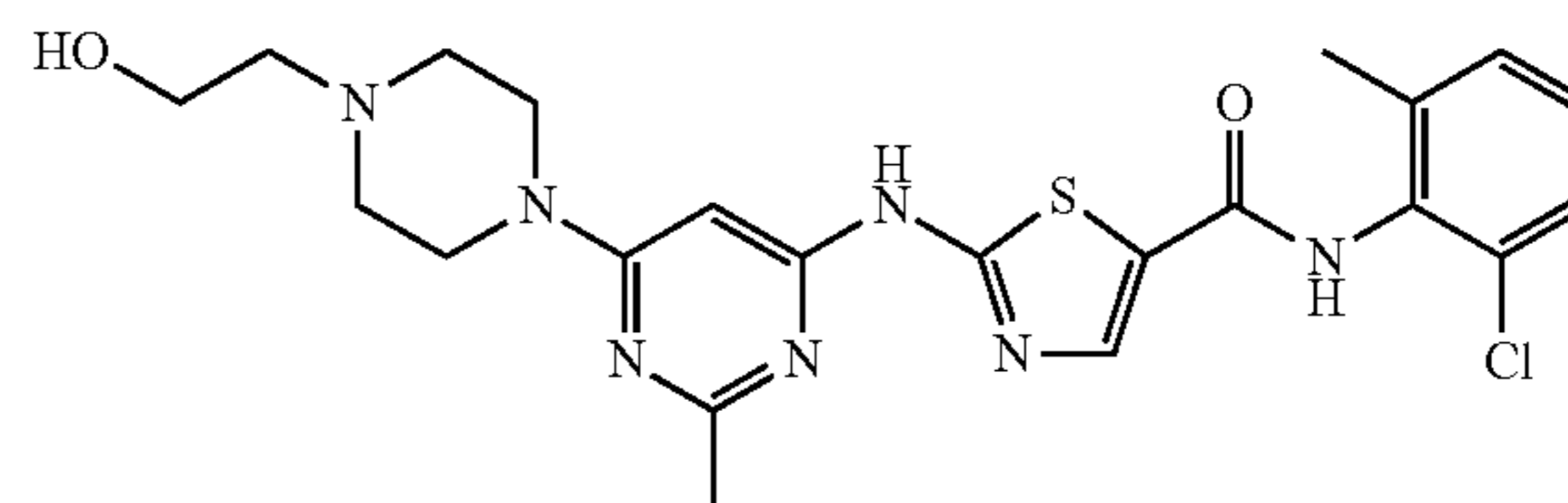
Dasatinib
