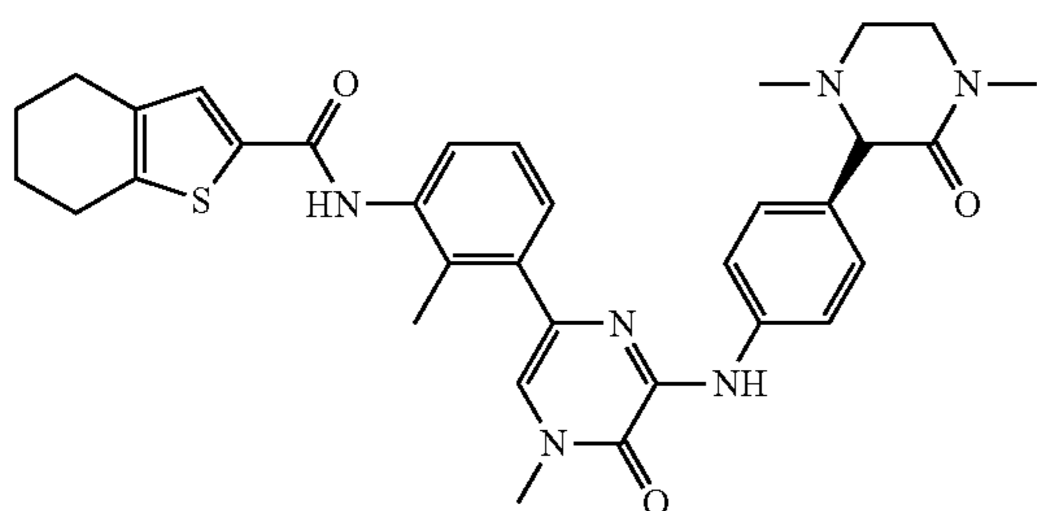
GDC-0834
