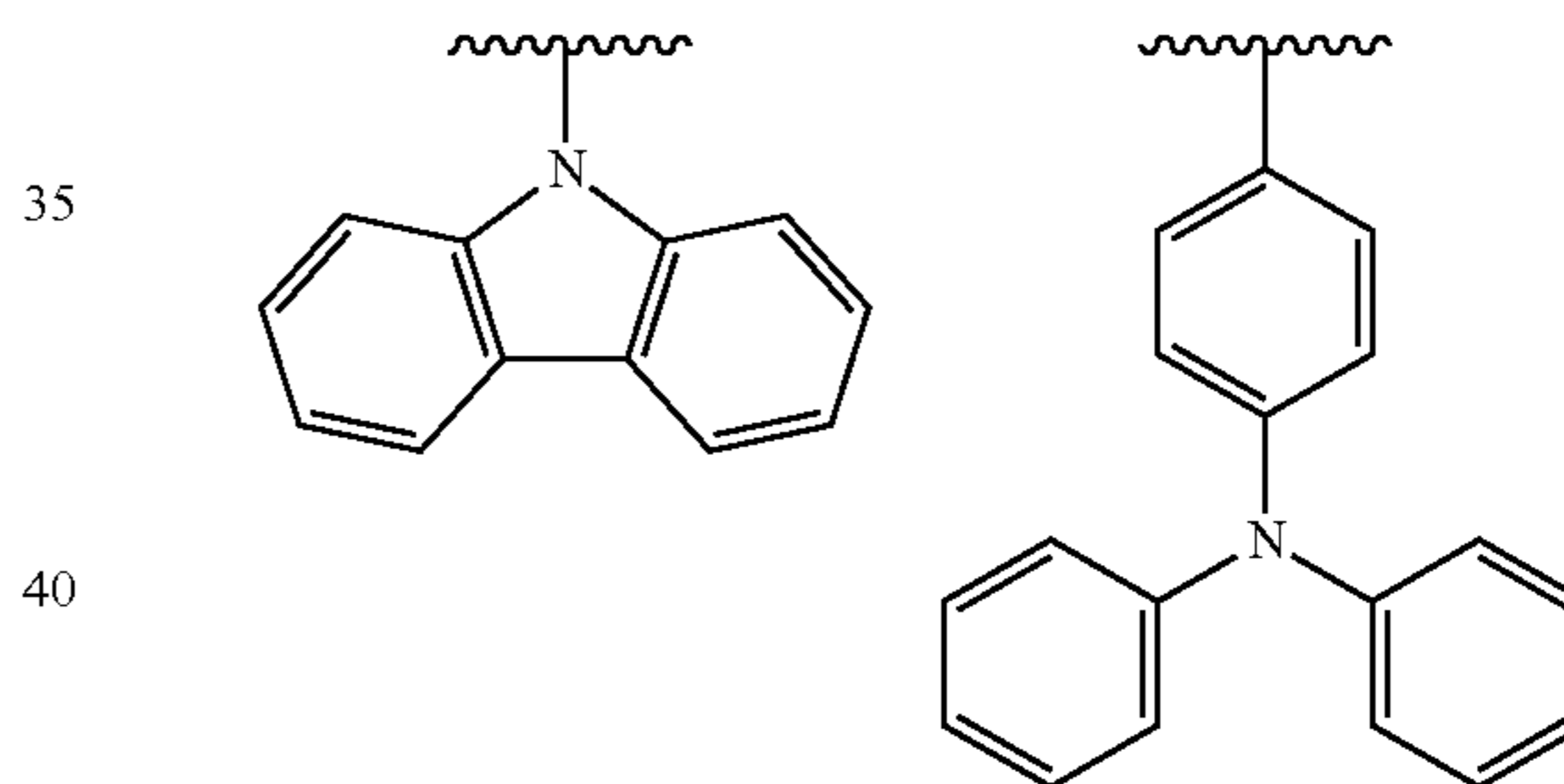
[Formula 3]
