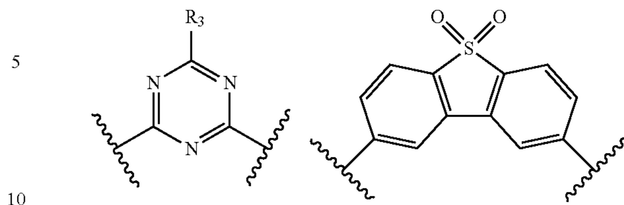
[Formula 5]
