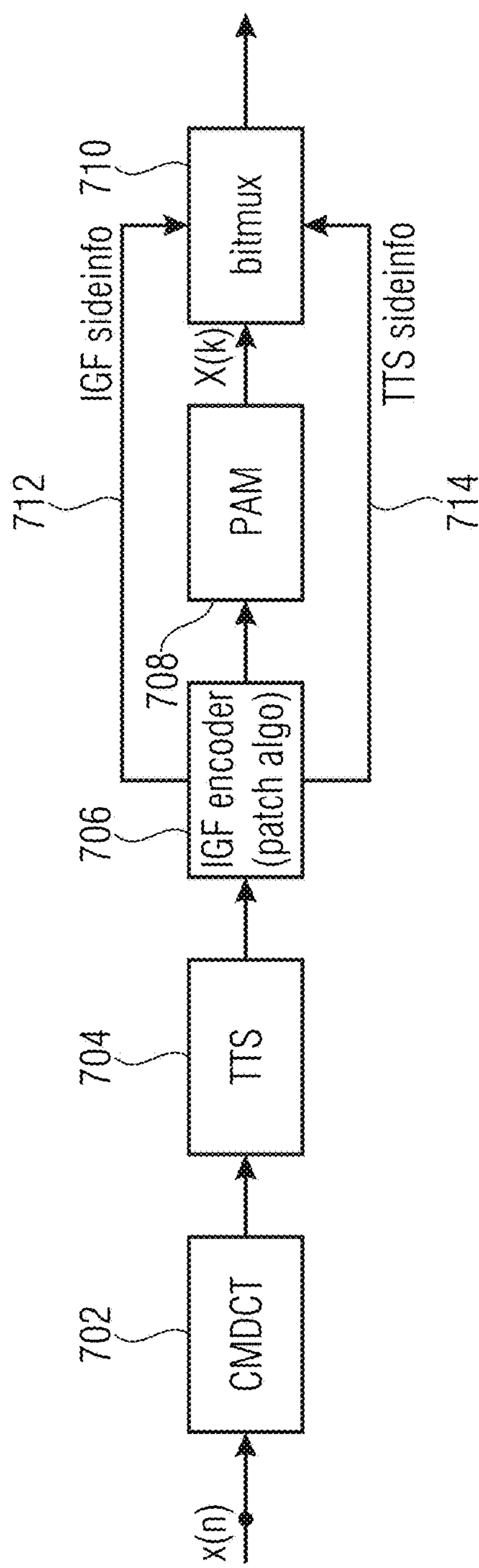
FIG 7A (ENCODER)
