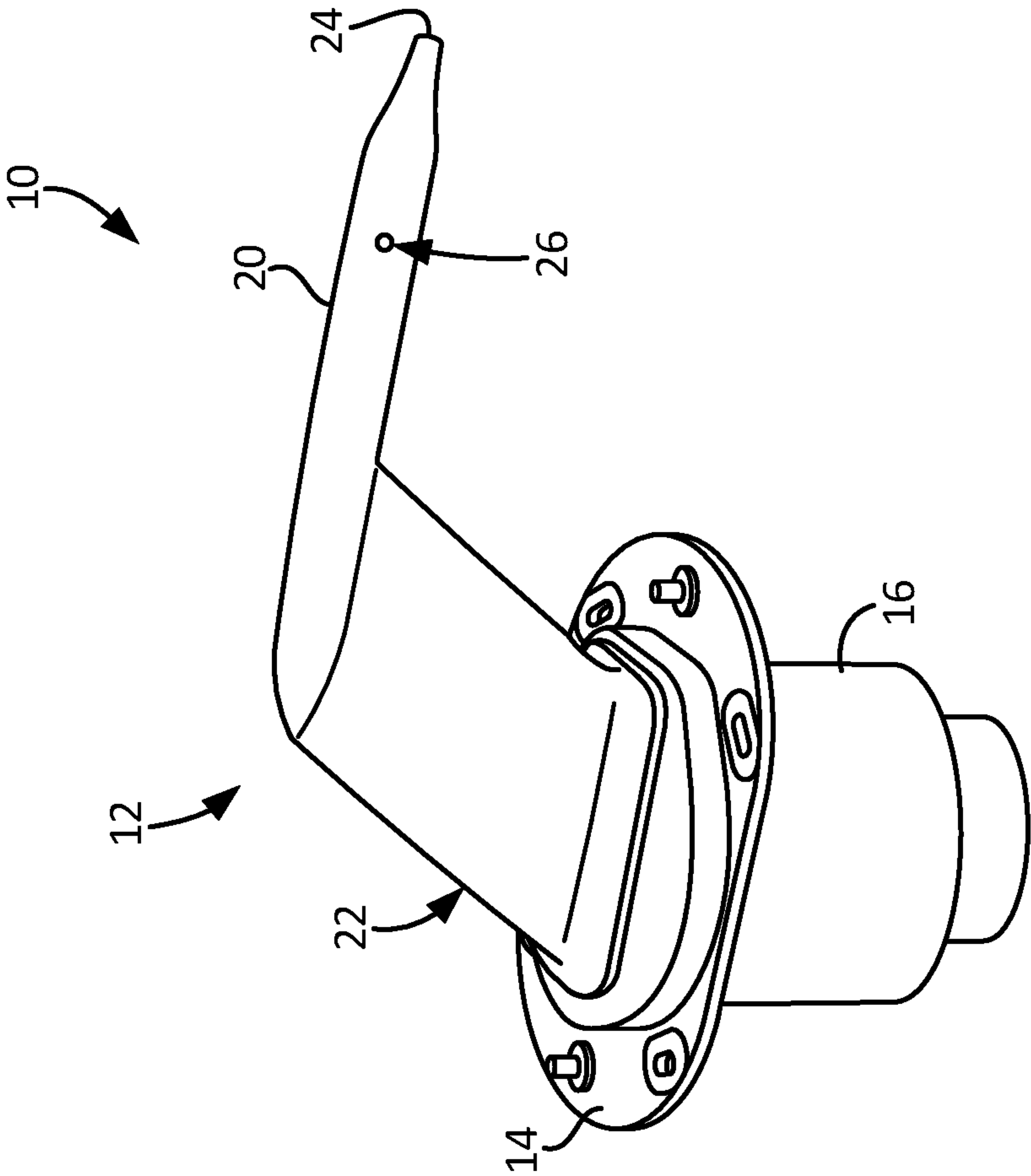
Fig. 1A
