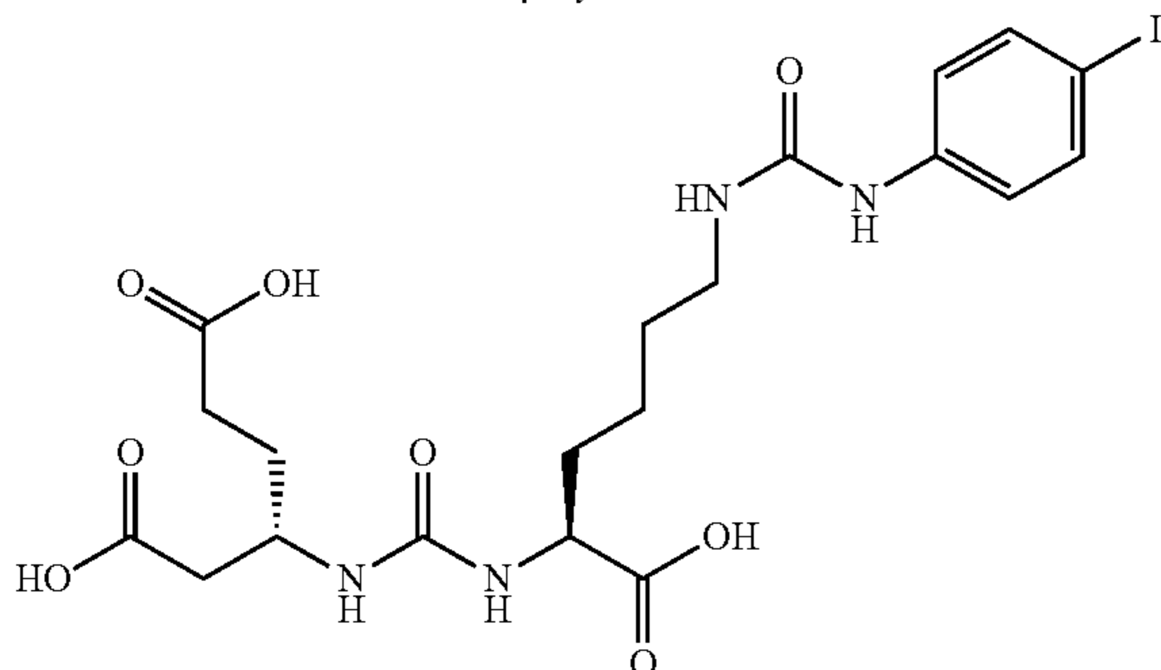
\beta -glu
