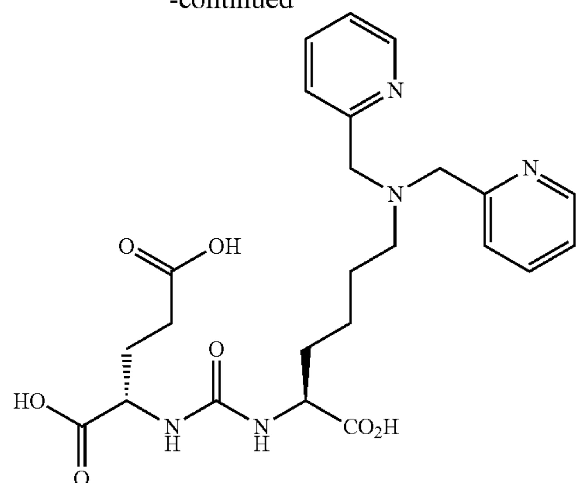
L-(S)-2-[(Imidazole-1-carbonyl)-amino]-pentanedioic acid di-tert-butyl ester (2)
