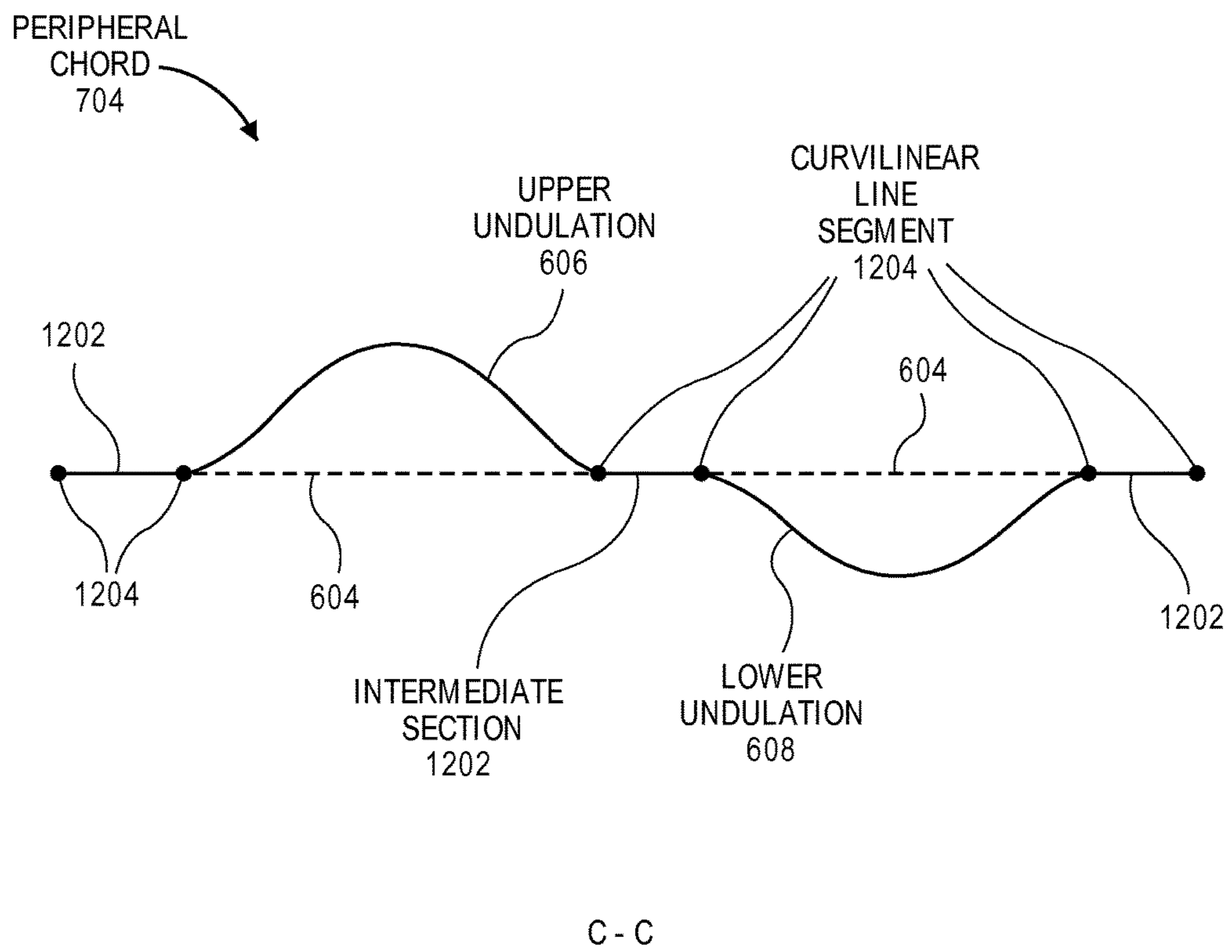
C - C FIG. 13
