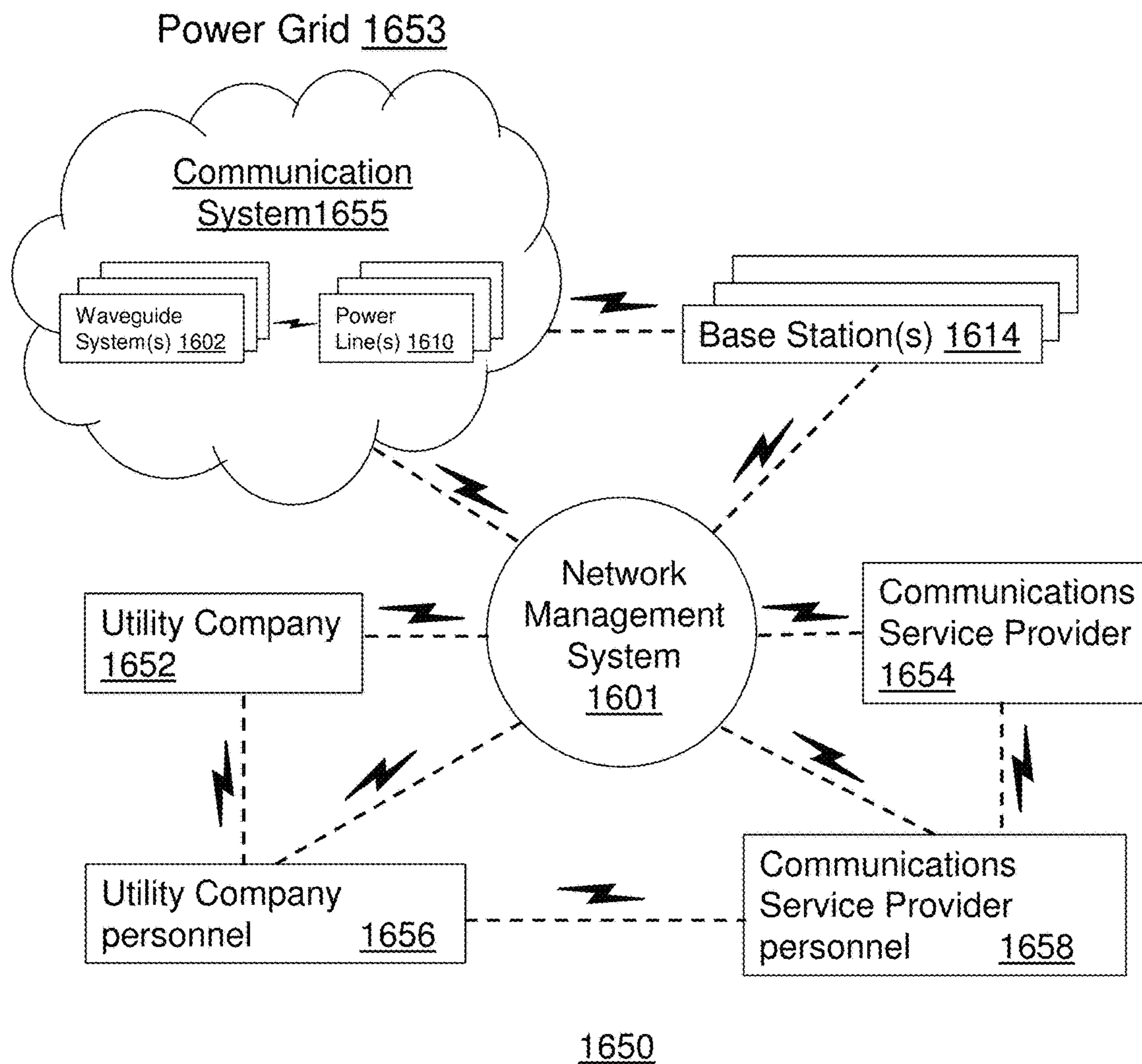
1650 FIG. 16B
