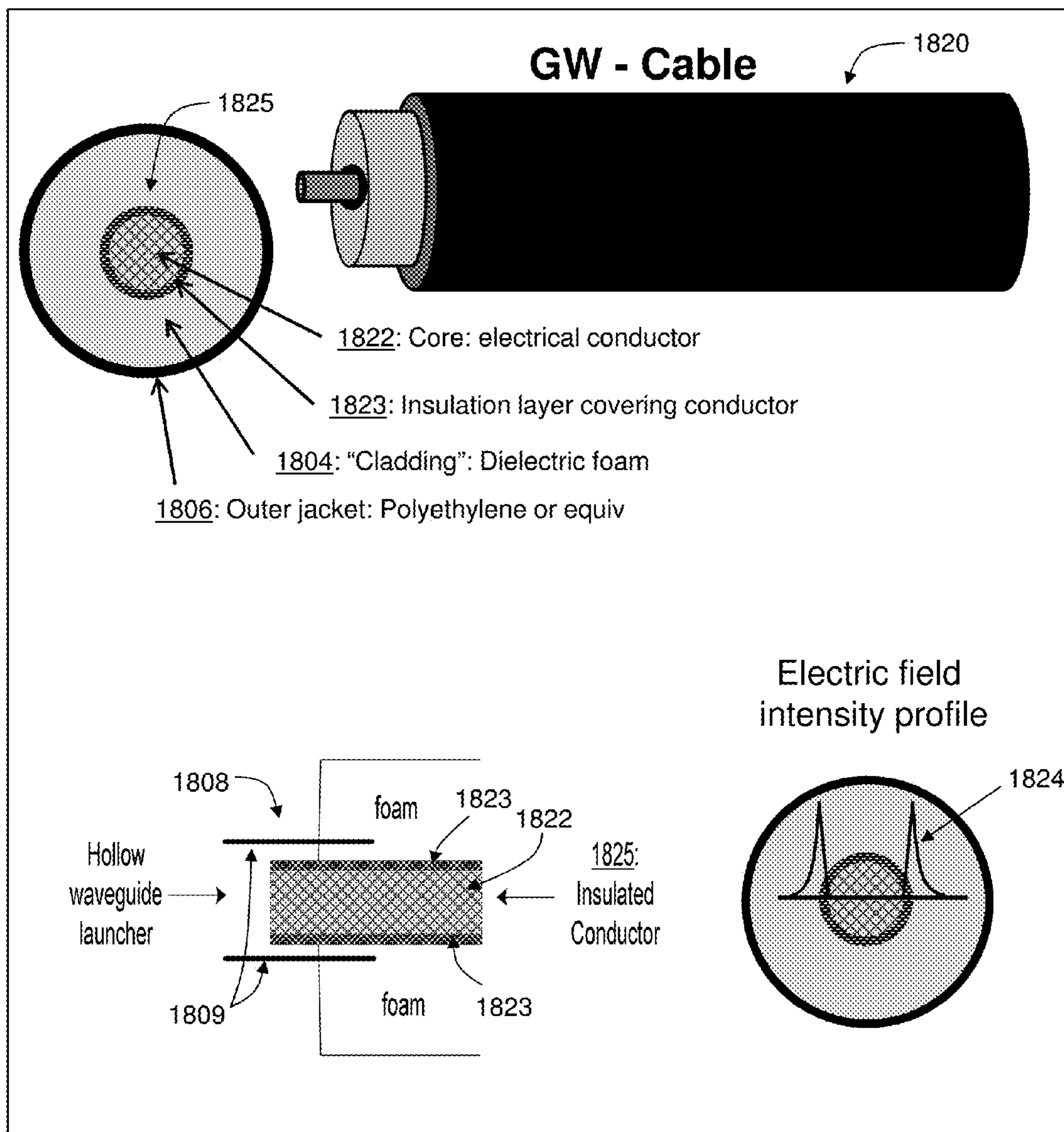
FIG. 18B
