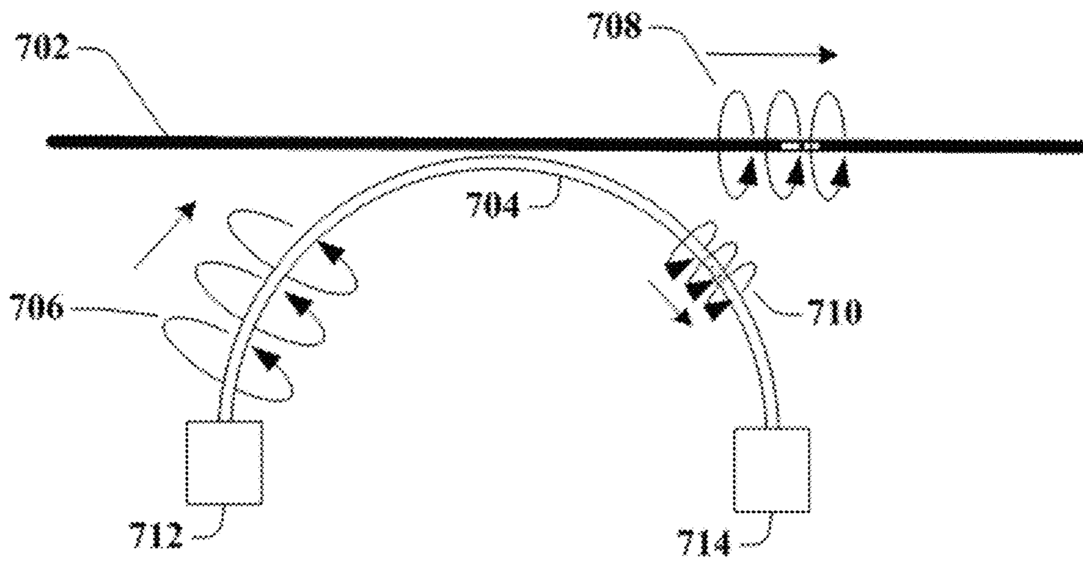
700 FIG. 7
