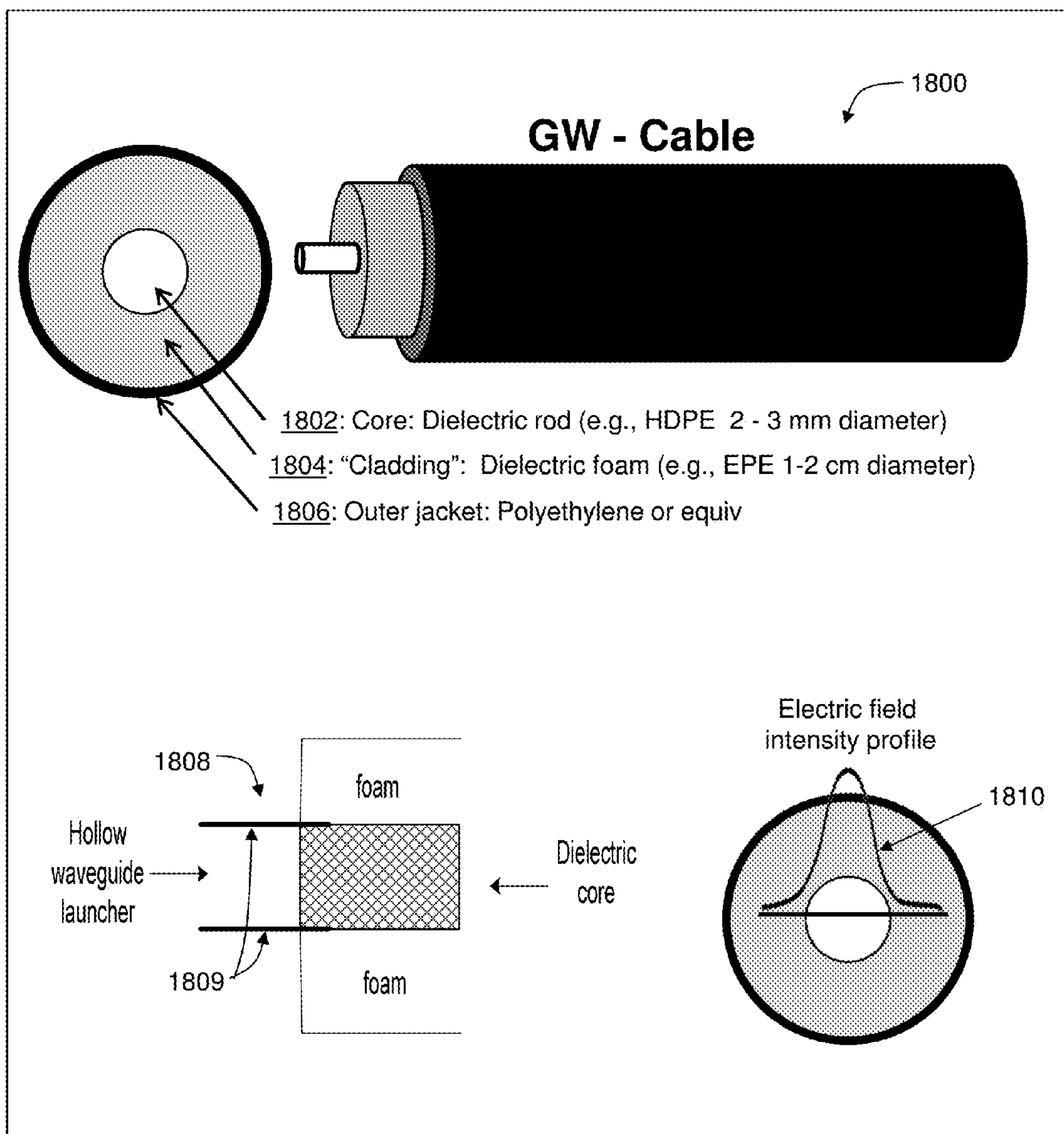
FIG. 18A
