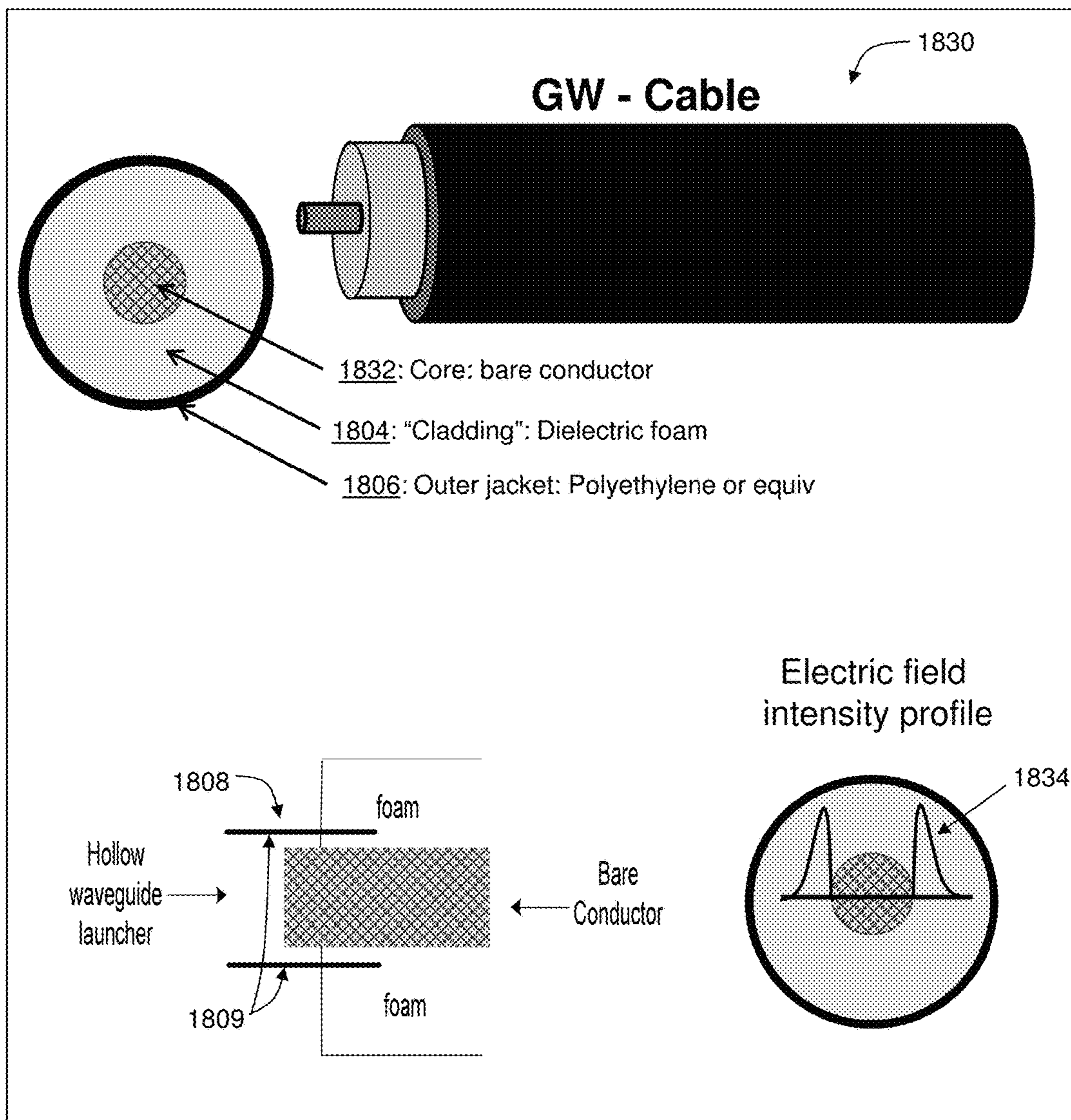
FIG. 18C
