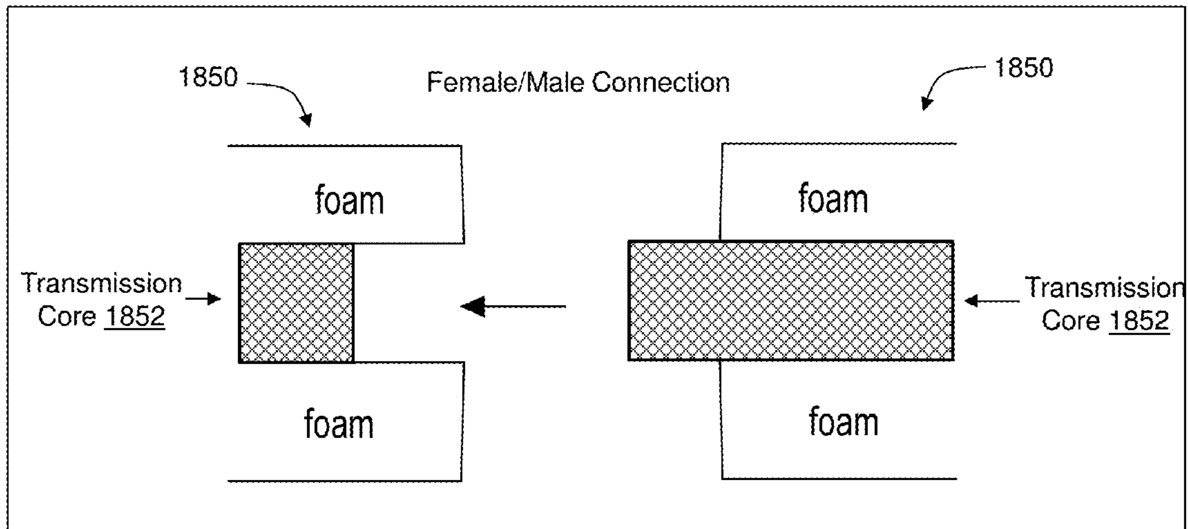
FIG. 18G
