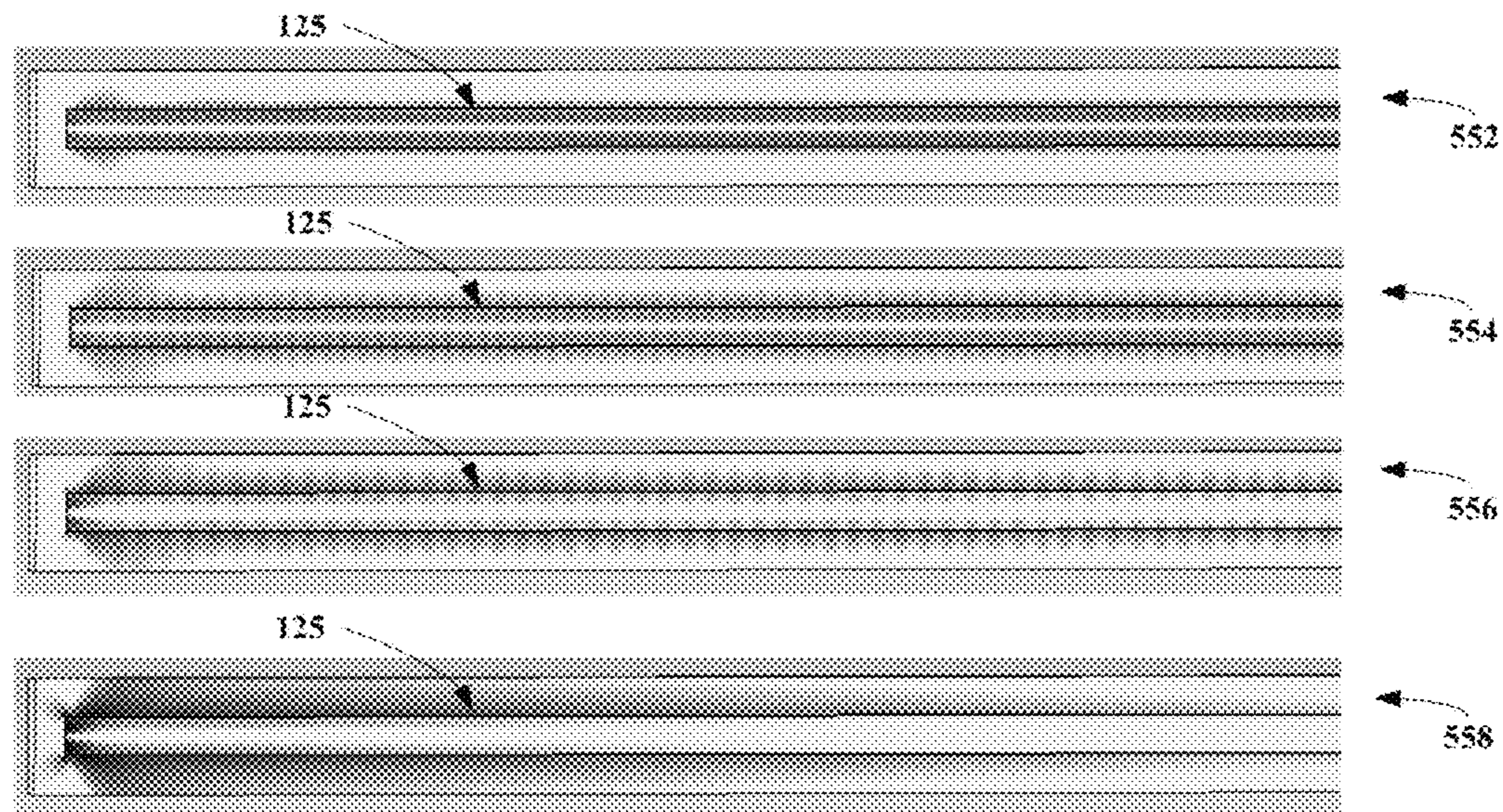
550 FIG. 5B
