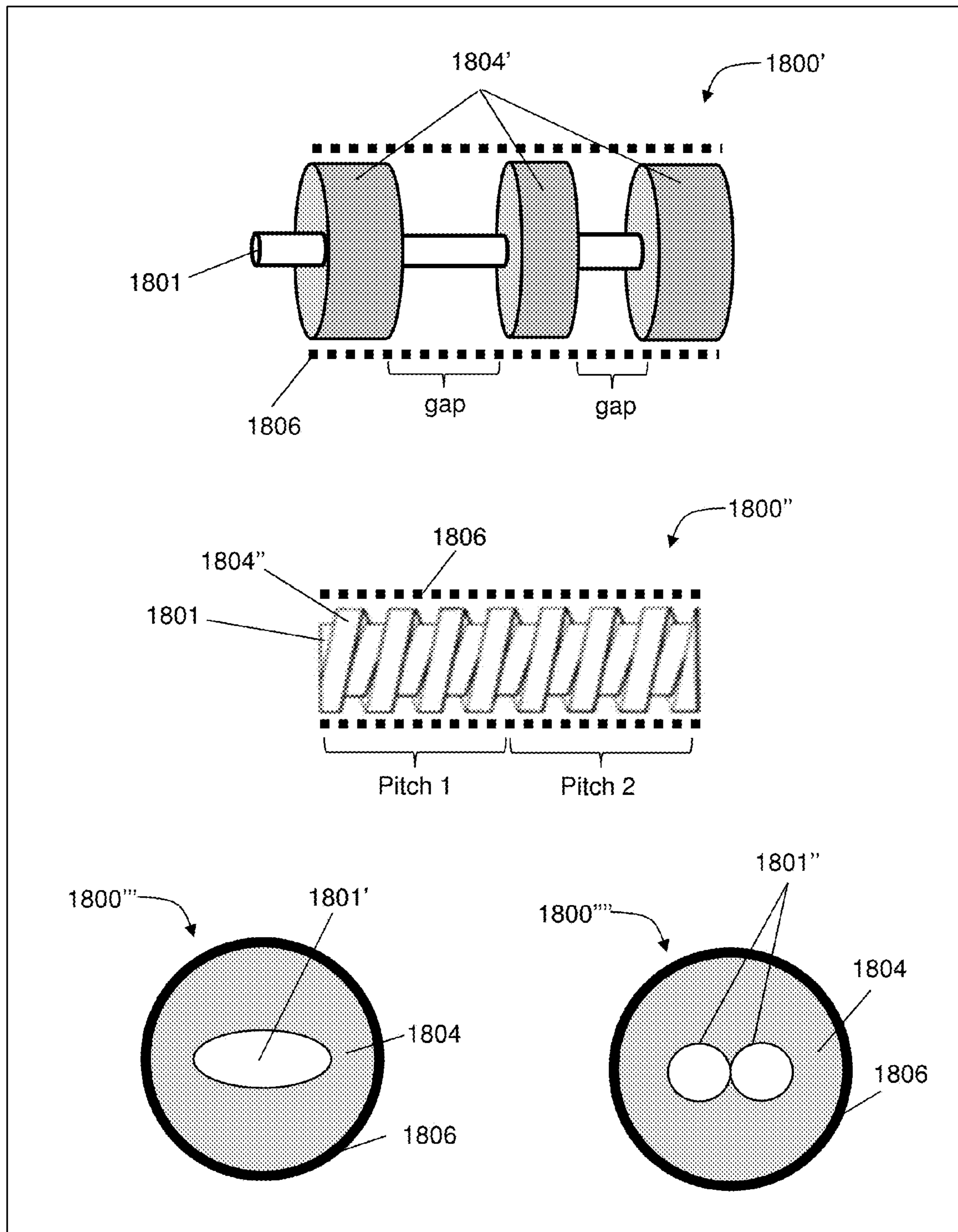
FIG. 18I
