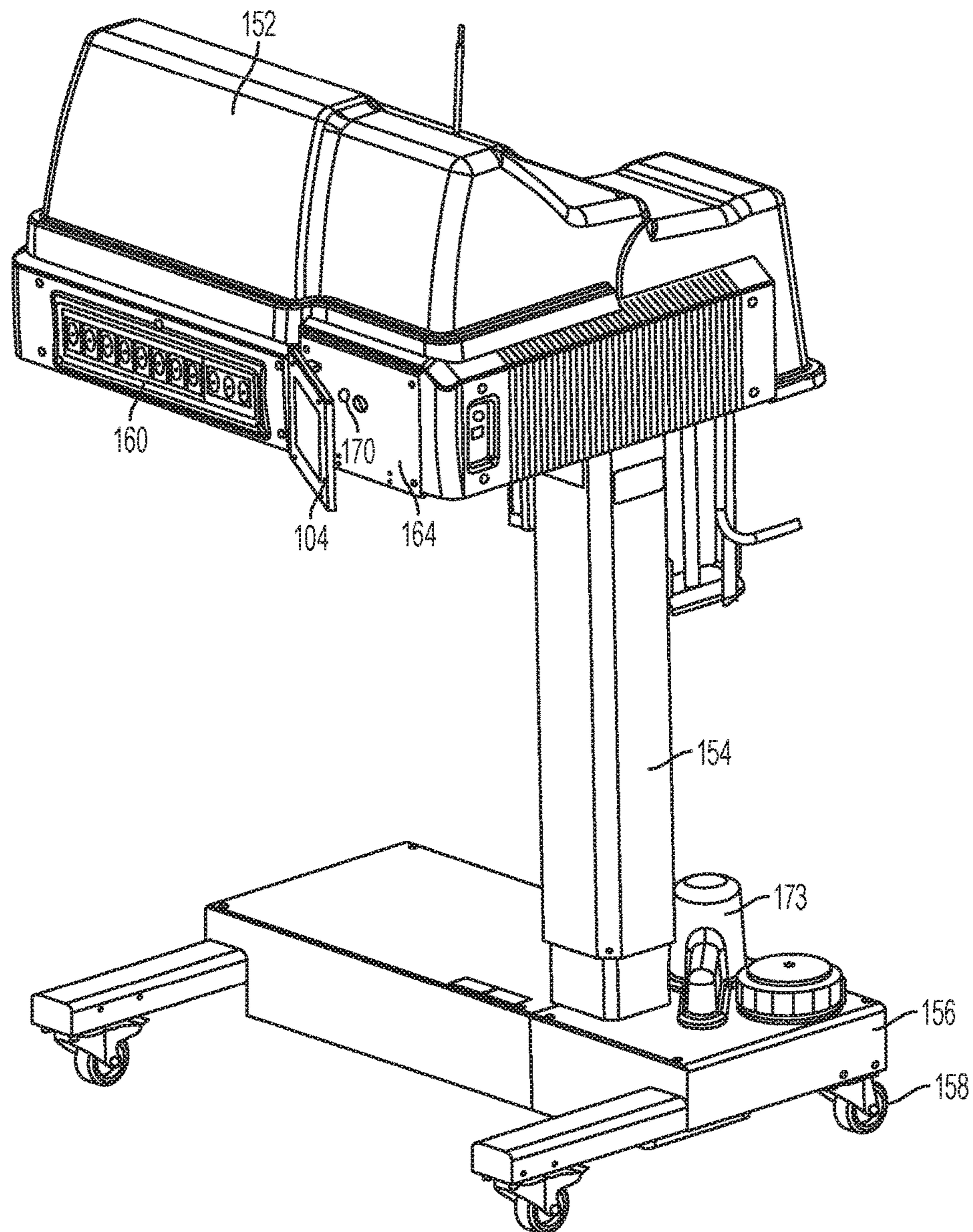
FIG. 4B
