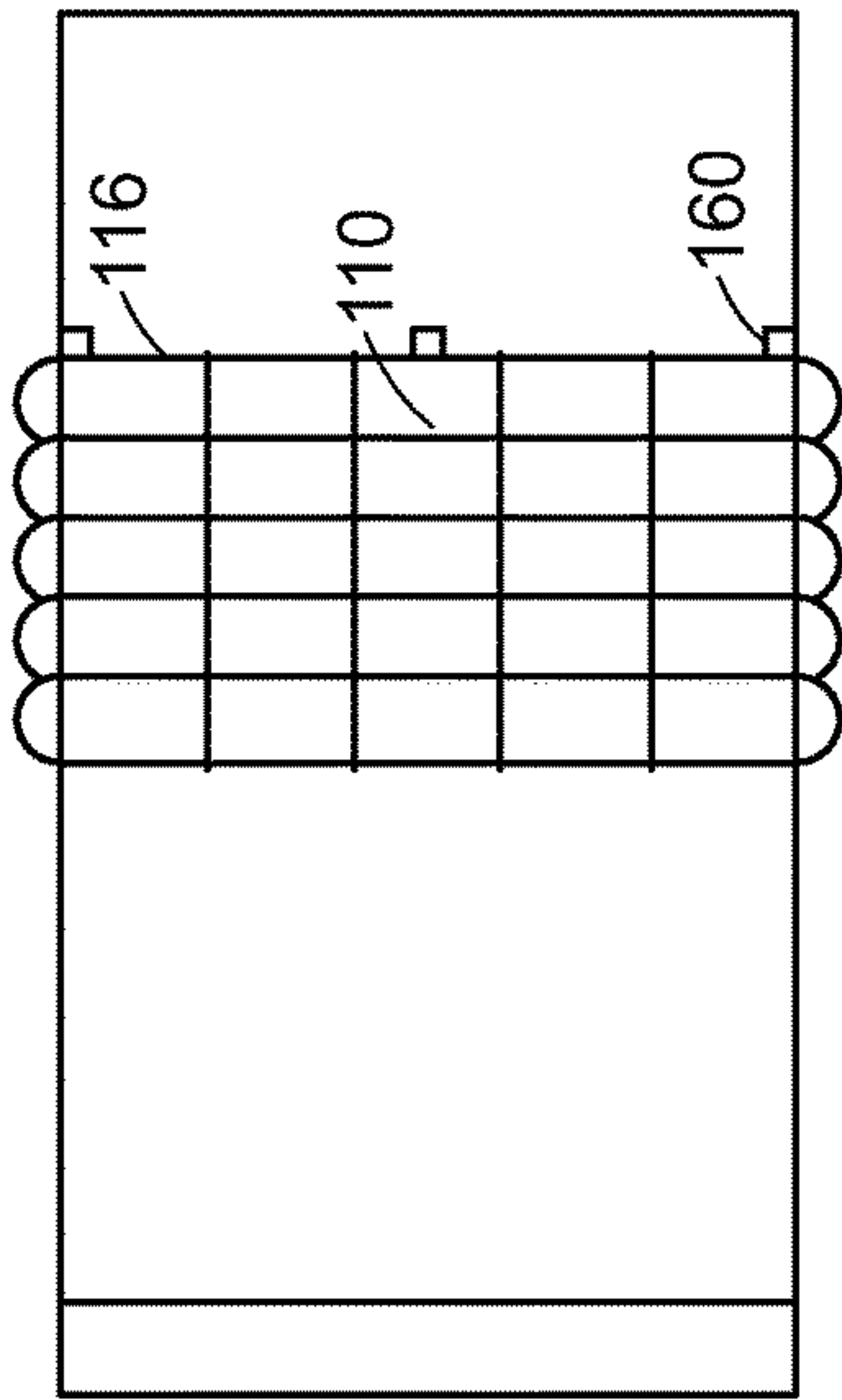
TOP VIEW FIG. 9A
