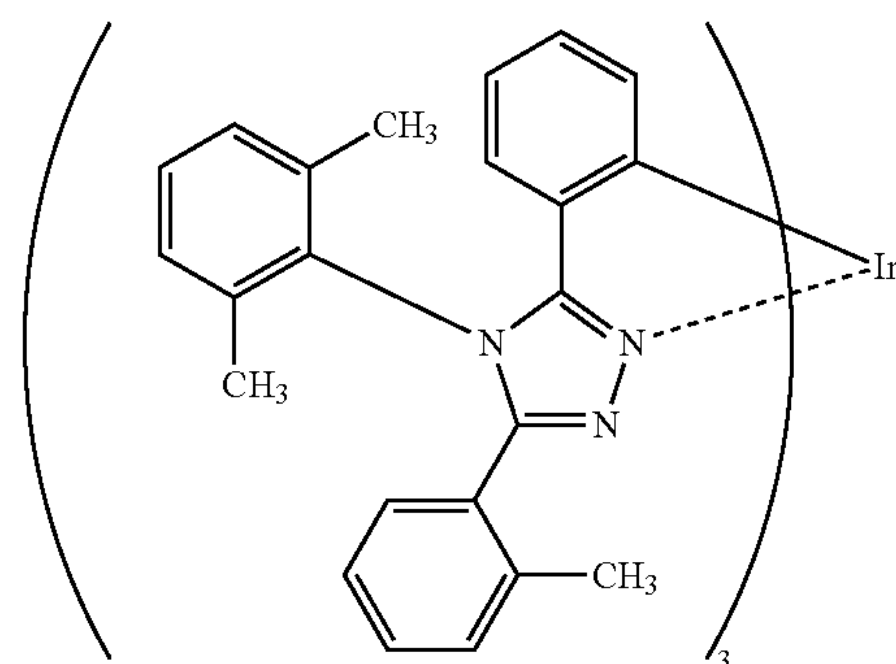
[Ir(mpptz-dmp) 3 ]
