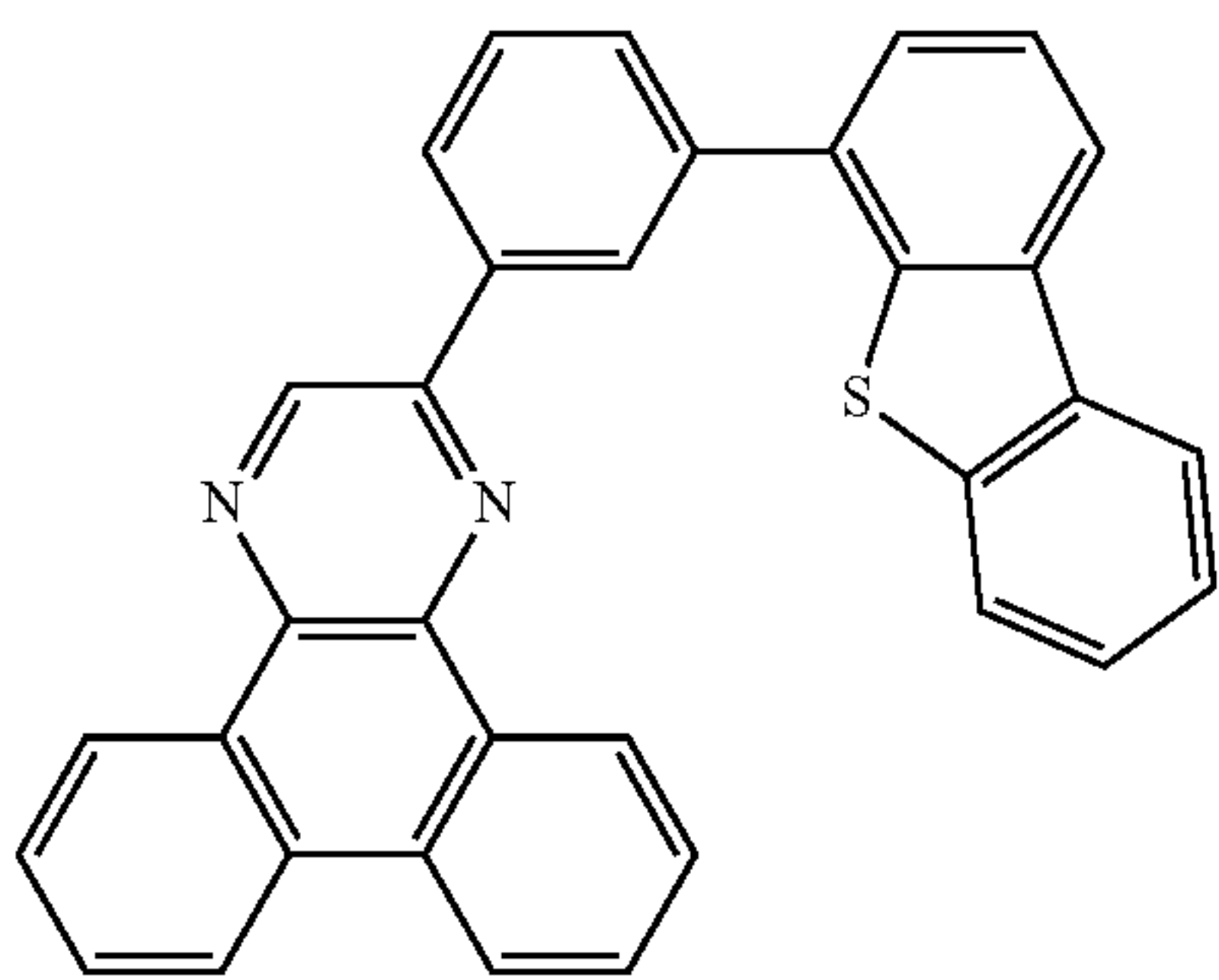
2mDBTPDBq-II
