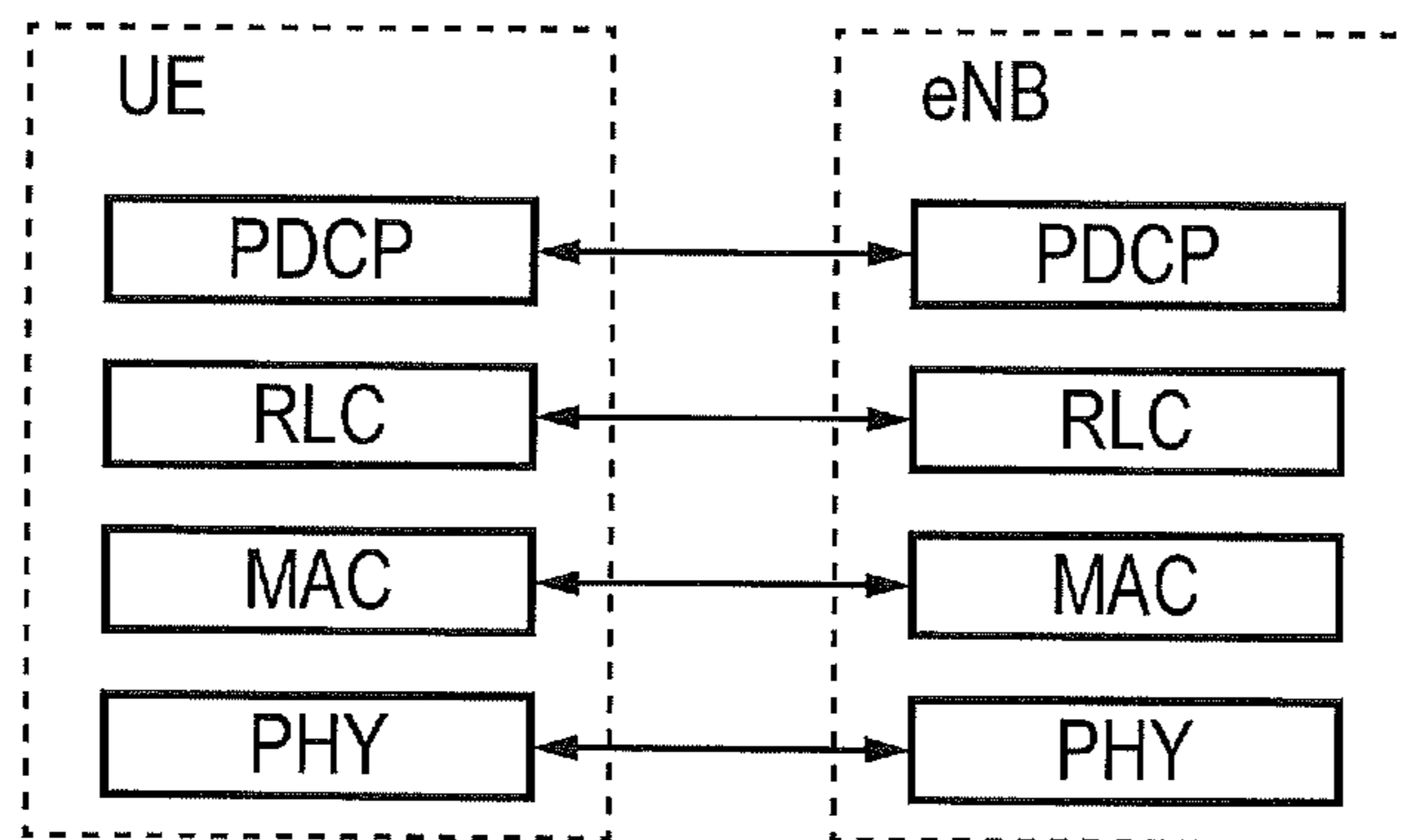
User-plane protocol stack
