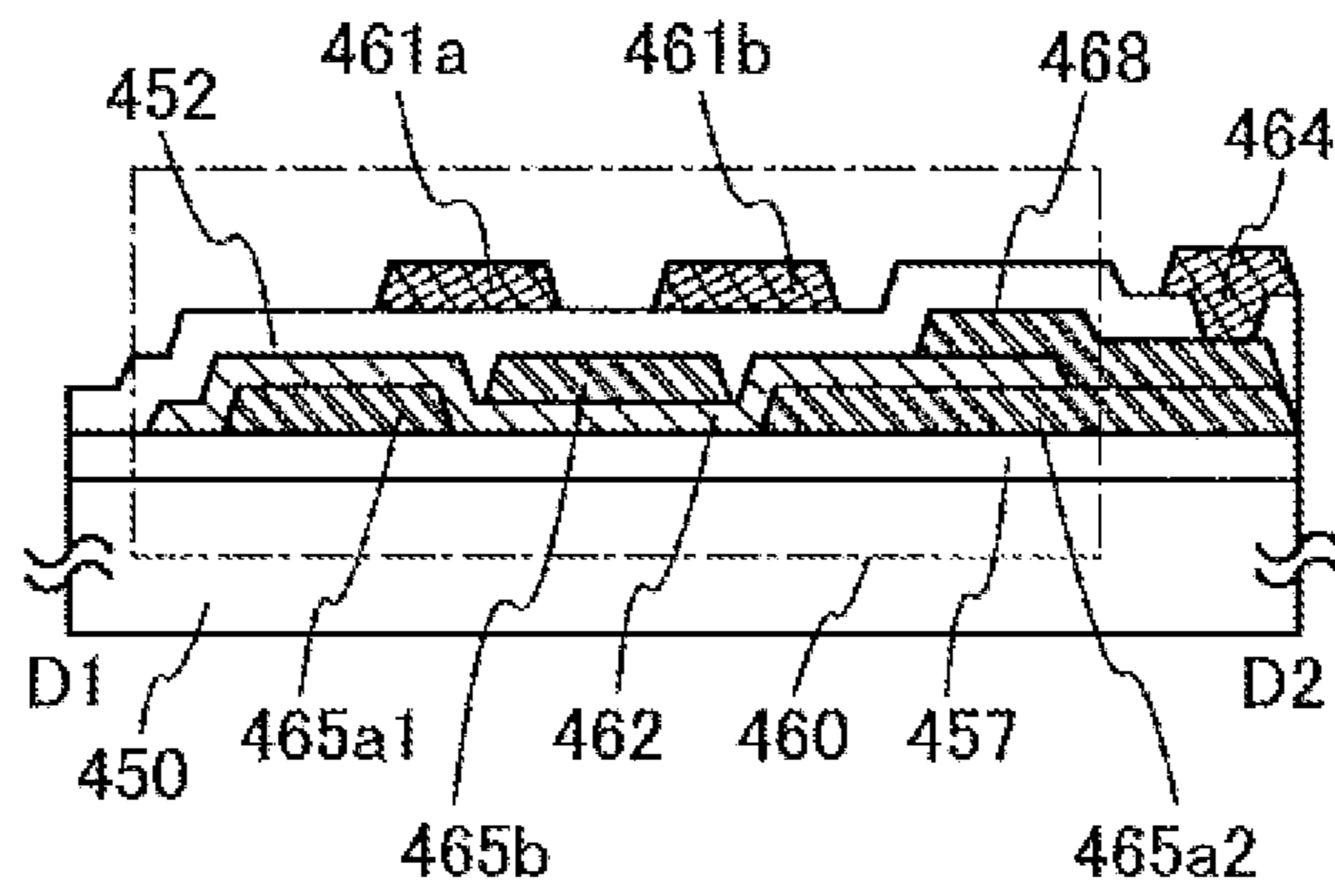
FIG. 5B
