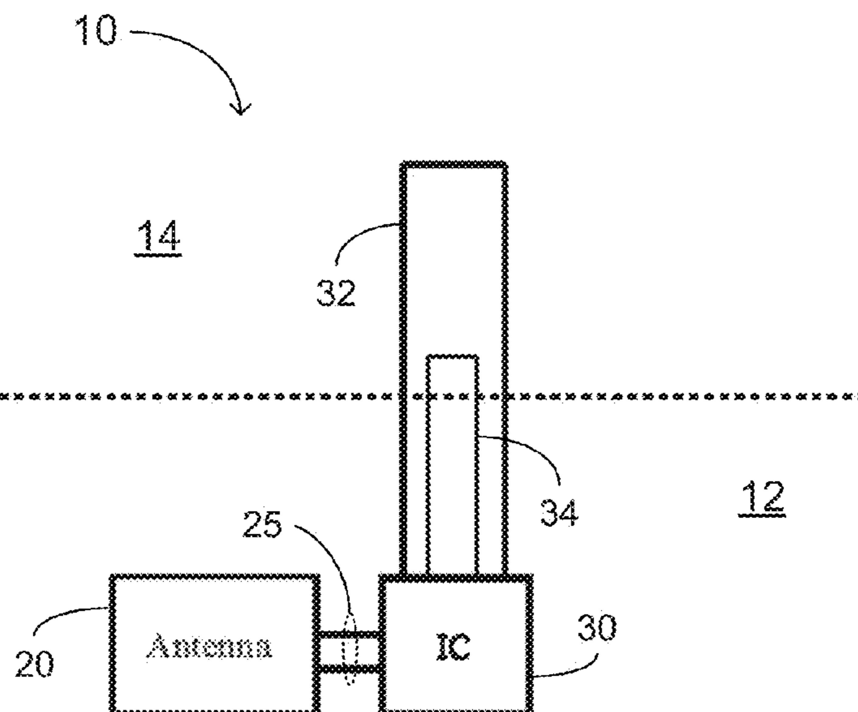
FIG. 1
