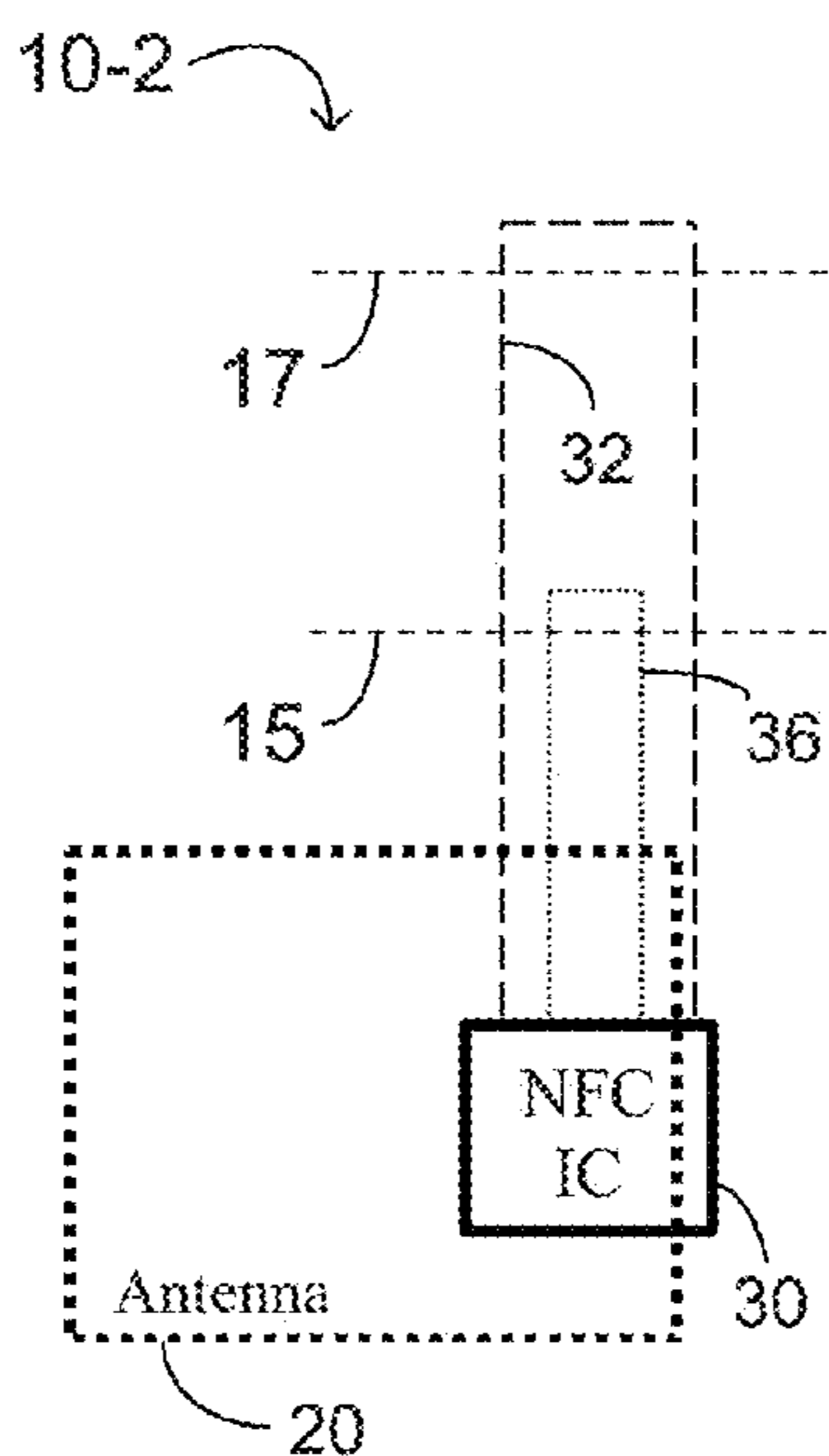
FIG. 2B
