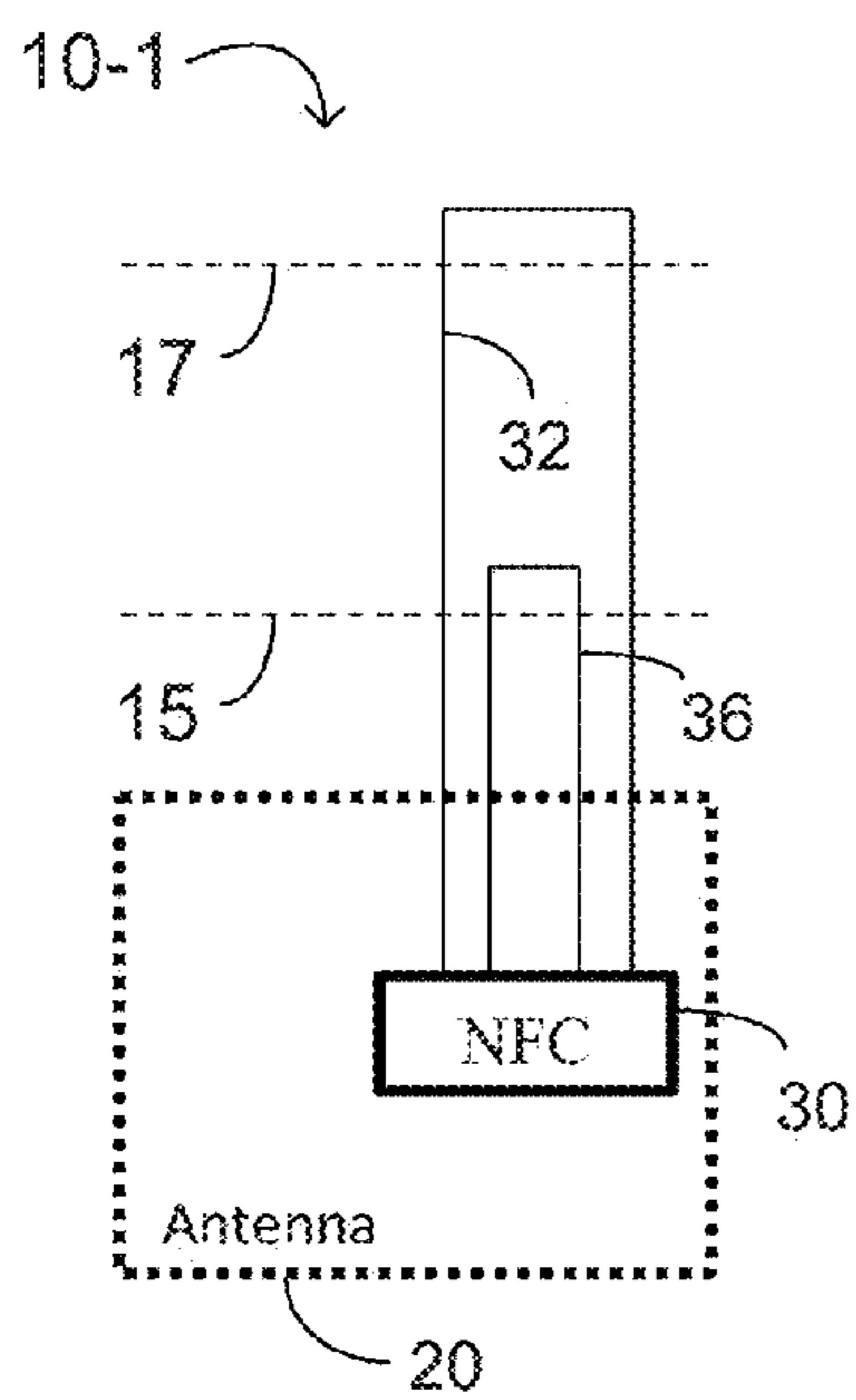
FIG. 2A
