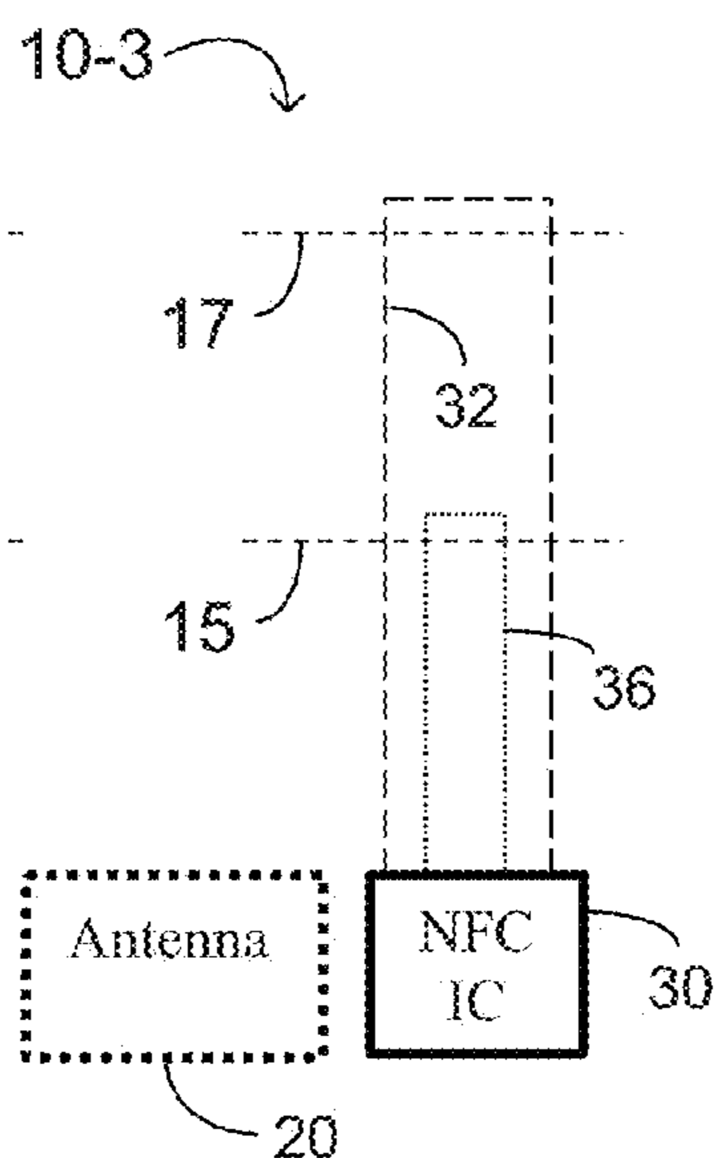
FIG. 2C
