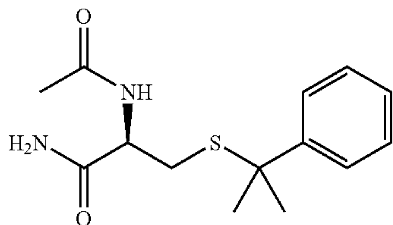
(2R)-2-Acetamido-3-[(2-phenylpropan-2-yl)sulfanyl]propanamide
