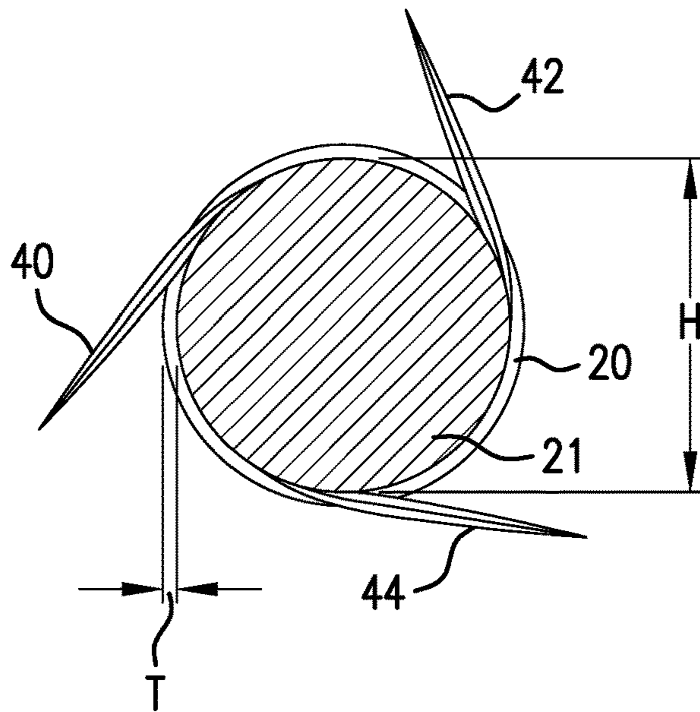
Section A-A'
