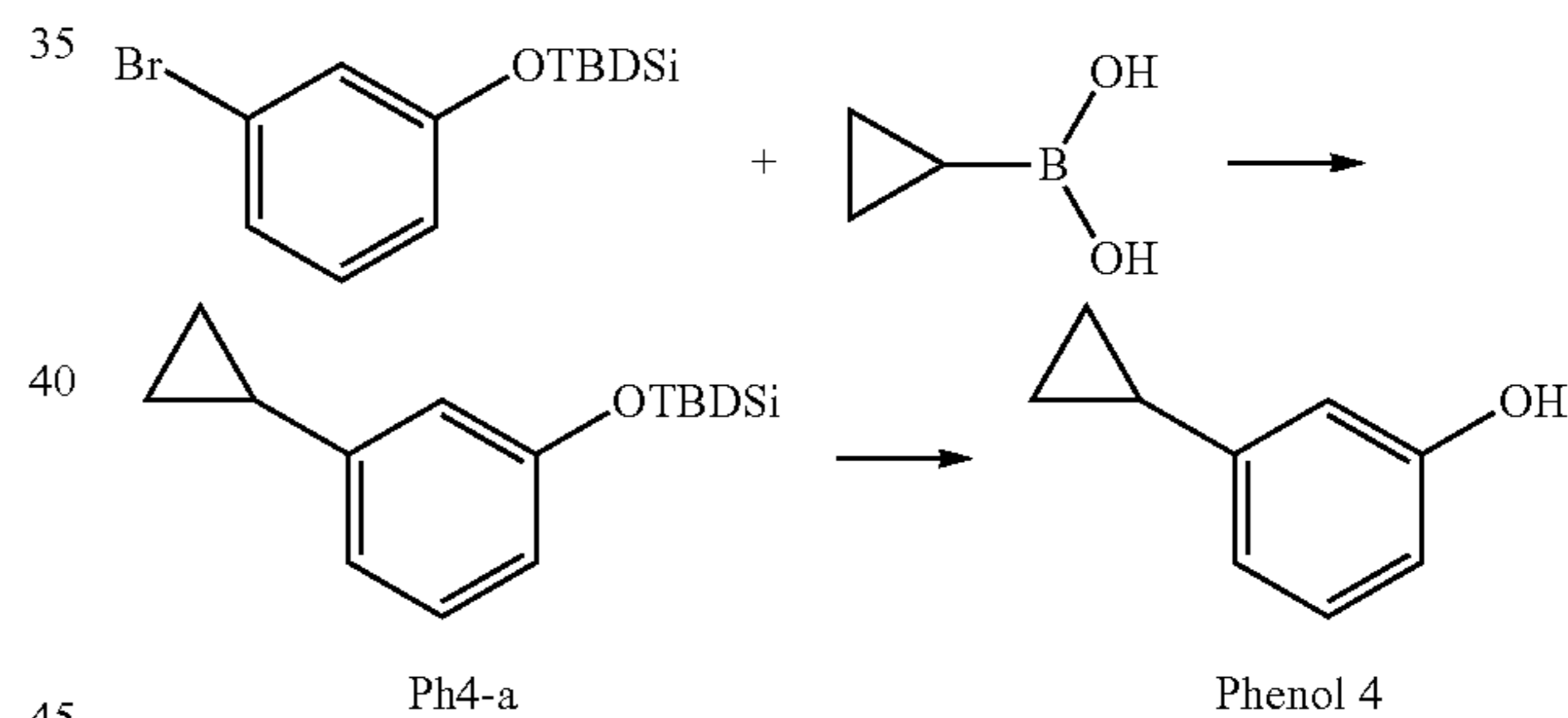
Step a) Tert-butyl(3-cyclopropylphenoxy)dimethylsilane (Ph4-a)
