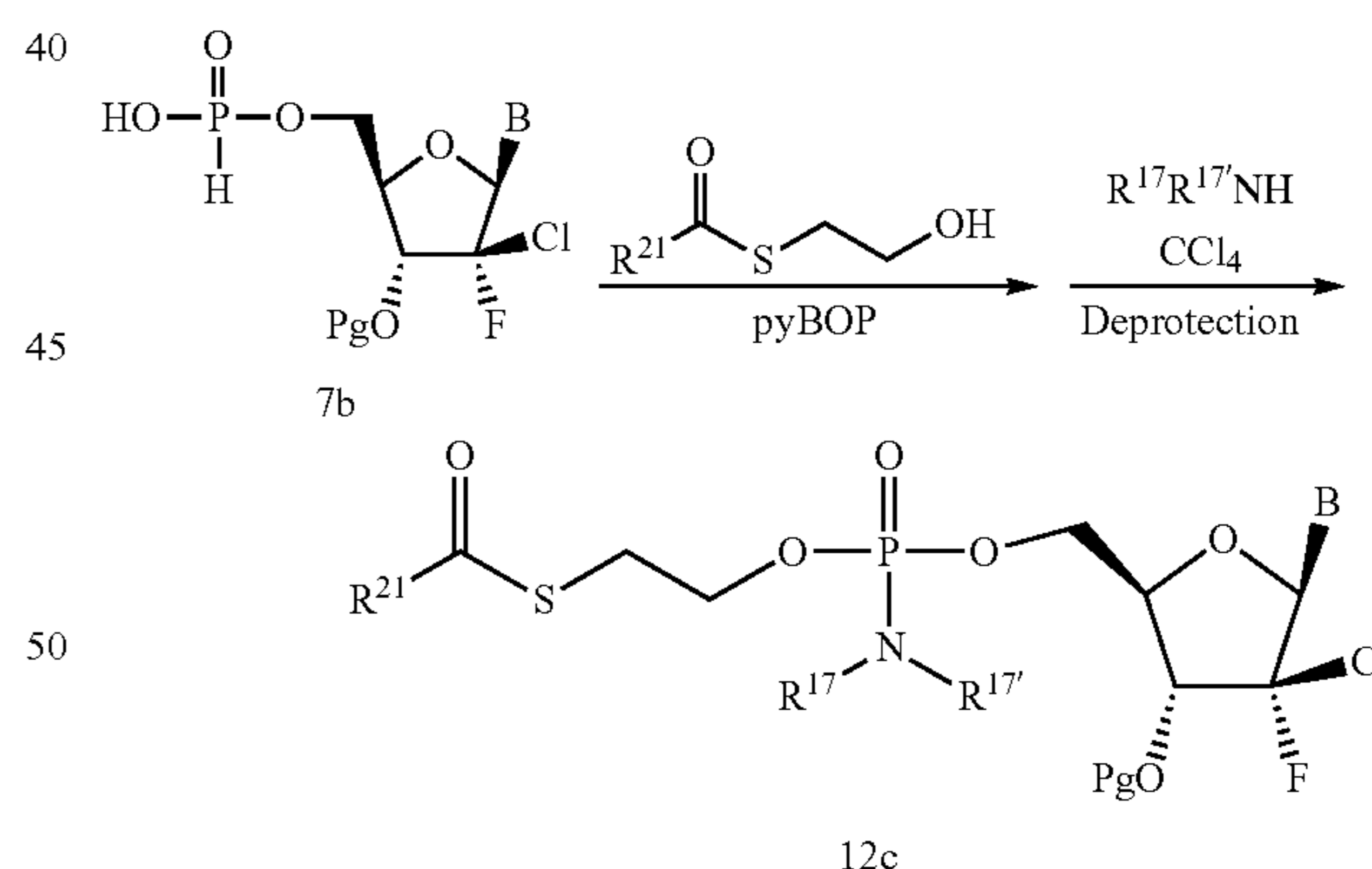
Scheme 12B
