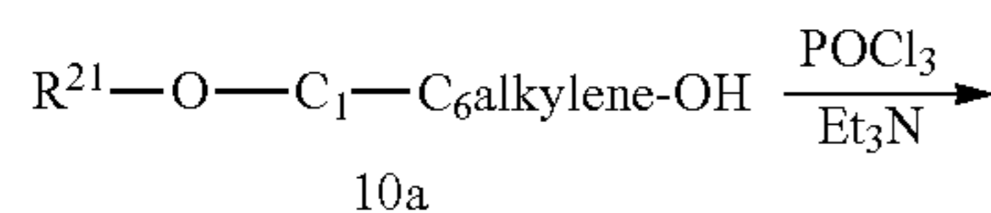
Scheme 10A
