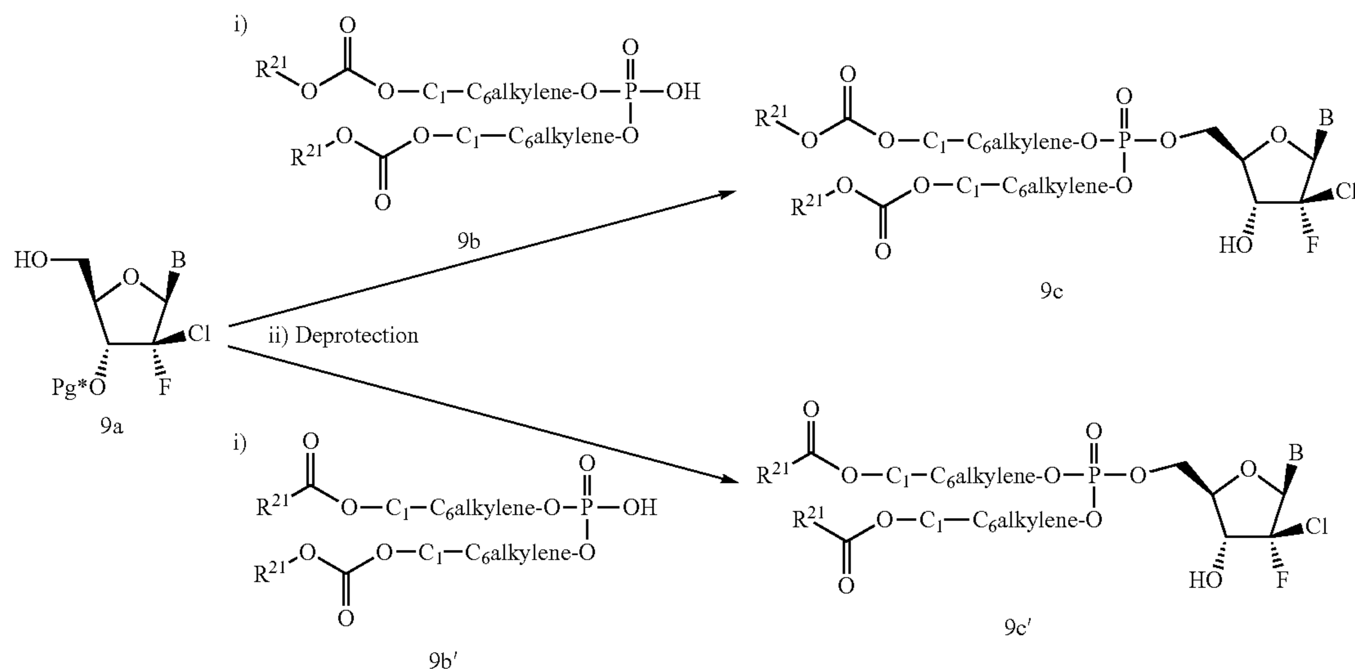
Scheme 9A
