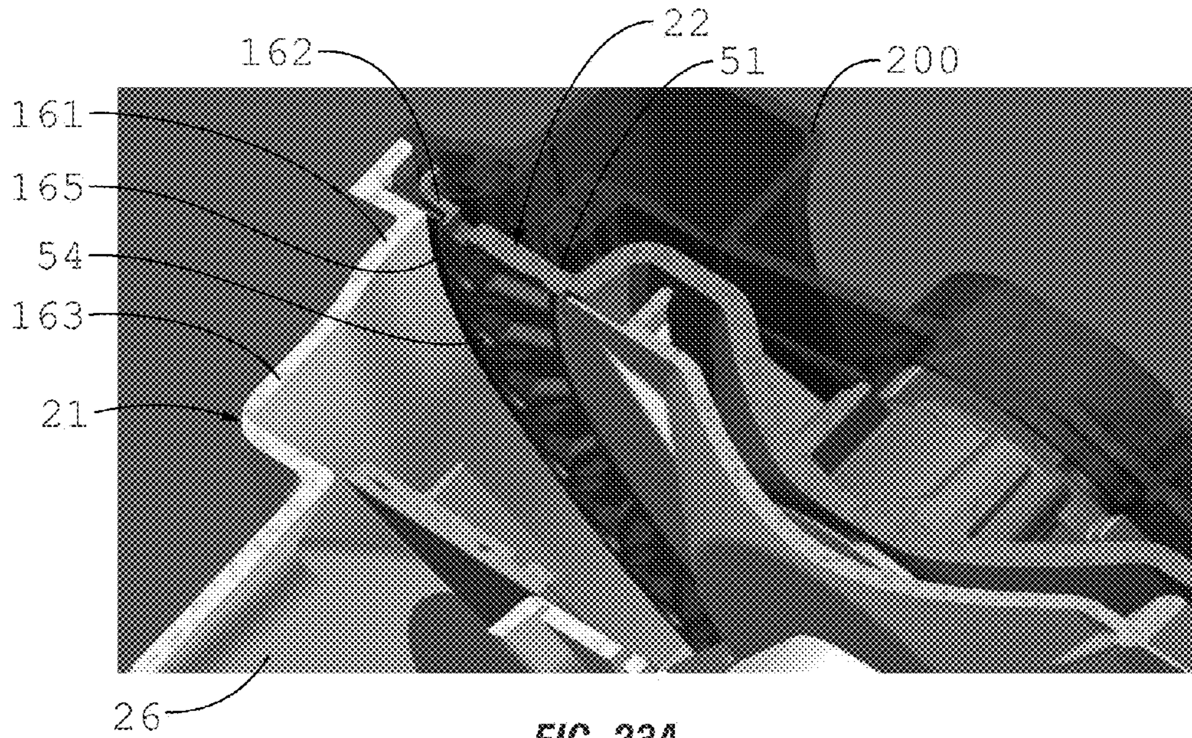
FIG. 23A
