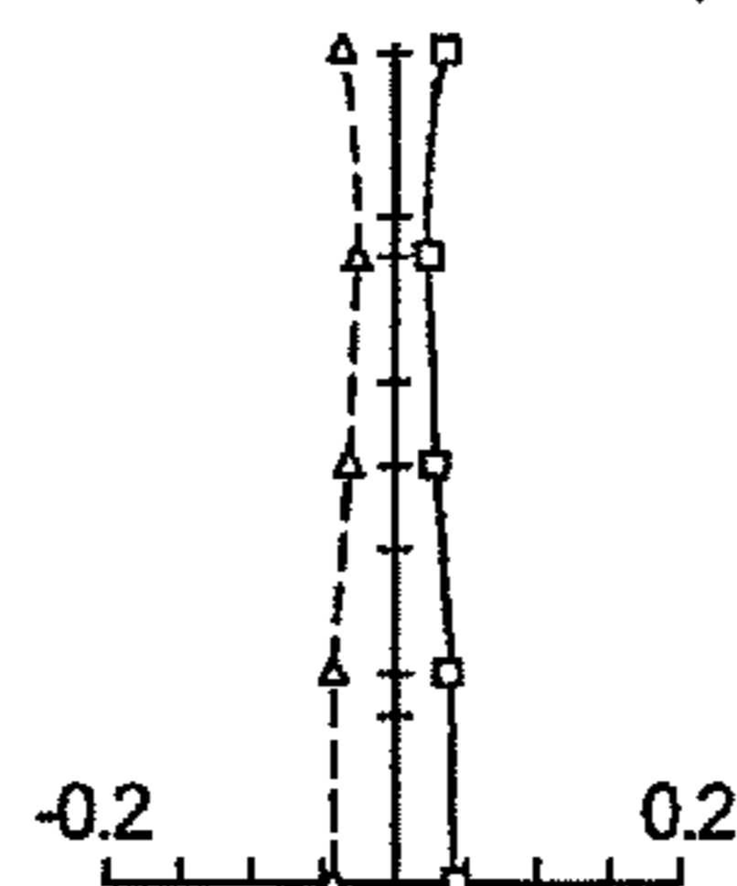
LONGITUDINAL SPHERICAL ABER. (mm)
