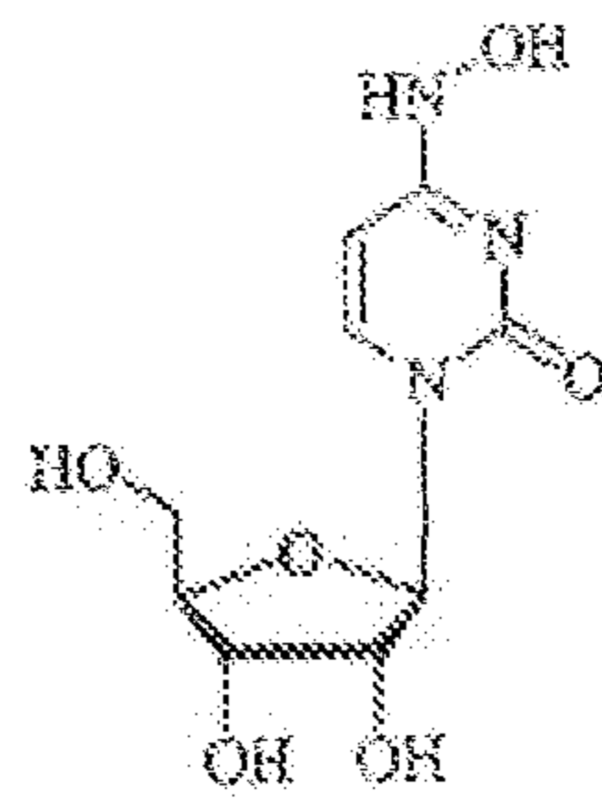
\beta -D-BS
