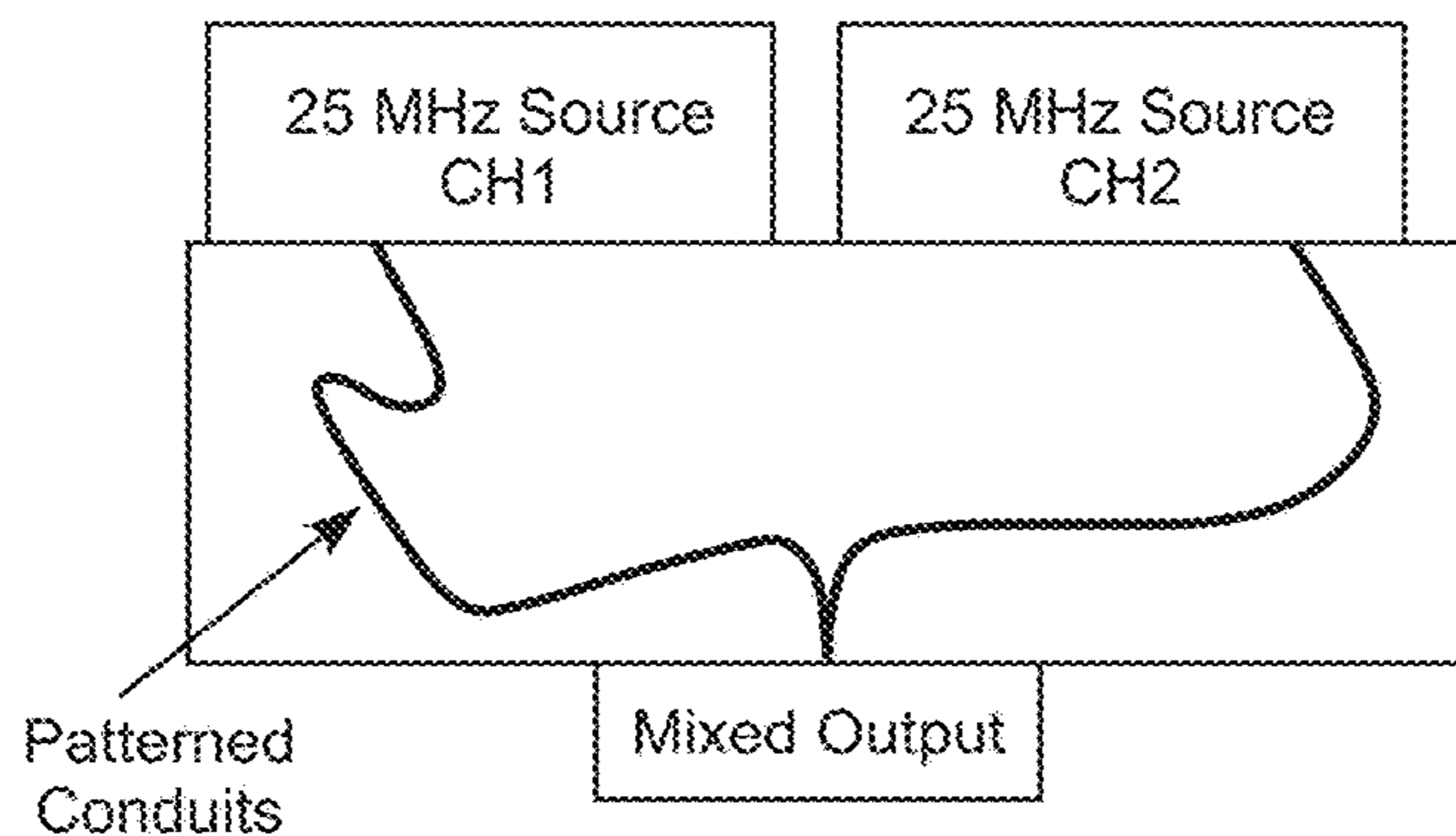
FIG. 8B
