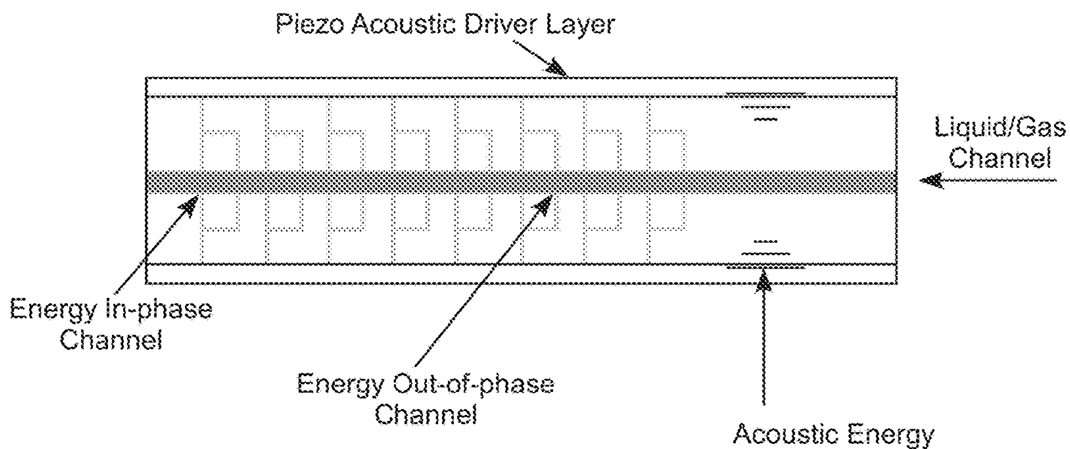
FIG. 8C
