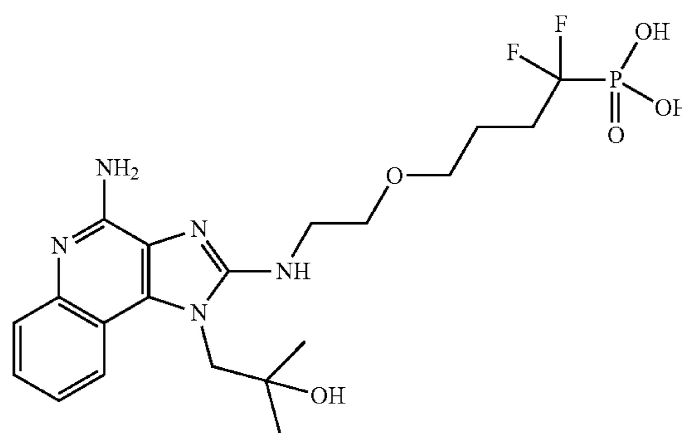
(4-(2-((4-amino-1-(2-hydroxy-2-methylpropyl)-1H-imidazo[4,5-c]quinolin-2-yl)amino)ethoxy)-1,1-difluorobutyl)phosphonic acid
