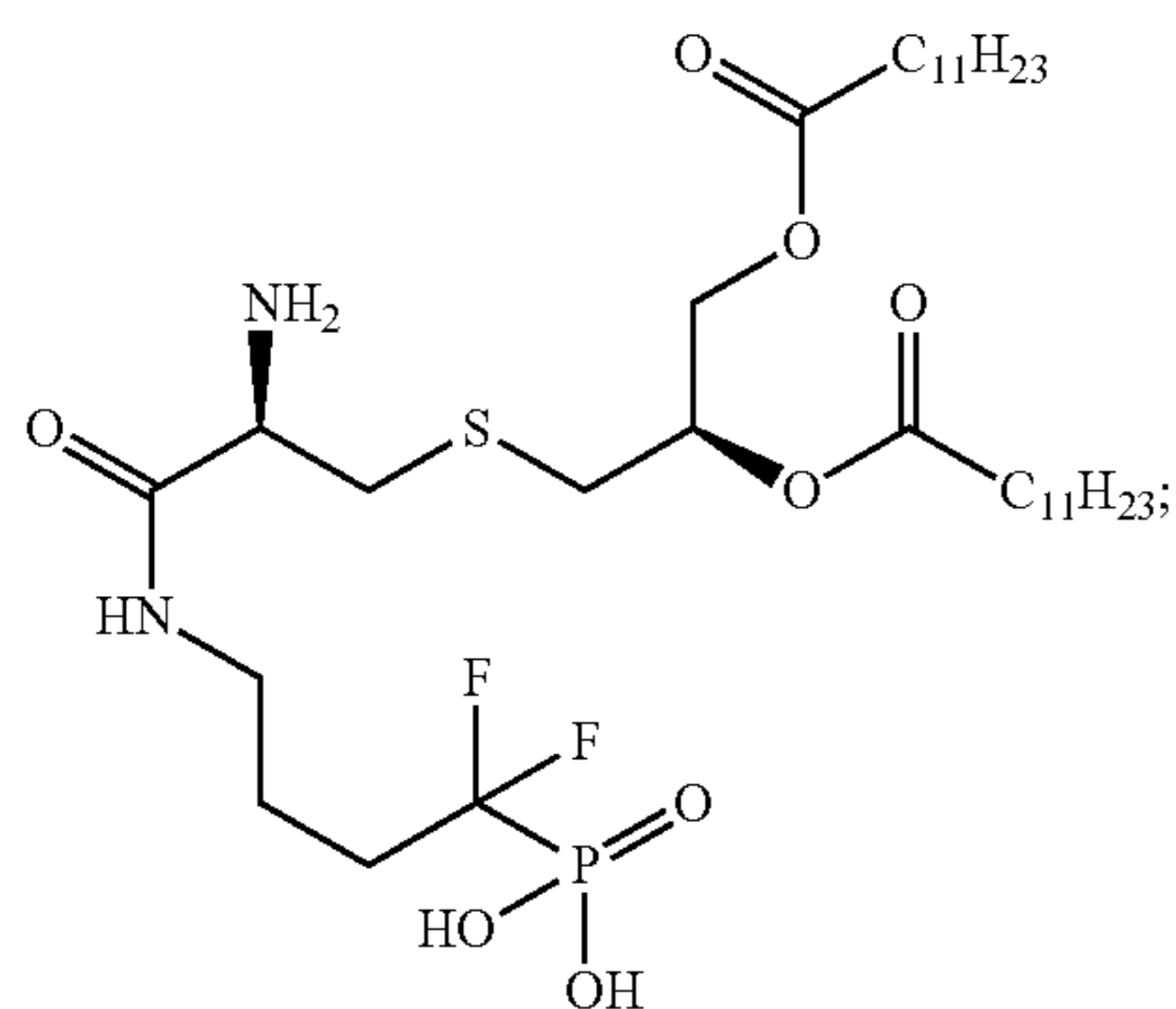
(4-((R)-2-amino-3-(((R)-2,3-bis(dodecanoyloxy)propyl)thio)propanamido)-1,1-difluorobutyl)phosphonic acid
