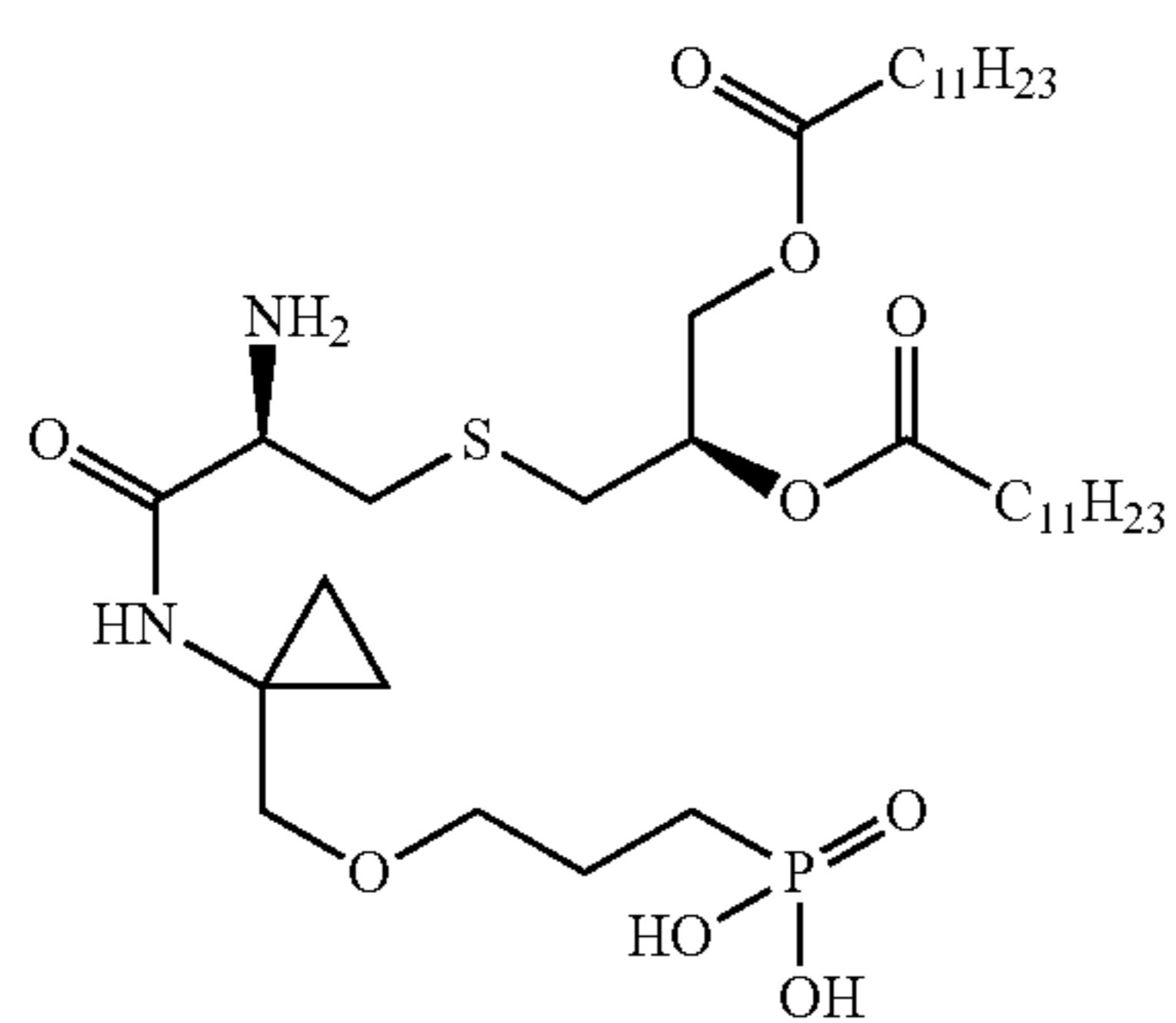
(3-((1-((R)-2-amino-3-(((R)-2,3-bis(dodecanoyloxy)propyl)thio)propanamido)-cyclopropyl)methoxy)propyl)phosphonic acid
