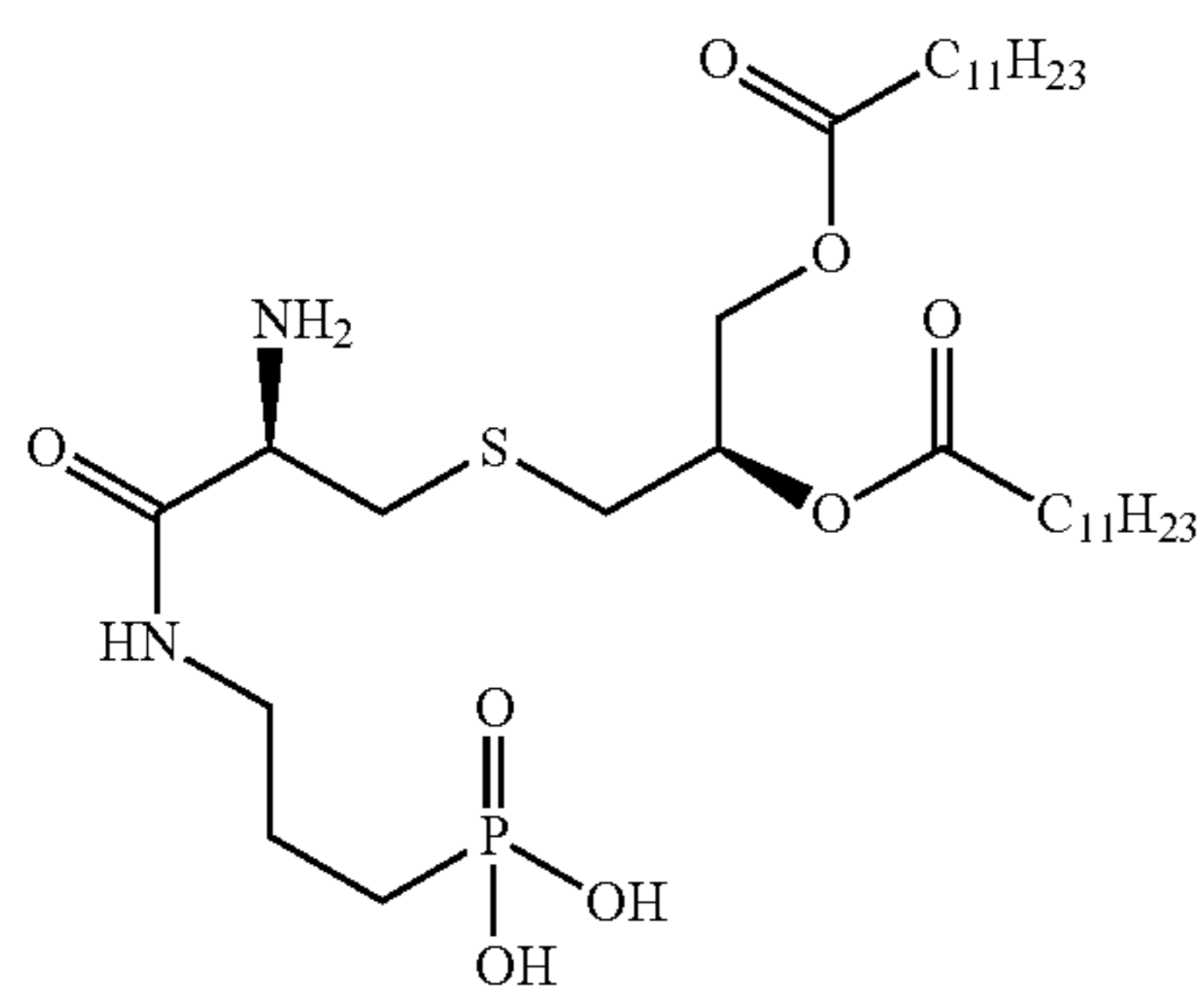
(3-((R)-2-amino-3-(((R)-2,3-bis(dodecanoyloxy)propyl)thio)propanamido)propyl)phosphonic acid
