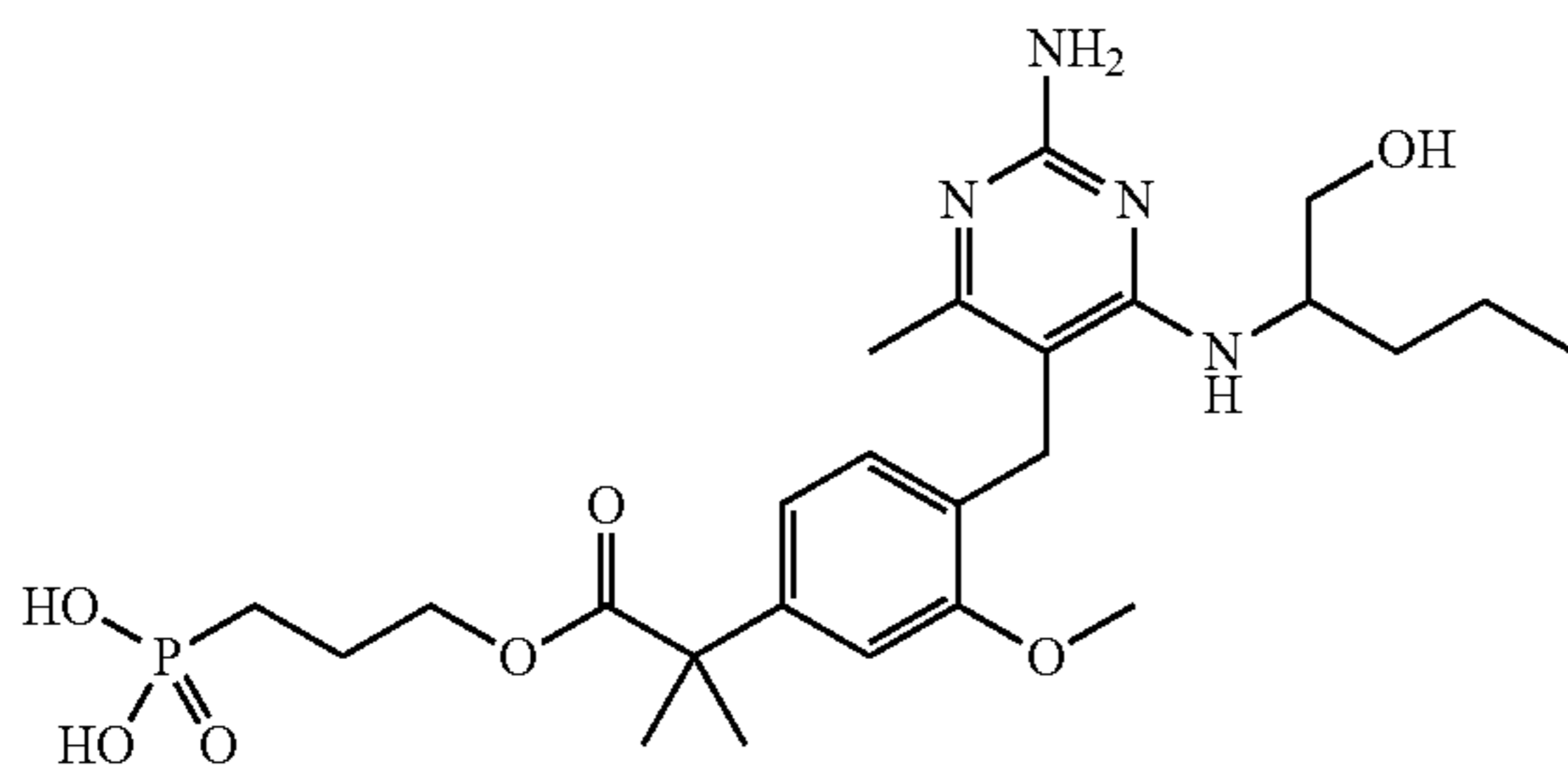
(3-((2-(4-((2-amino-4-((1-hydroxypentan-2-yl)amino)-6-methylpyrimidin-5-yl)methyl)-3-methoxyphenyl)-2-methylpropanoyl)oxy)propyl)phosphonic acid
