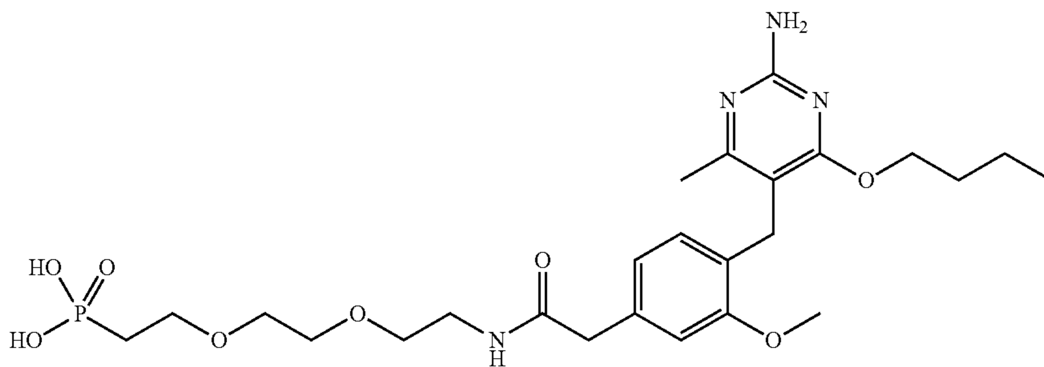
(2-(2-(2-(2-(4-((2-amino-4-butoxy-6-methylpyrimidin-5-yl)methyl)-3-methoxyphenyl)acetamido)ethoxy)ethoxy)ethyl)phosphonic acid
