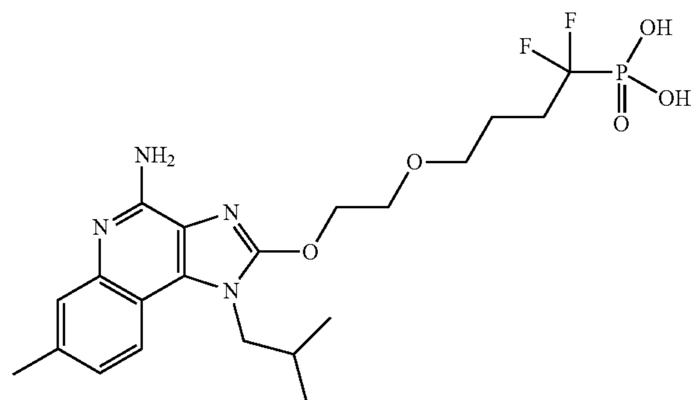
(4-(2-((4-amino-1-isobutyl-7-methyl-1H-imidazo[4,5-c]quinolin-2-yl)oxy)ethoxy)-1,1-difluorobutyl)phosphonic acid
