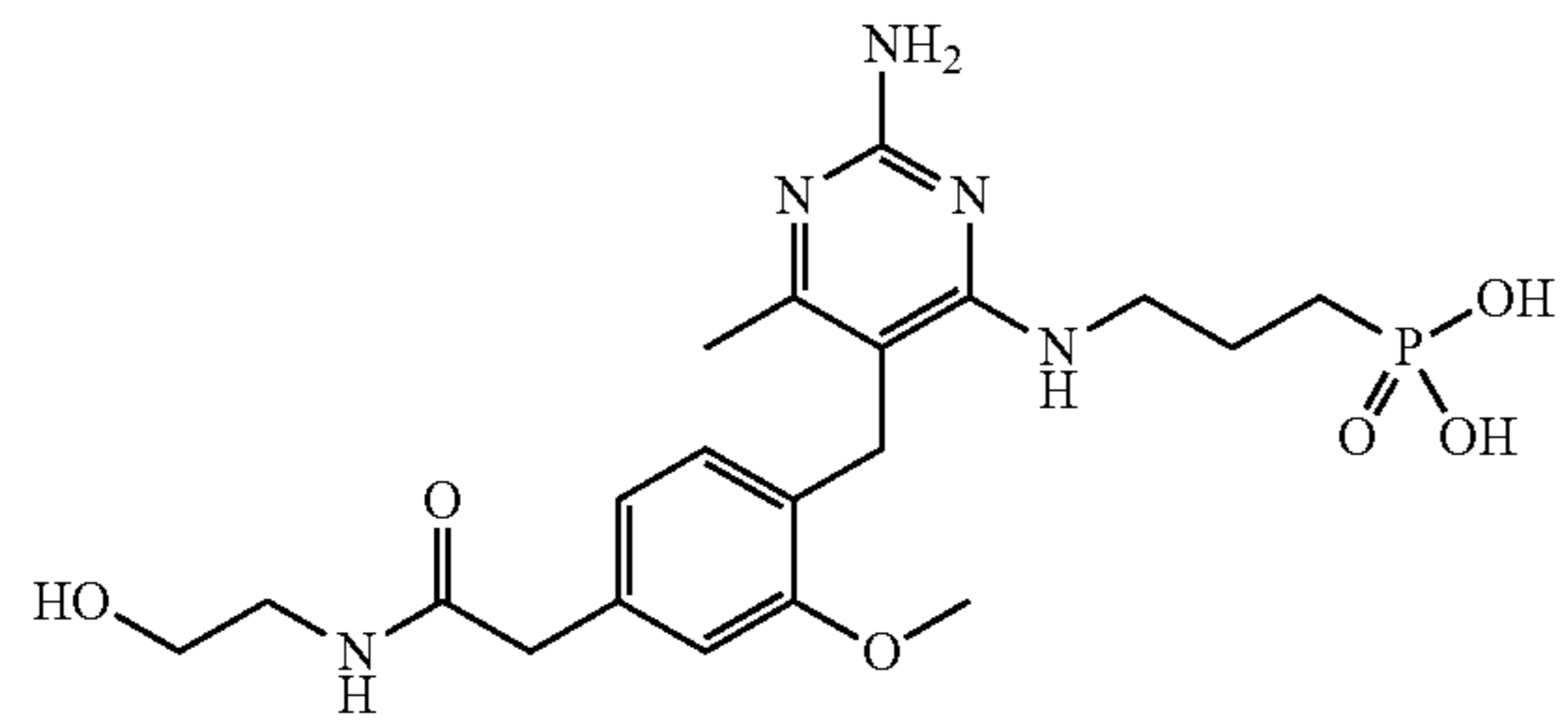
(3-((2-amino-5-(4-(2-((2-hydroxyethyl)amino)-2-oxoethyl)-2-methoxybenzyl)-6-methylpyrimidin-4-yl)amino)propyl)phosphonic acid
