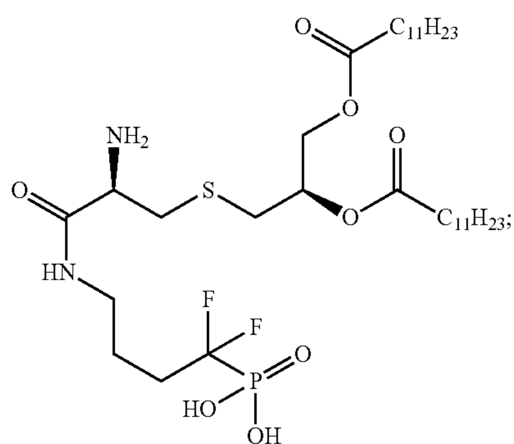
(4-((R)-2-amino-3-(((R)-2,3-bis(dodecanoyloxy)propyl)thio)propanamido)-1,1-difluorobutyl)phosphonic acid
