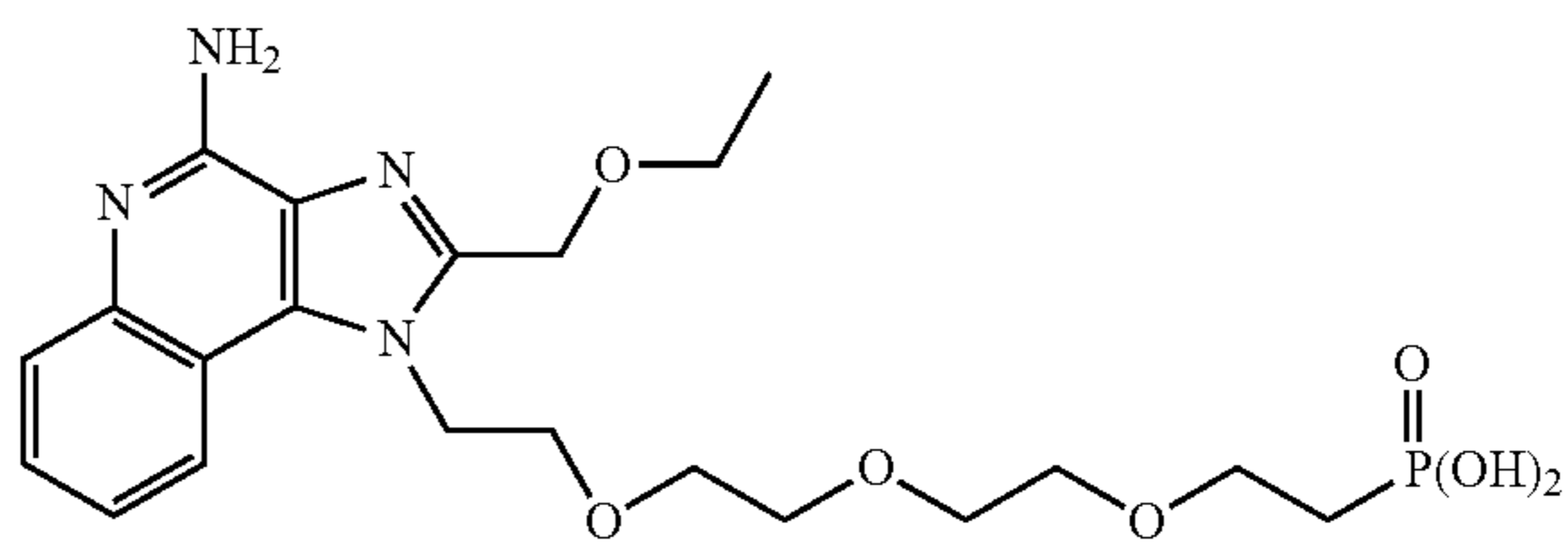
(2-(2-(2-(2-(4-amino-2-(ethoxymethyl)-1H-imidazo[4,5-c]quinolin-1-yl)ethoxy)ethoxy)ethoxy)ethyl)phosphonic acid
