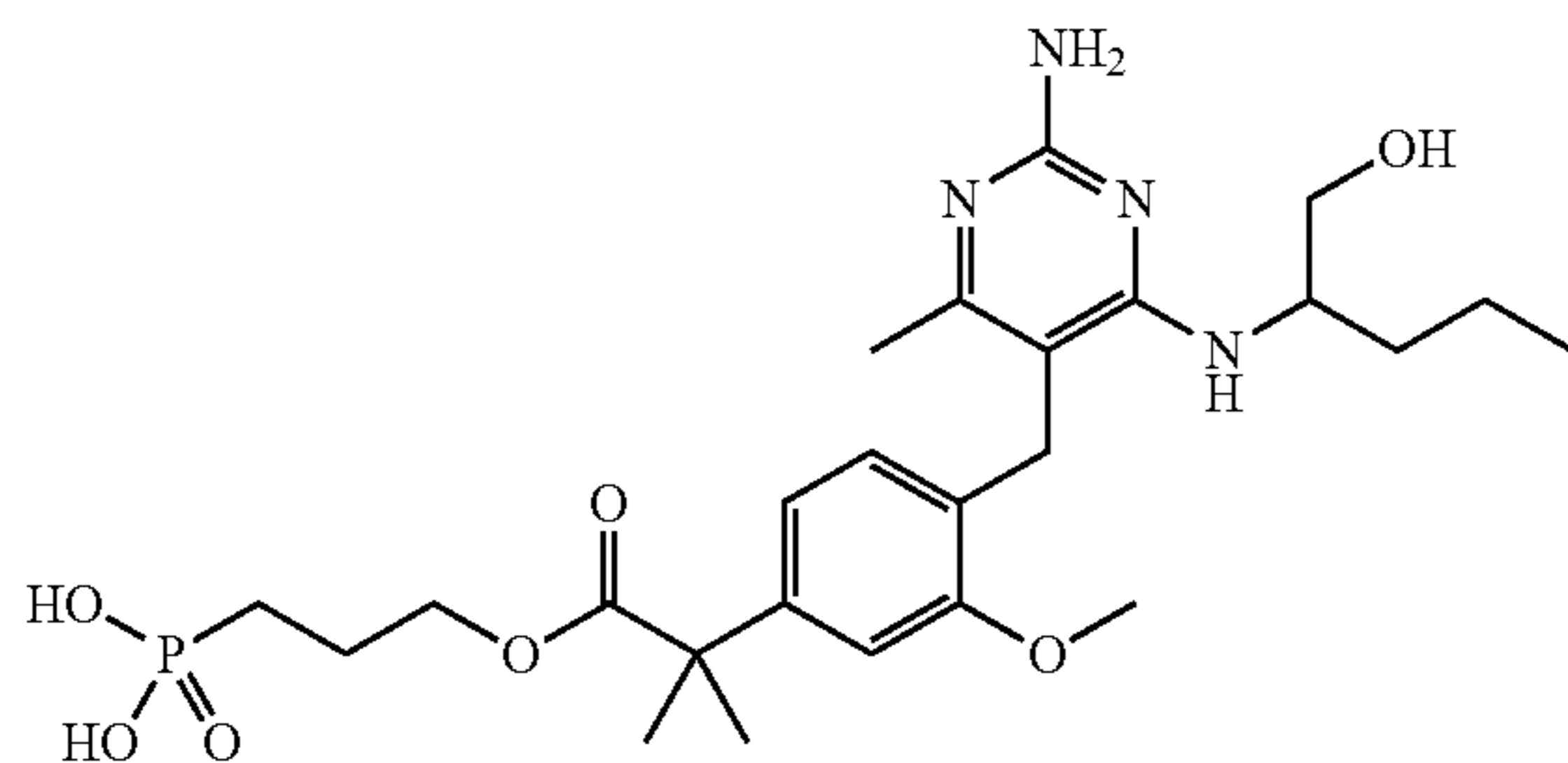
(3-((2-(4-((2-amino-4-((1-hydroxypentan-2-yl)amino)-6-methylpyrimidin-5-yl)methyl)-3-methoxyphenyl)-2-methylpropanoyl)oxy)propyl)phosphonic acid
