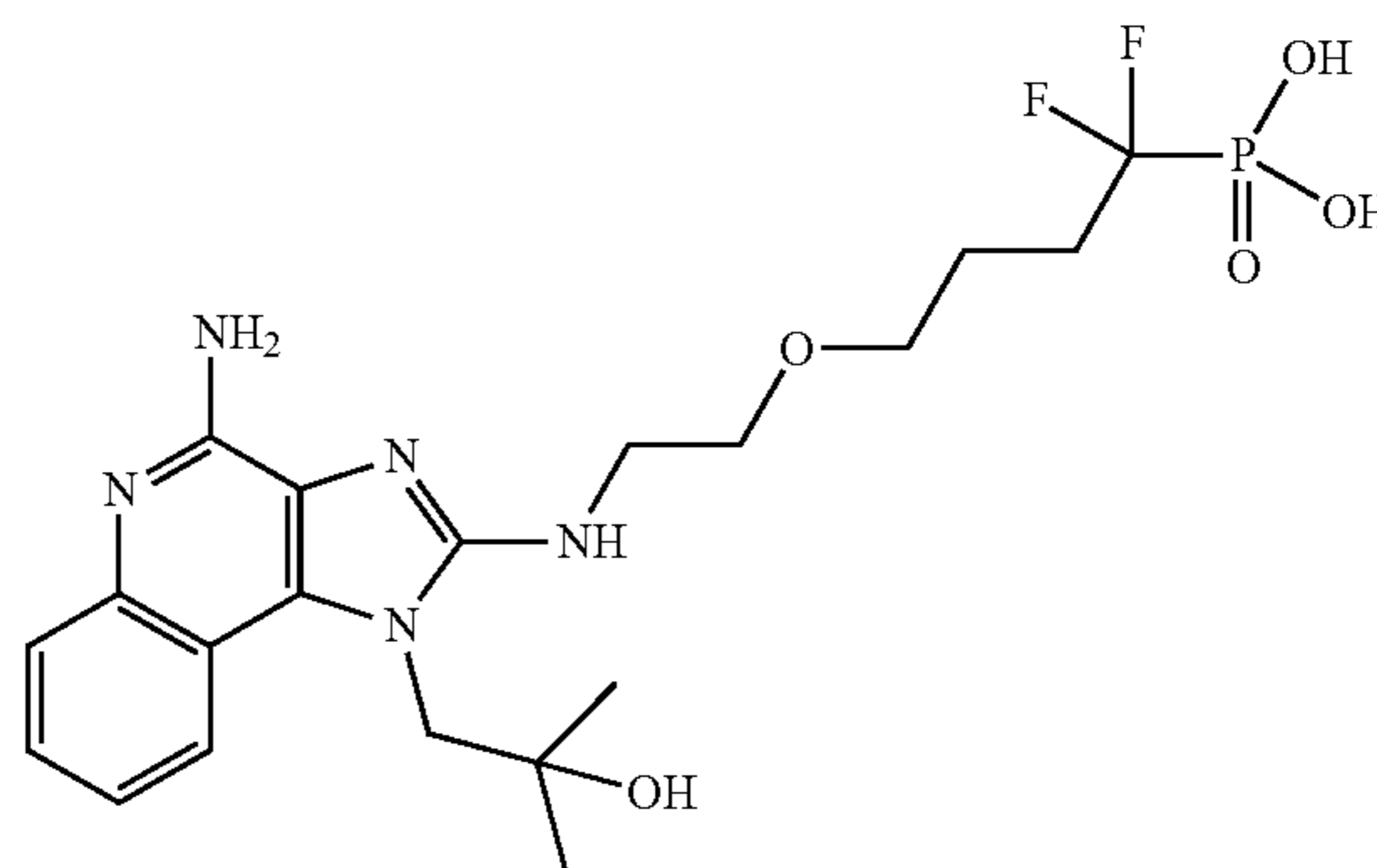
(4-(2-((4-amino-1-(2-hydroxy-2-methylpropyl)-1H-imidazo[4,5-c]quinolin-2-yl)amino)ethoxy)-1,1-difluorobutyl)phosphonic acid
