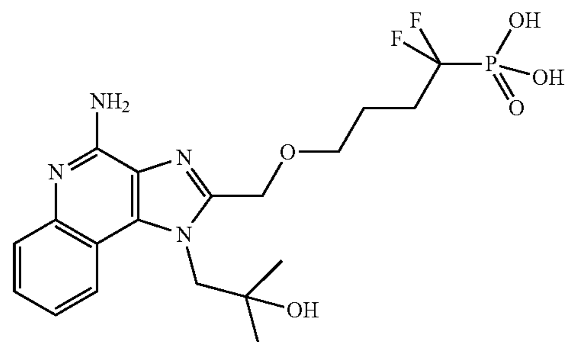
(4-((4-amino-1-(2-hydroxy-2-methylpropyl)-1H-imidazo[4,5-c]quinolin-2-yl)methoxy)-1,1-difluorobutyl)phosphonic acid
