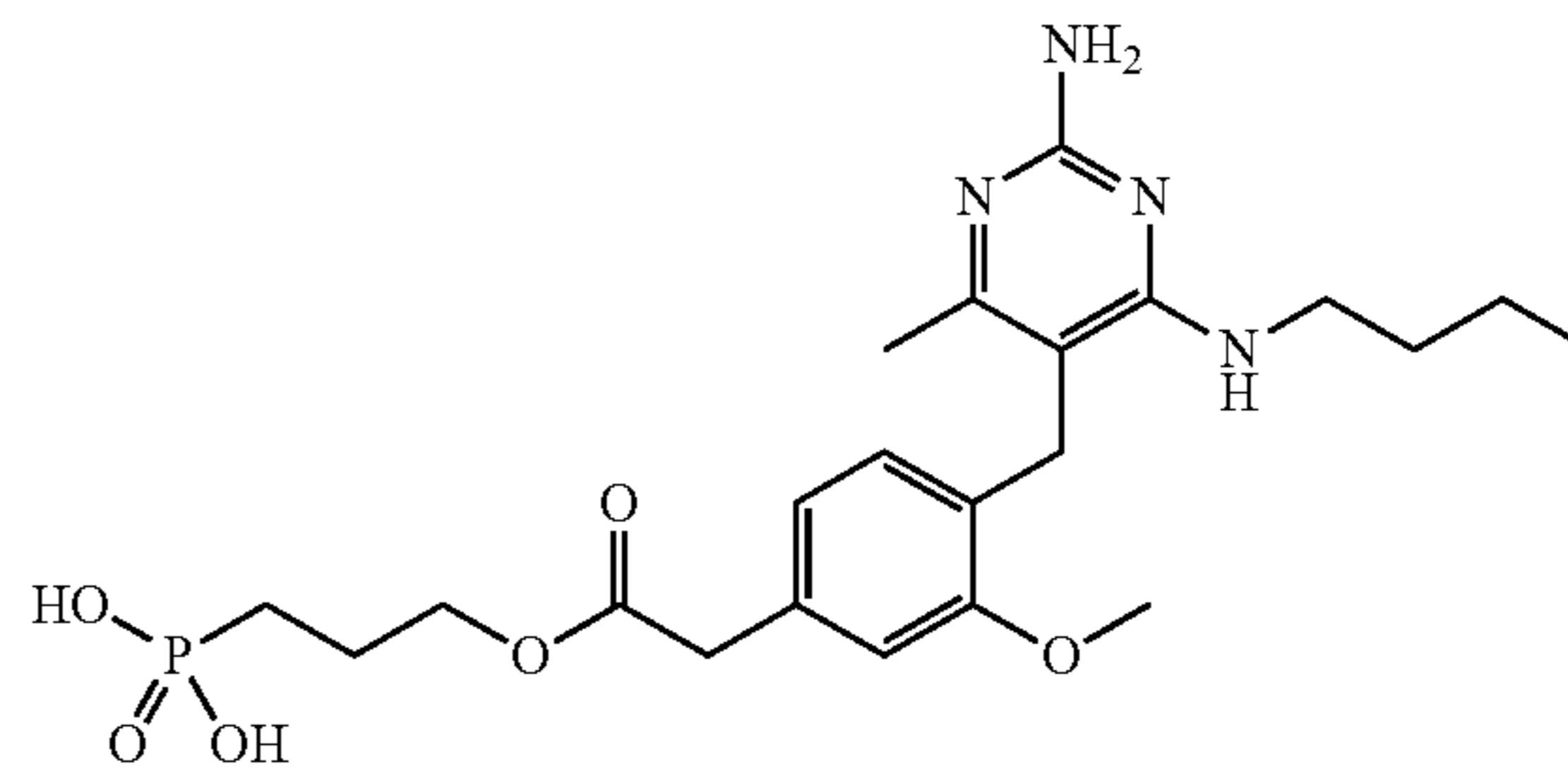
(3-(2-(4-((2-amino-4-(butylamino)-6-methylpyrimidin-5-yl)methyl)-3-methoxyphenyl)acetoxyl)propyl)phosphonic acid
