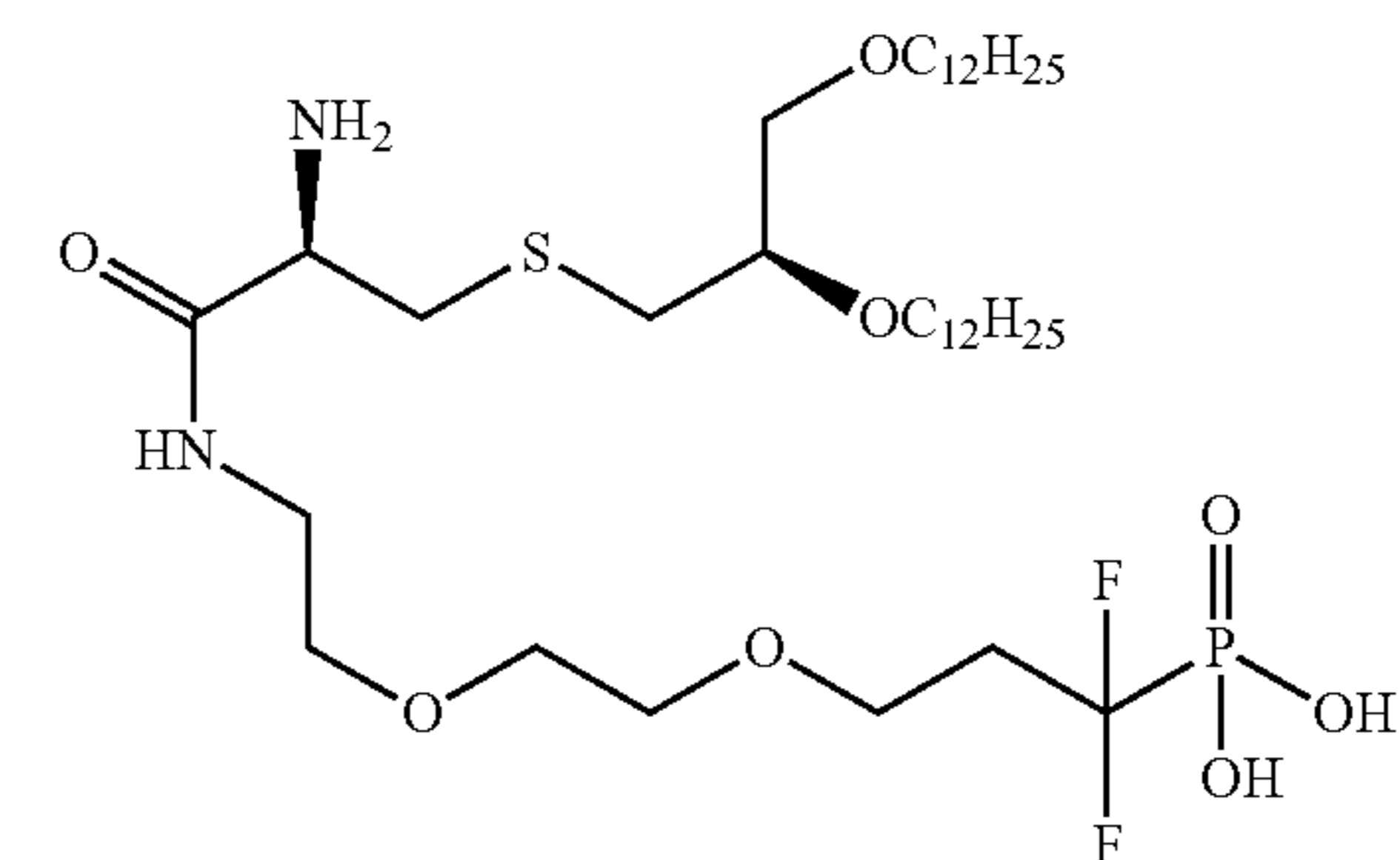
((12R,16R)-12-amino-16-(dodecyloxy)-1,1-difluoro-11-oxo-4,7,18-trioxa-14-thia-10-azatriacetyl)phosphonic acid
