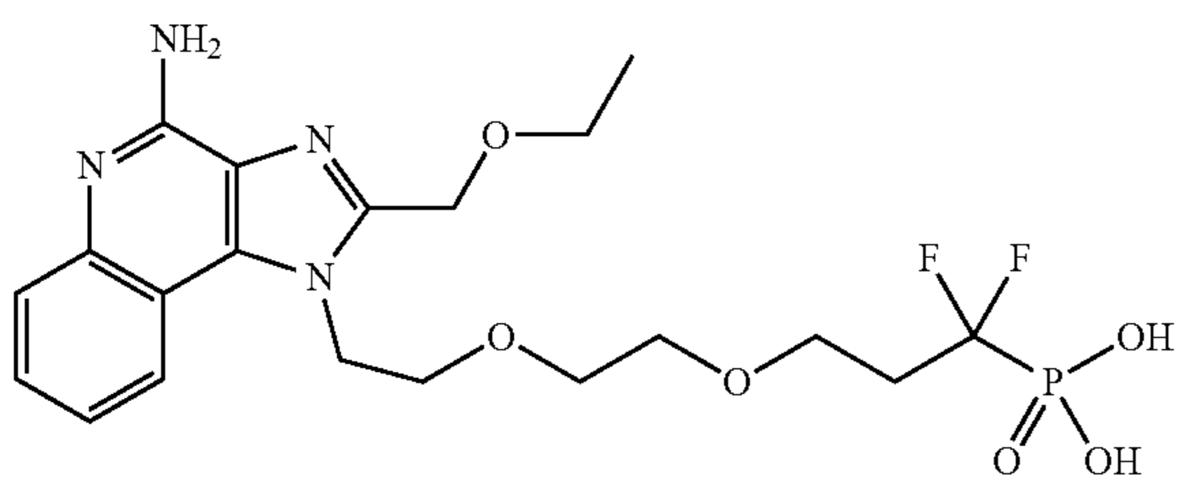
(3-(2-(2-(4-amino-2-(ethoxymethyl)-1H-imidazo[4,5-c]quinolin-1-yl)ethoxy)ethoxy)-1,1-difluoropropyl)phosphonic acid
