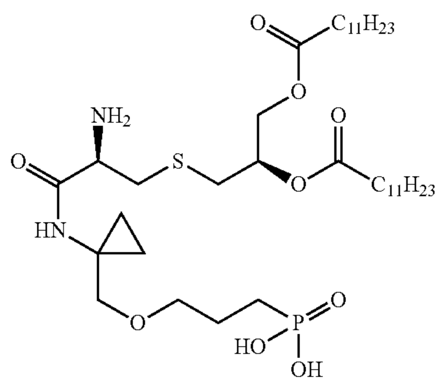
(3-((1-((R)-2-amino-3-(((R)-2,3-bis(dodecanoyloxy)propyl)thio)propanamido)-cyclopropyl)methoxy)propyl)phosphonic acid
