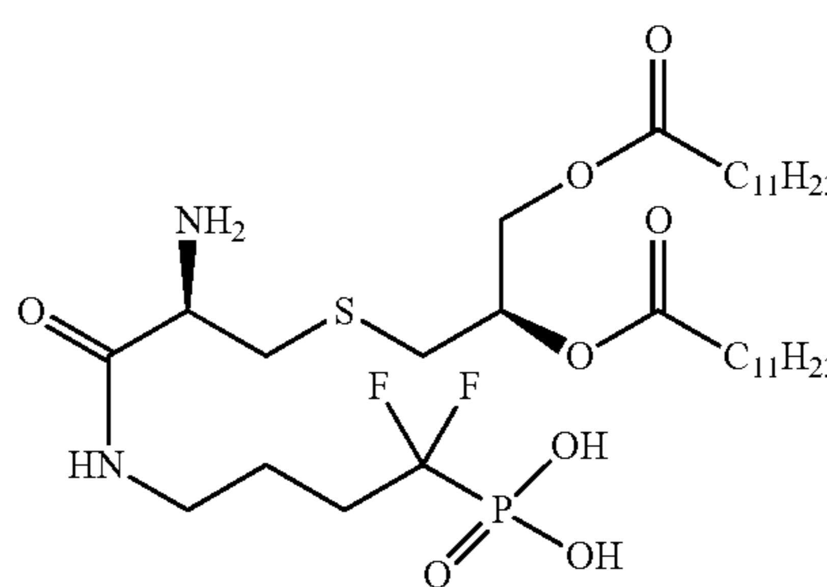
4-((R)-2-amino-3-((R)-2,3-bis(dodecanoyloxy)propylthio)propanamido)-1,1-difluorobutylphosphonic acid
