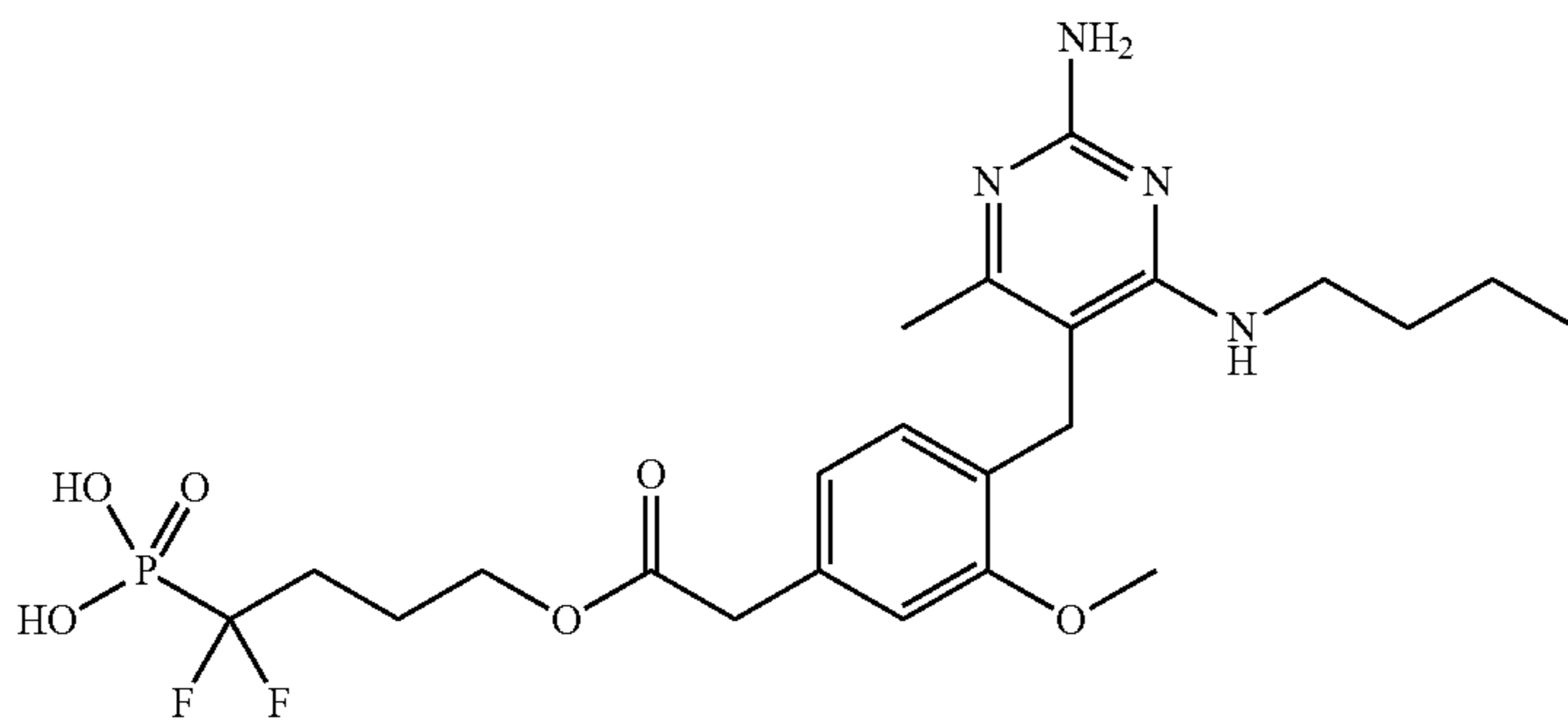
(4-(2-(4-((2-amino-4-(butylamino)-6-methylpyrimidin-5-yl)methyl)-3-methoxyphenyl)acetoxyl)-1,1-difluorobutyl)phosphonic acid
