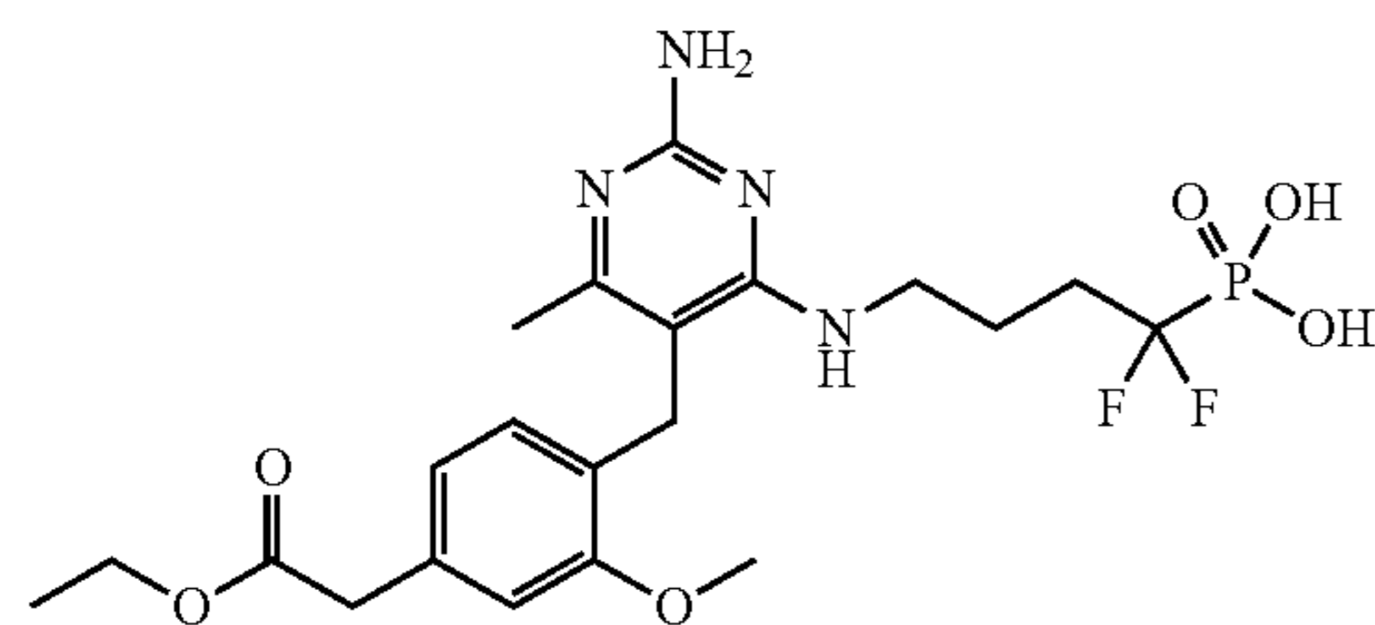
(4-((2-amino-5-(4-(2-ethoxy-2-oxoethyl)-2-methoxybenzyl)-6-methylpyrimidin-4-yl)amino)-1,1-difluorobutyl)phosphonic acid
