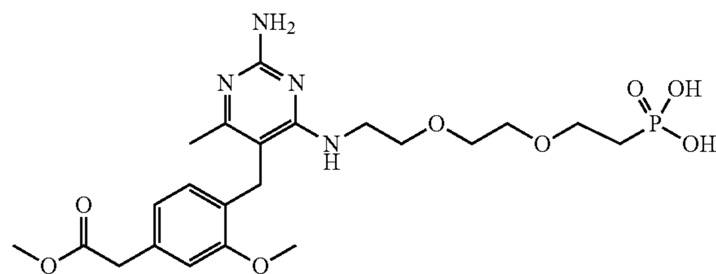
(2-(2-(2-((2-amino-5-(2-methoxy-4-(2-methoxy-2-oxoethyl)benzyl)-6-methylpyrimidin-4-yl)amino)ethoxy)ethoxy)ethyl)phosphonic acid
