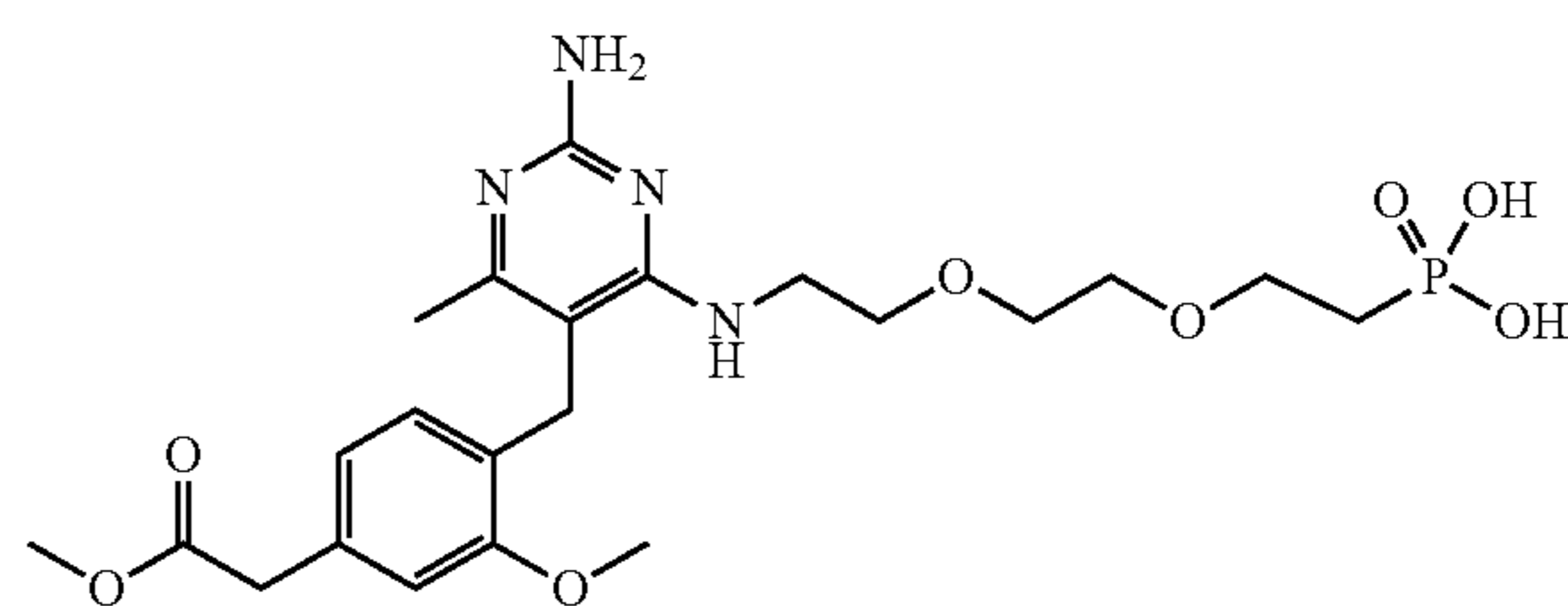
(2-(2-(2-((2-amino-5-(2-methoxy-4-(2-methoxy-2-oxoethyl)benzyl)-6-methylpyrimidin-4-yl)amino)ethoxy)ethoxy)ethyl)phosphonic acid
