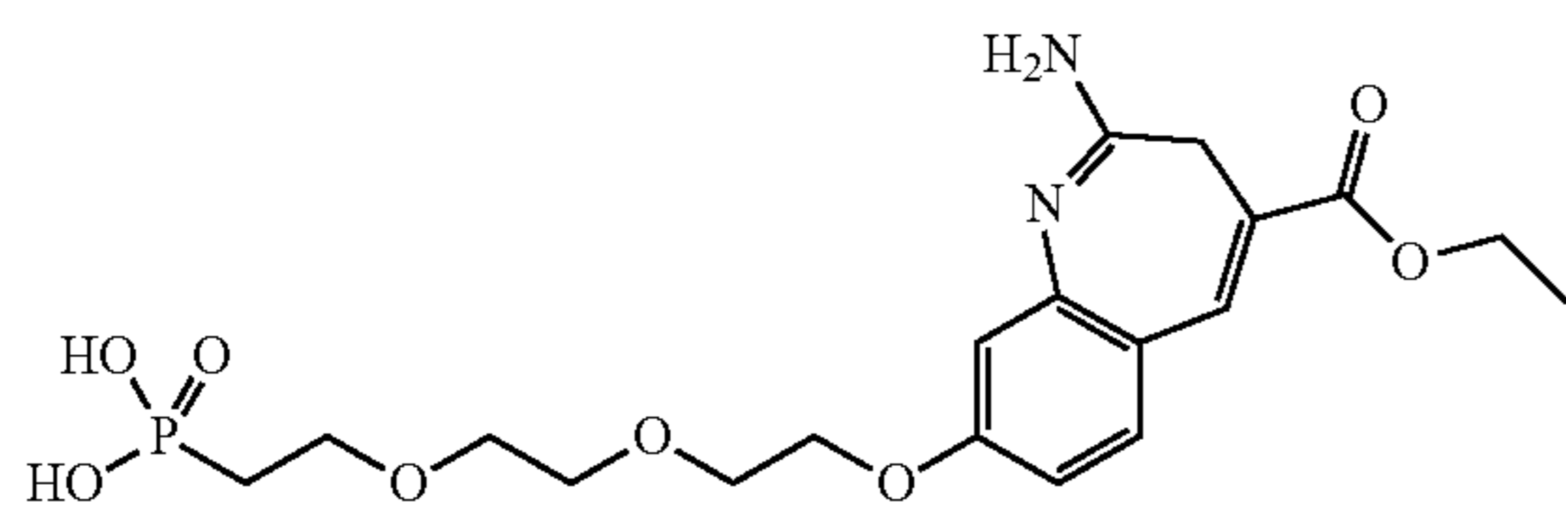
(2-(2-(2-((2-amino-4-(ethoxycarbonyl)-3H-benzo[b]azepin-8-yl)oxy)ethoxy)ethoxy)ethyl)phosphonic acid
