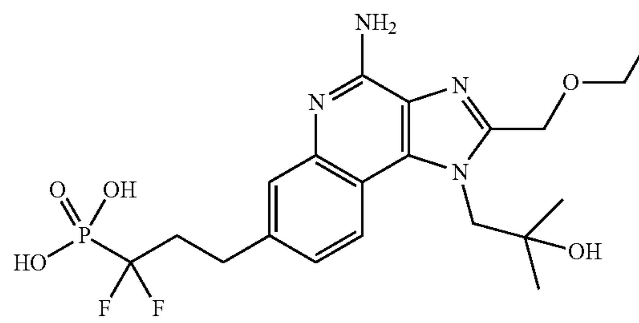
(3-(4-amino-2-(ethoxymethyl)-1-(2-hydroxy-2-methylpropyl)-1H-imidazo[4,5-c]quinolin-7-yl)-1,1-difluoropropyl)phosphonic acid
