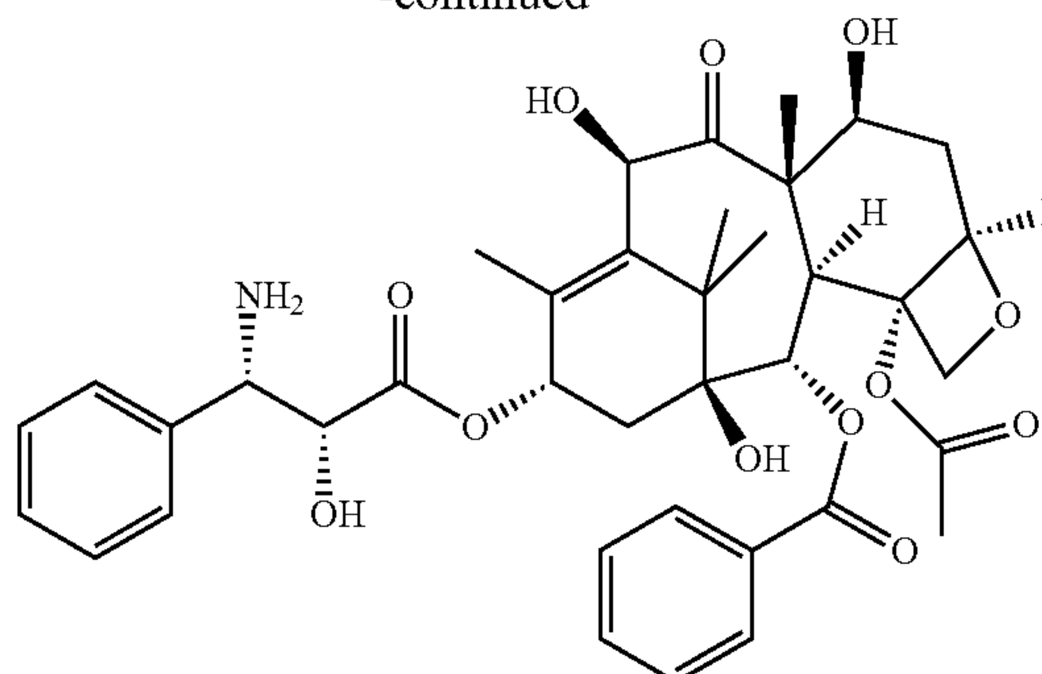
3'-Aminodocetaxel
