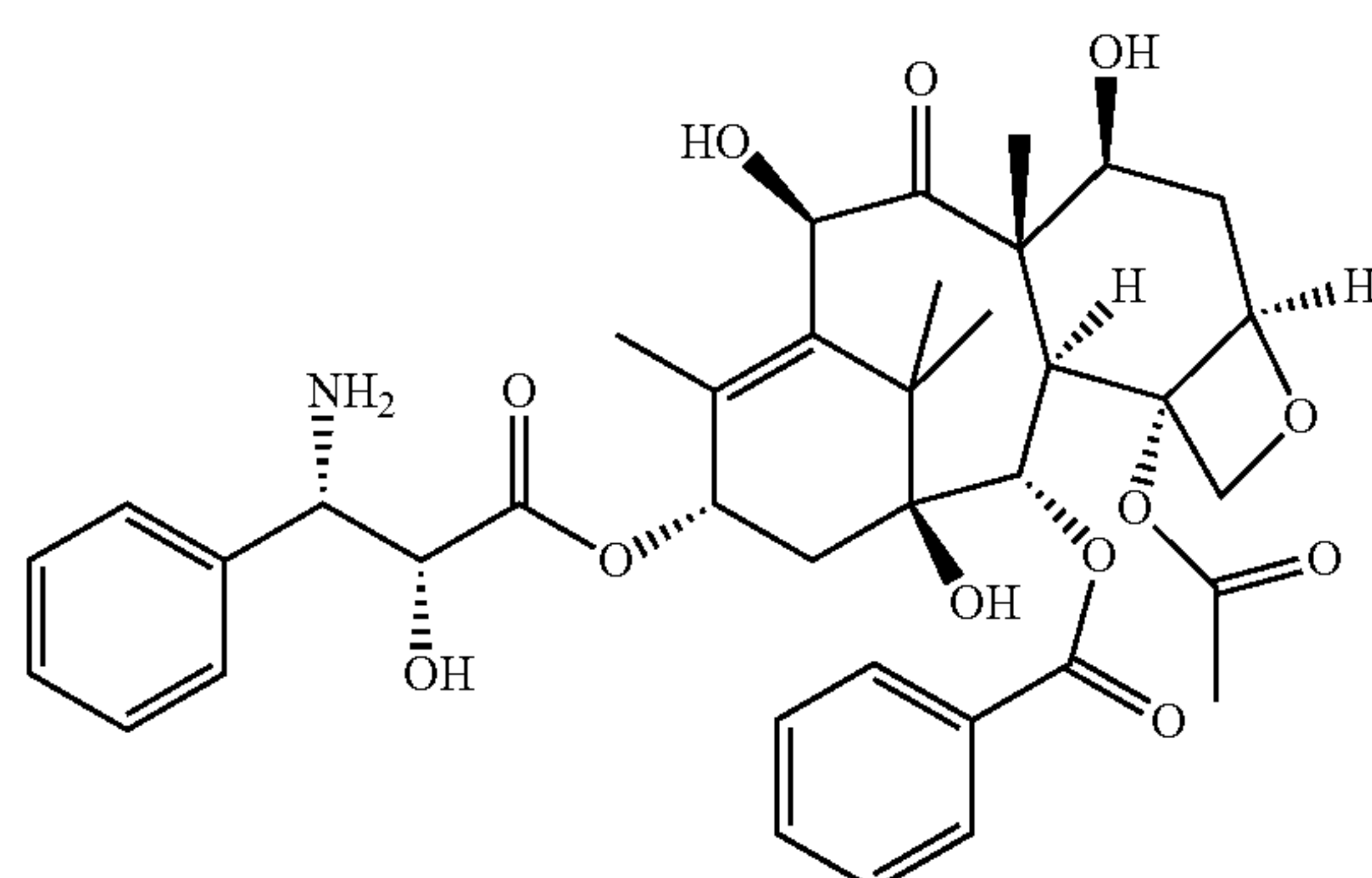
3'-Aminodocetaxel
