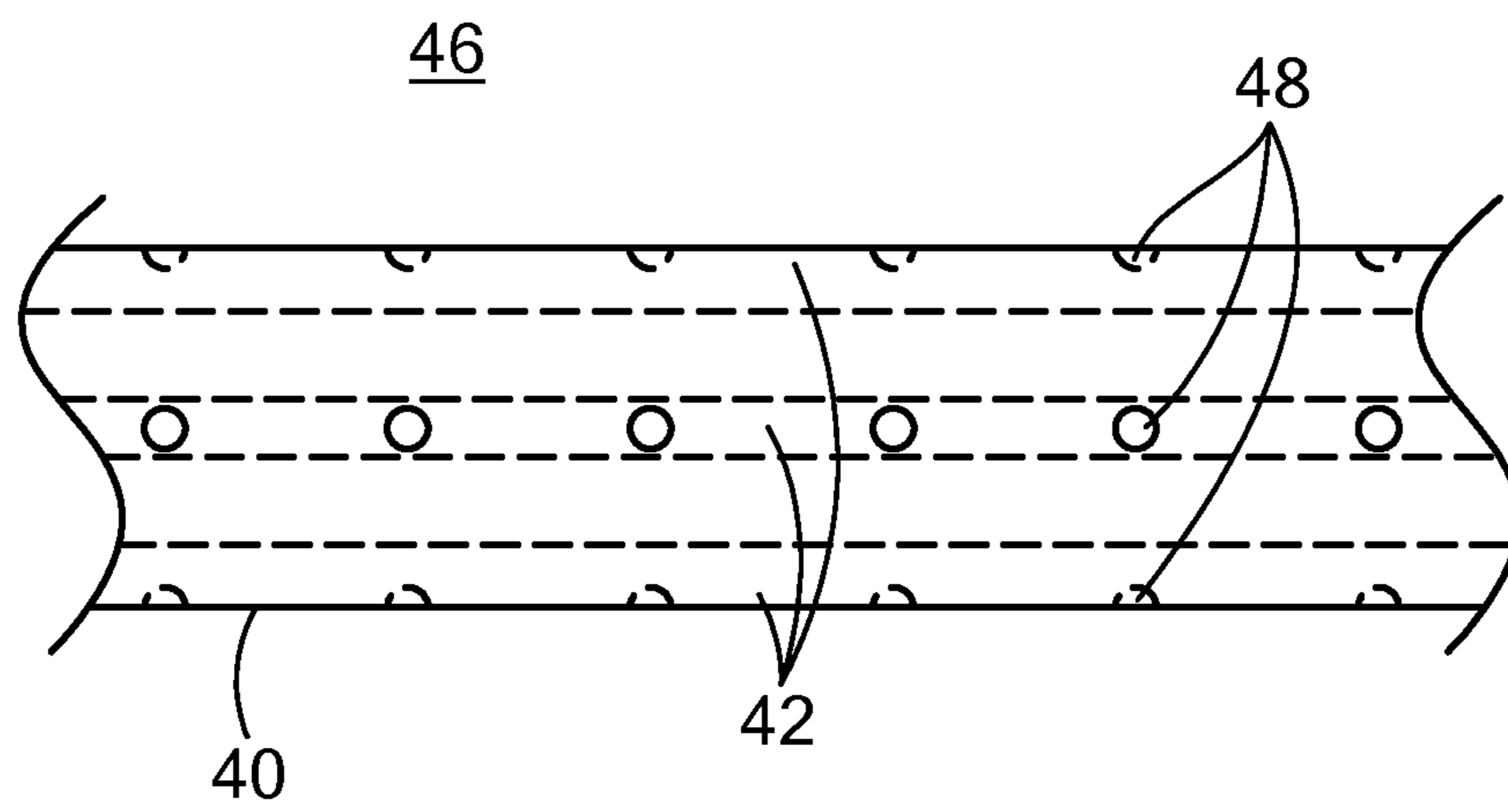
FIG. 4A
