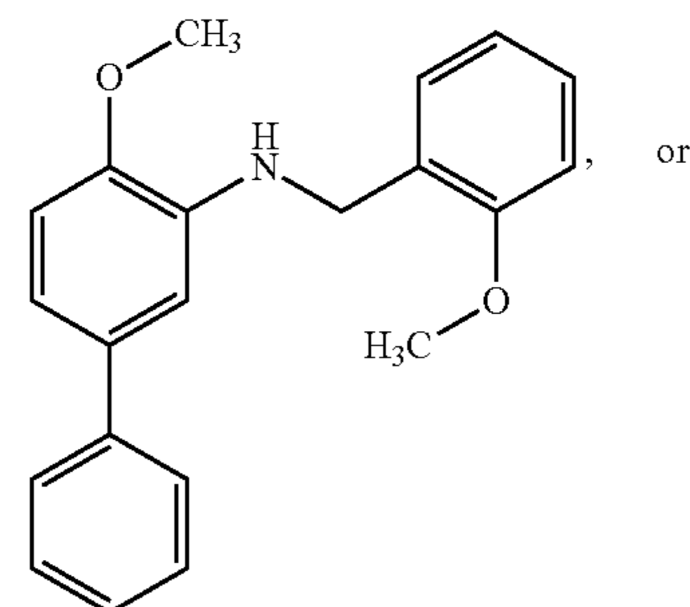
(2-methoxybenzyl)(4-methoxy-3-biphenyl)amine
