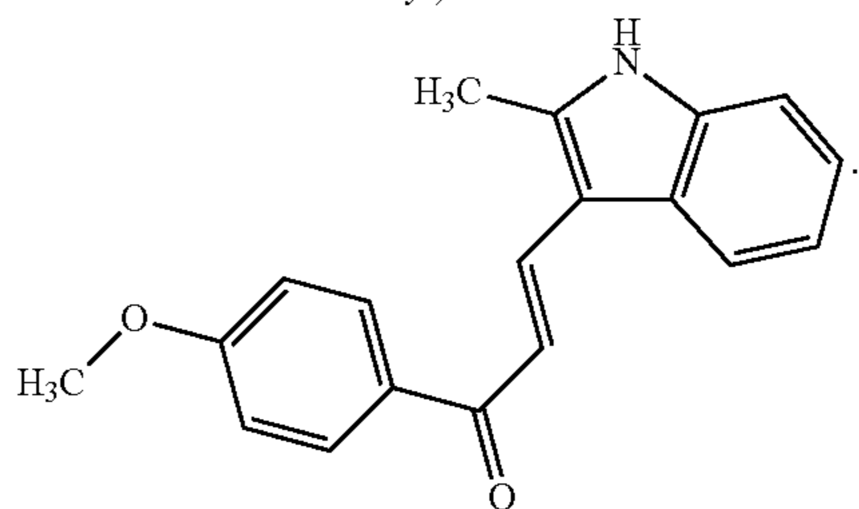
1-(4-methoxyphenyl)-3-(2-methyl-1H-indol-3-yl)-2-propen-1-one
