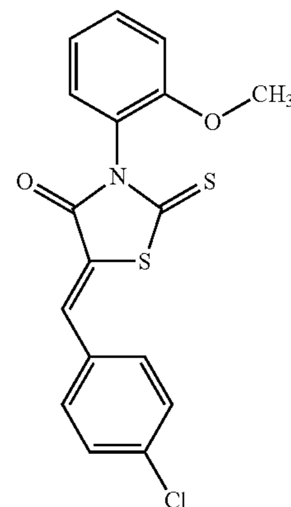
5-(4-chlorobenzylidene)-3-(2-methoxyphenyl)-2-thioxo-1,3-thiazolidin-4-one
