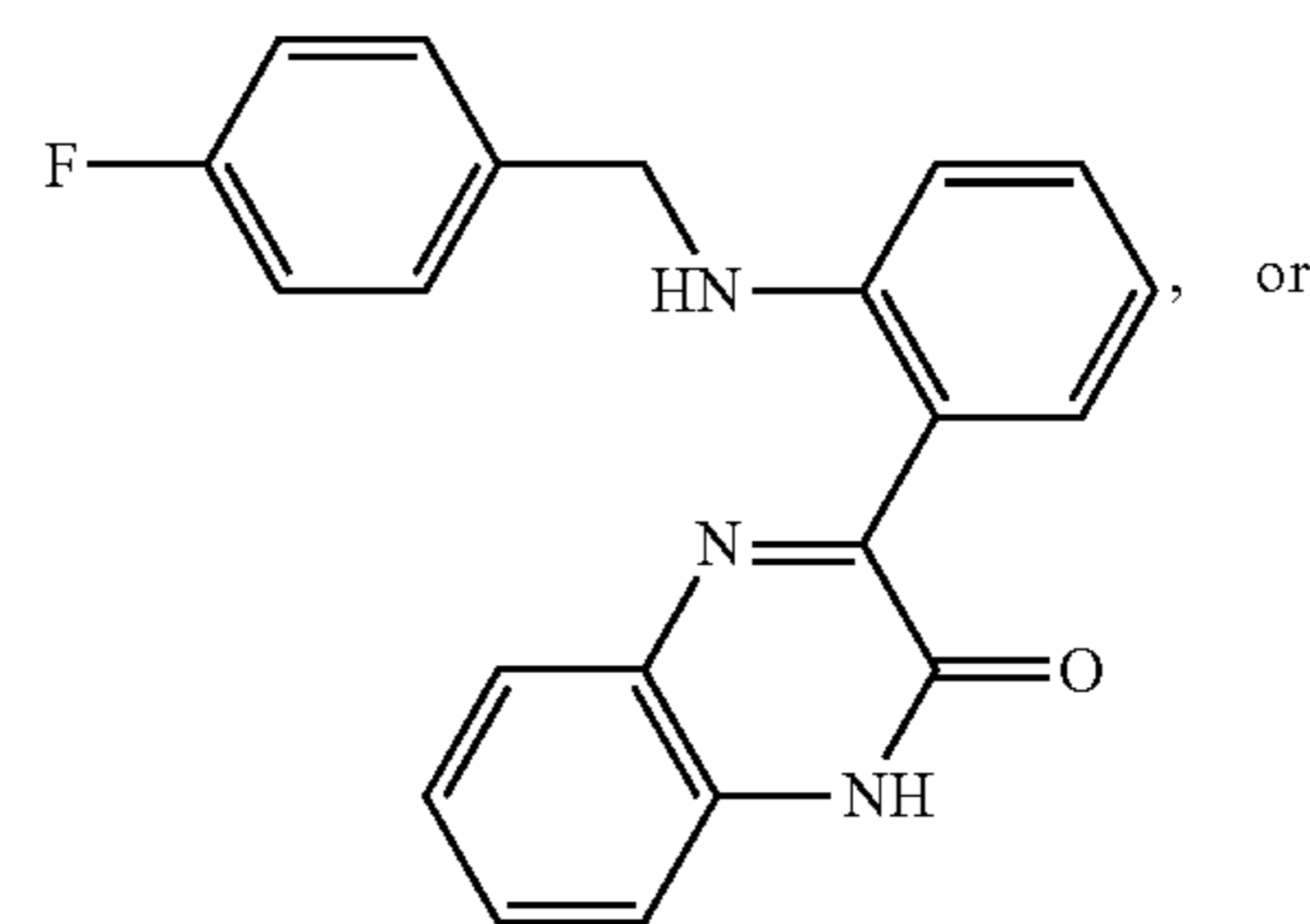
3-{2-[(fluorobenzyl)amino]phenyl}-2(1H)-quinoxalinone
