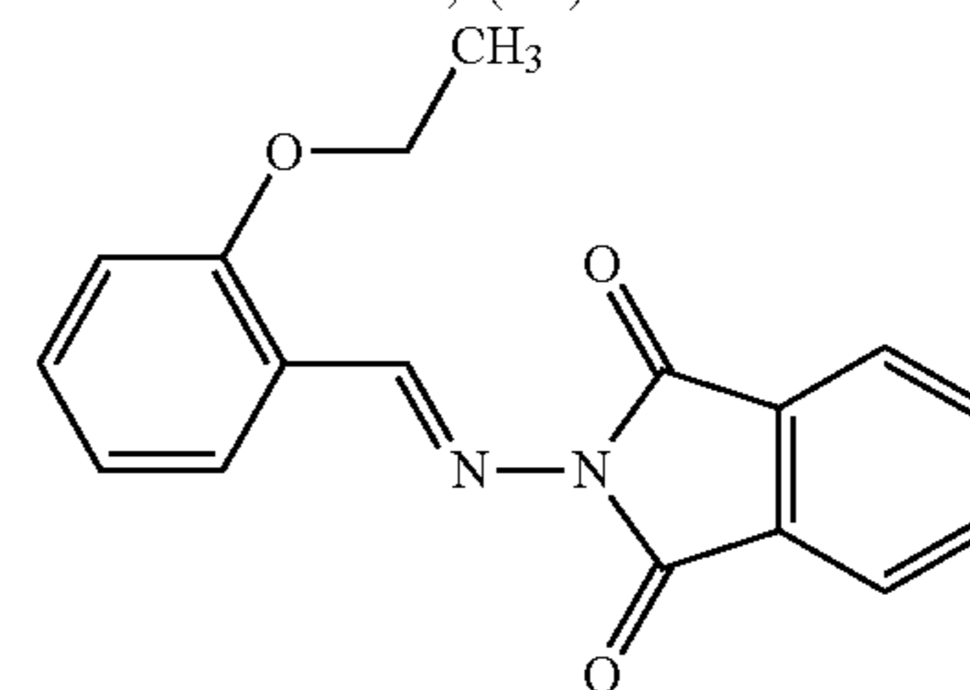
2-[(2-ethoxybenzylidene)amino]-1H-isoindole-1,3(2H)-dione
